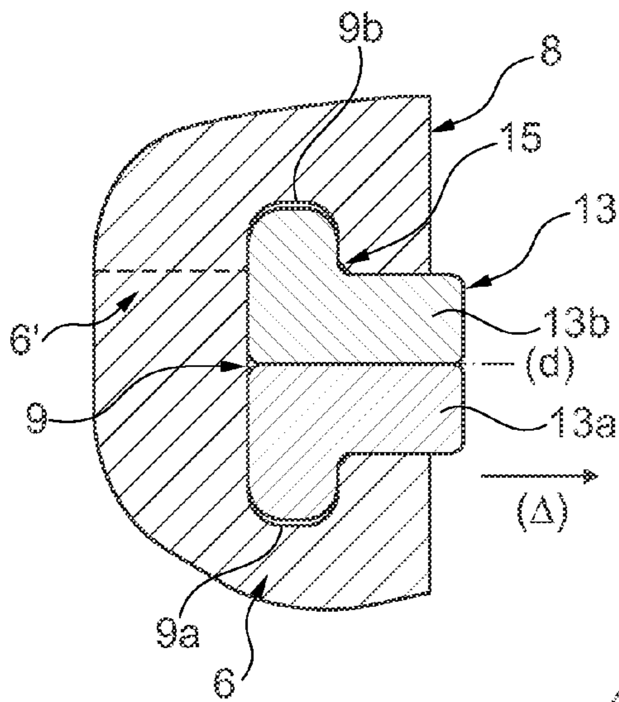
Fig. 7a Section A-A
