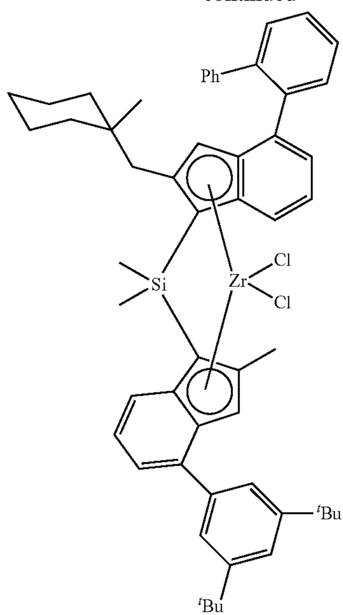
MTC-2 rac/meso = 23/1
