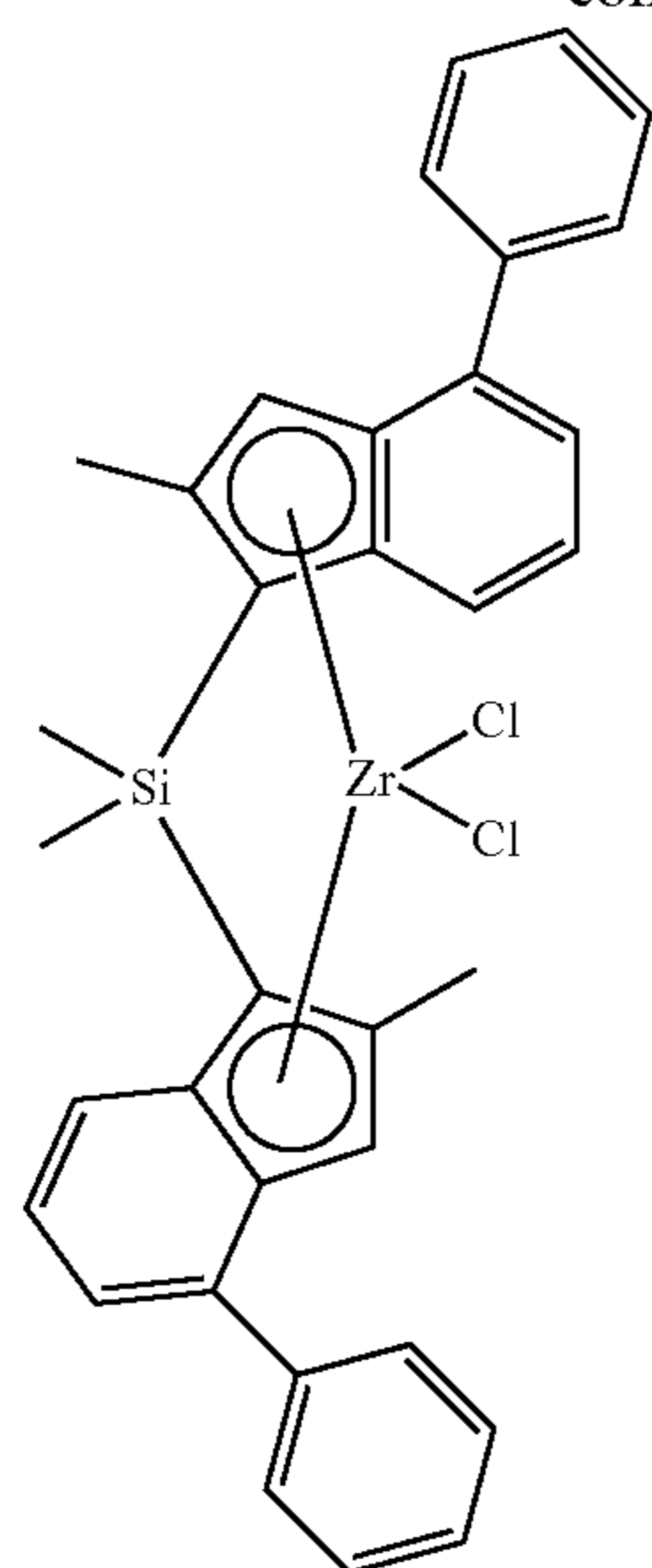
MTC-A rac/meso > 20:1
