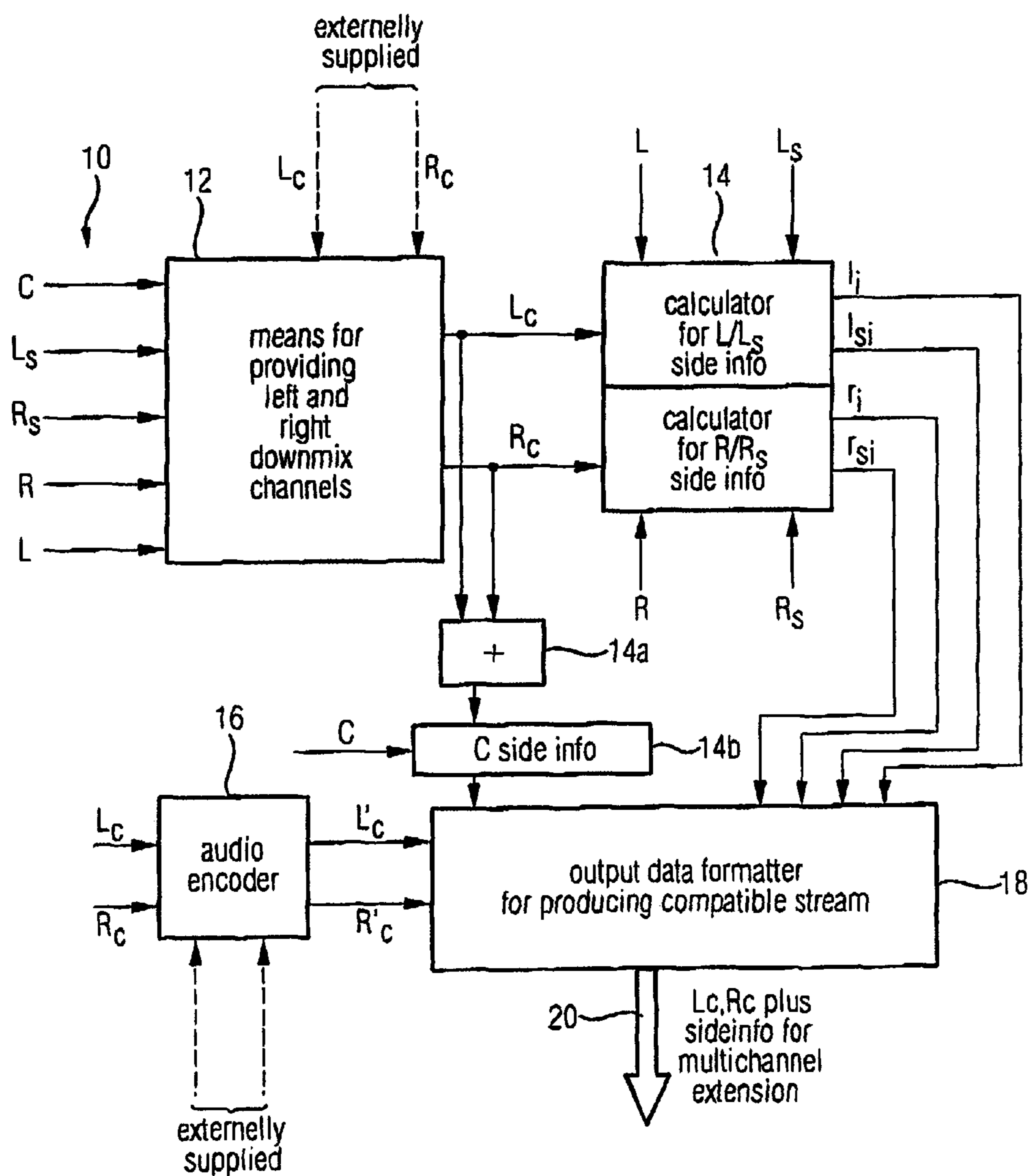
FIG 1 (Encoder)
