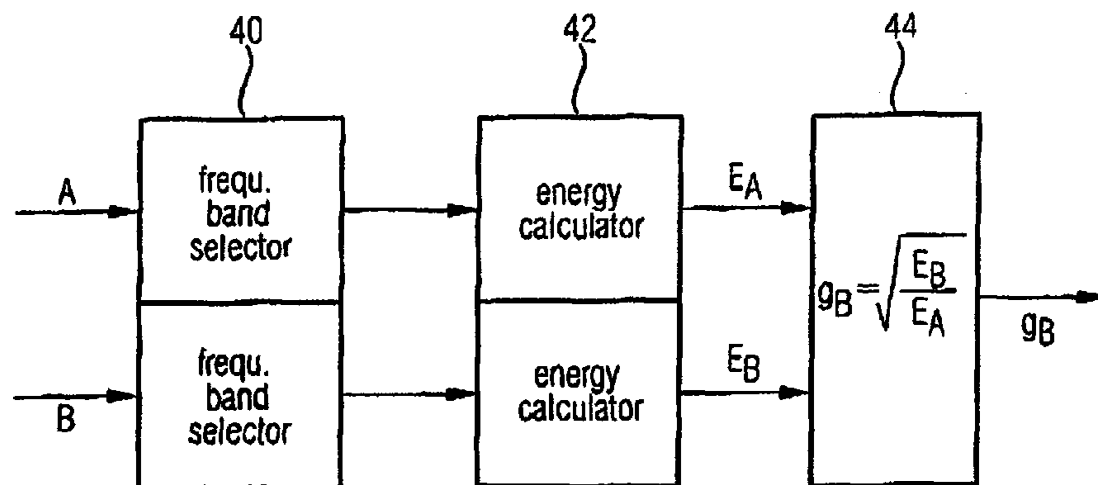
FIG 4 (encoder side)
