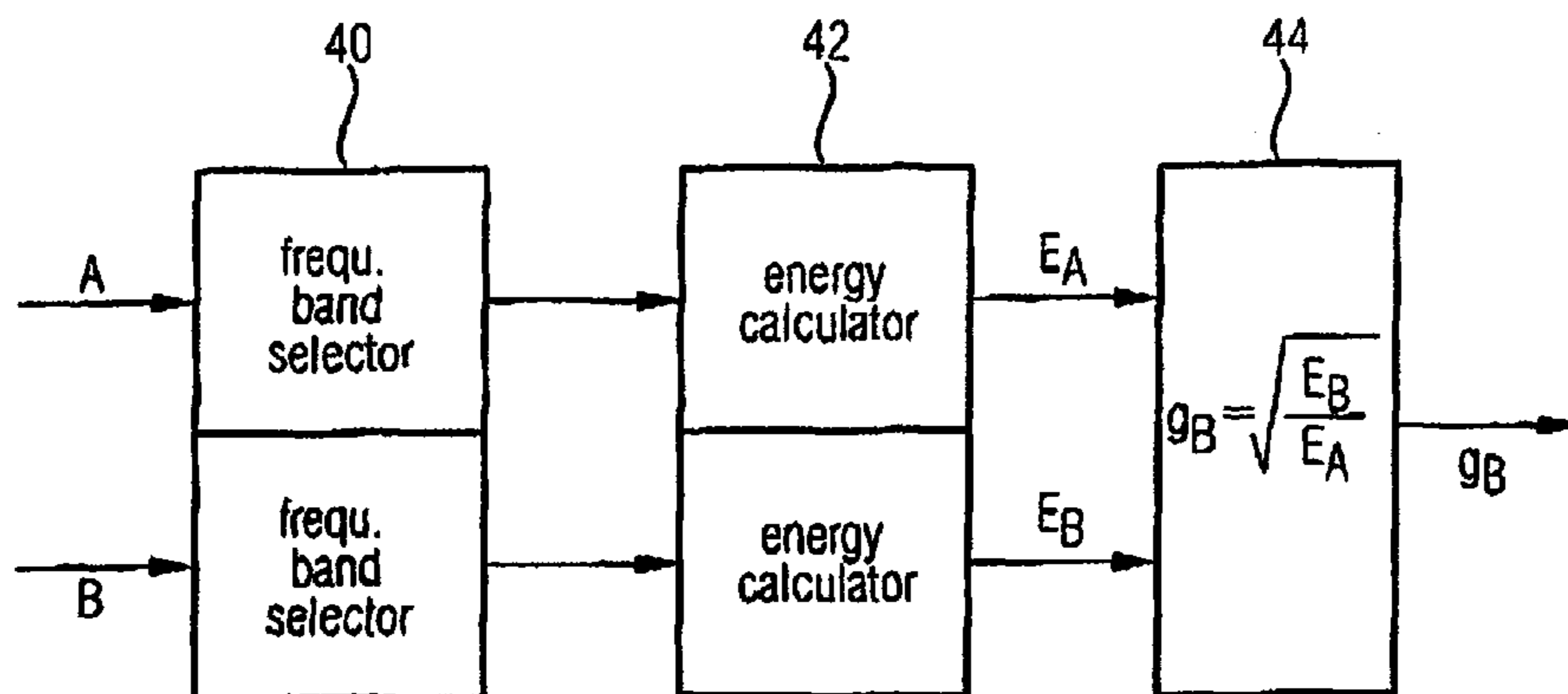
FIG 4 (encoder side)
