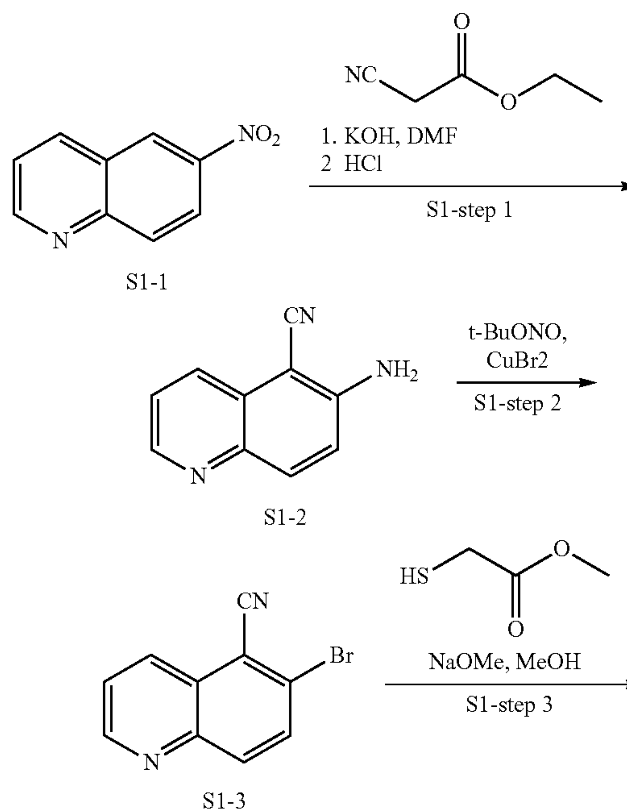
Scheme 1A
