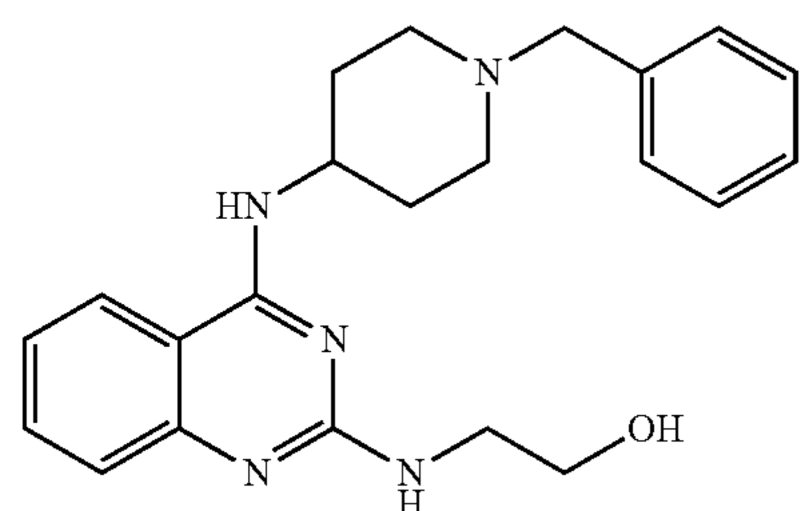
2-((4-((1-benzylpiperidin-4-yl)amino)quinazolin-2-yl)amino)ethanol
