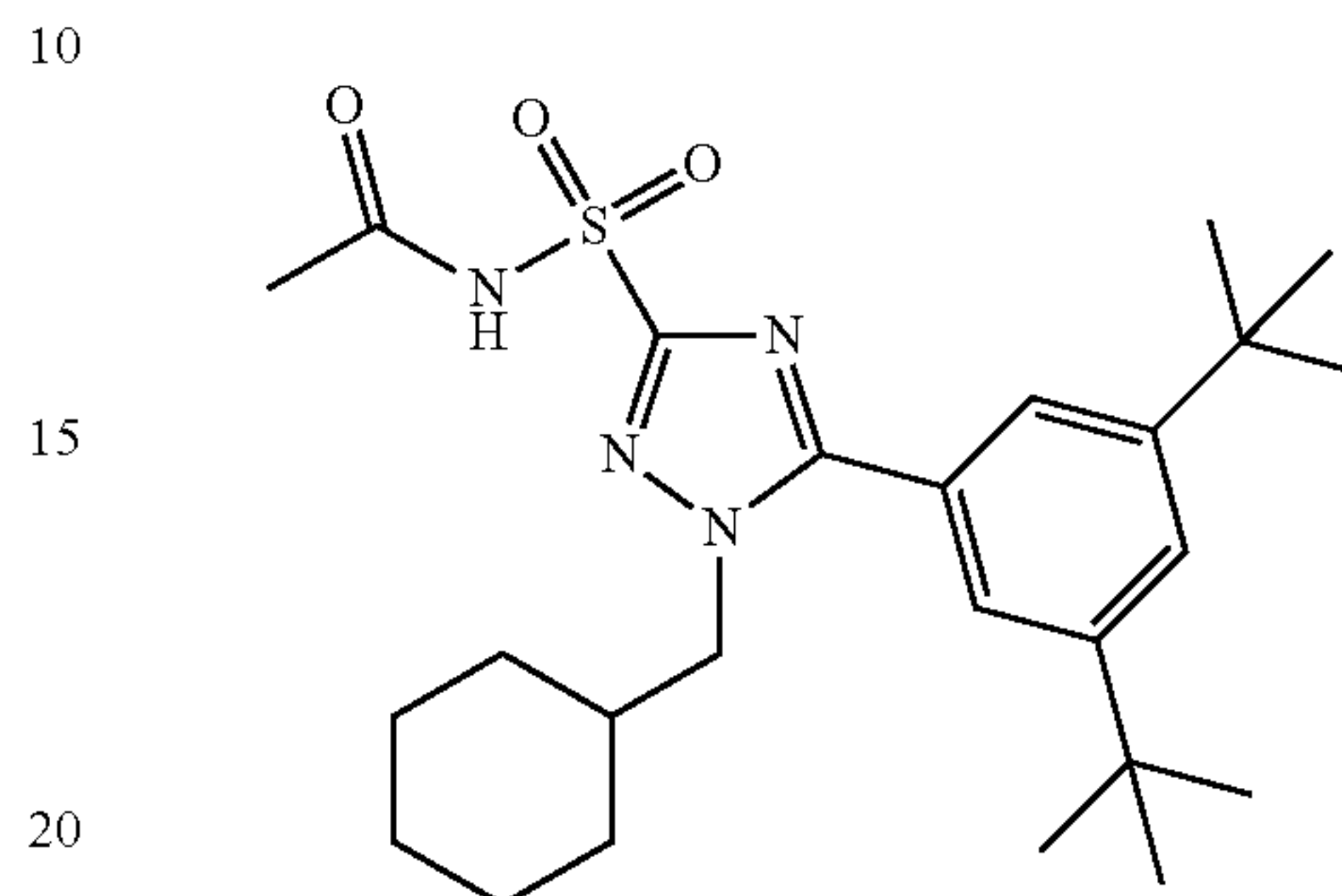
N-((1-(Cyclohexylmethyl)-5-(3,5-di-tert-butylphenyl)-1H-1,2,4-triazol-3-yl)sulfonyl)acetamide
