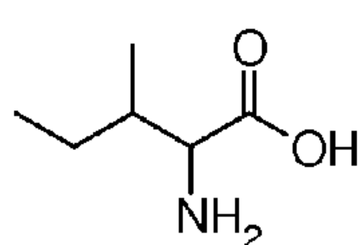
Allo-isoleucine
