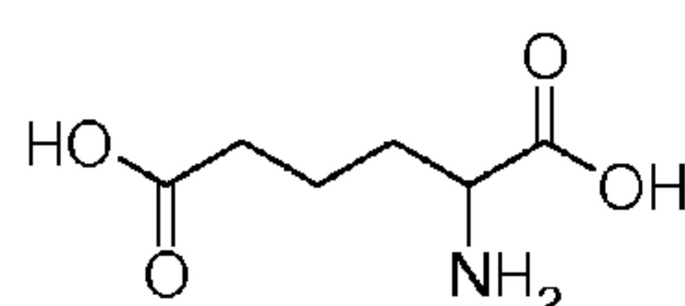
2-Aminoadipic acid
