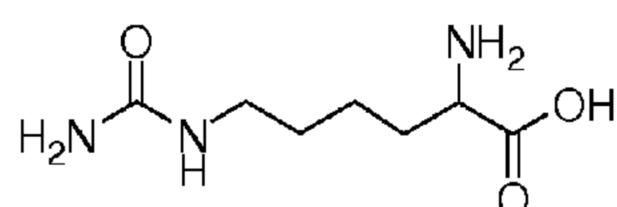
Homocitrulline
