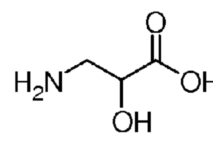
Isoserine
