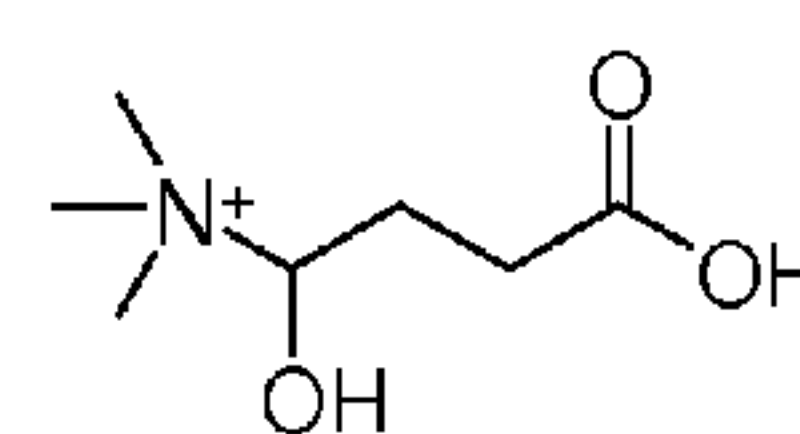
Carnitine
