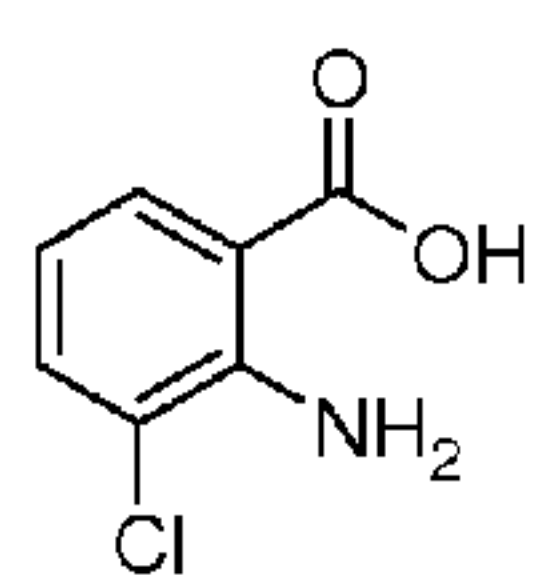
2-Amino-3-chlorobenzoic acid
