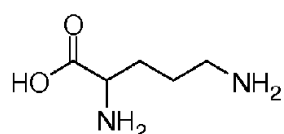
Ornithine
