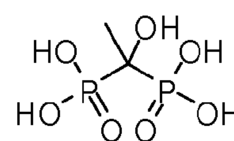
Etidronate
