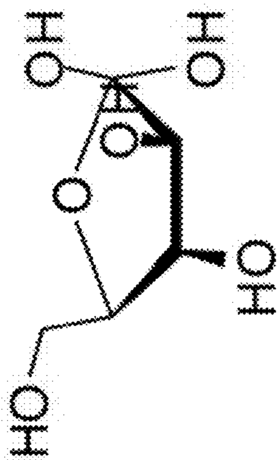
D-Fructofuranose
