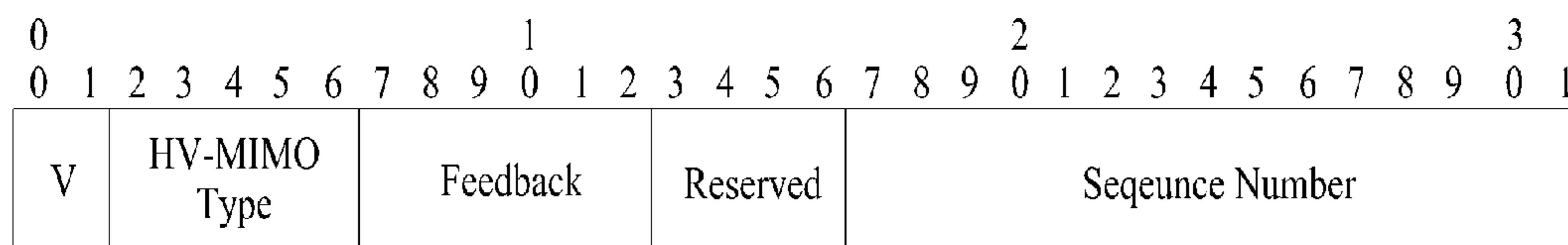
HV-MIMO Header
