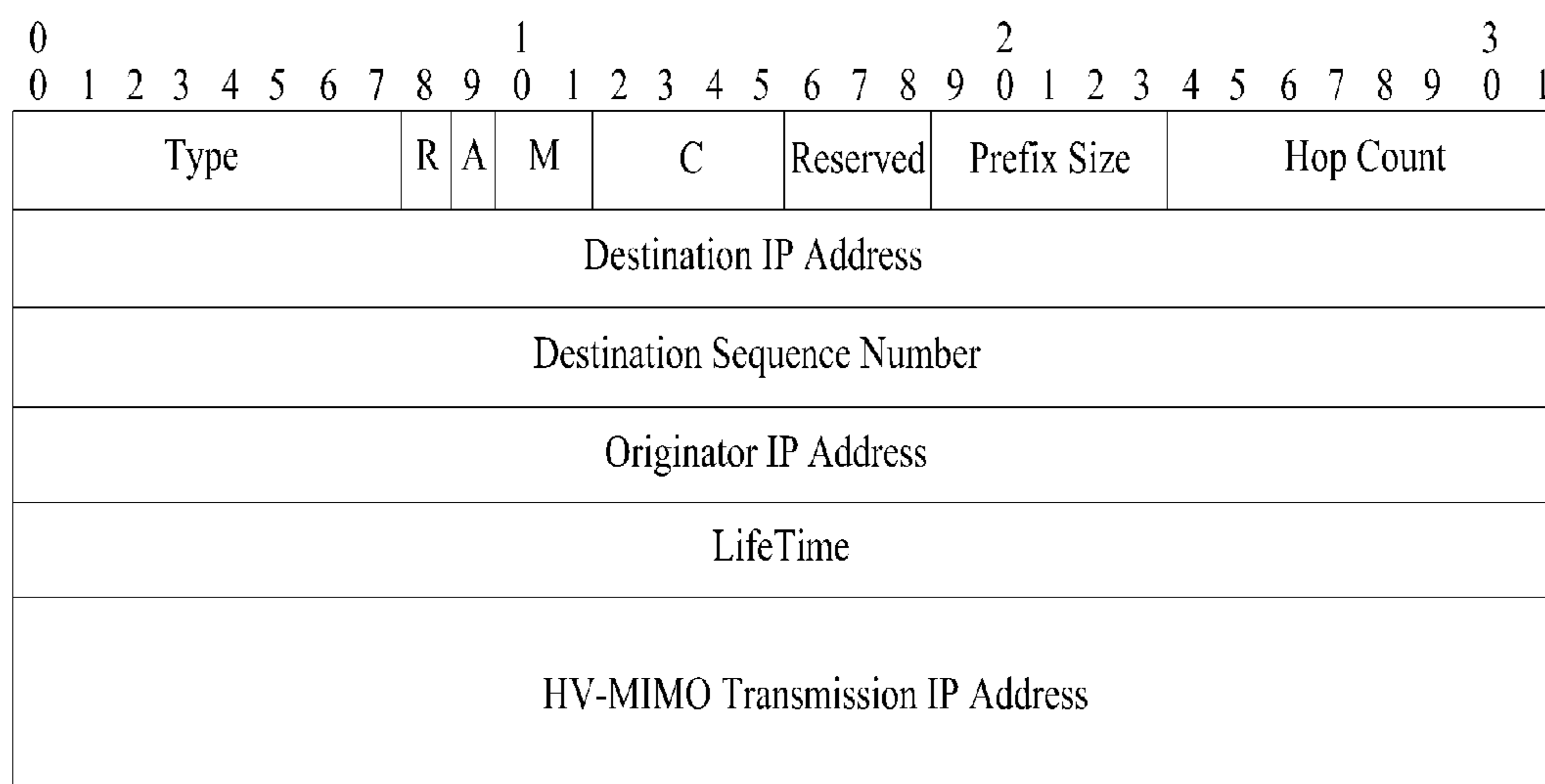
HV-MIMO Setup Message Format
