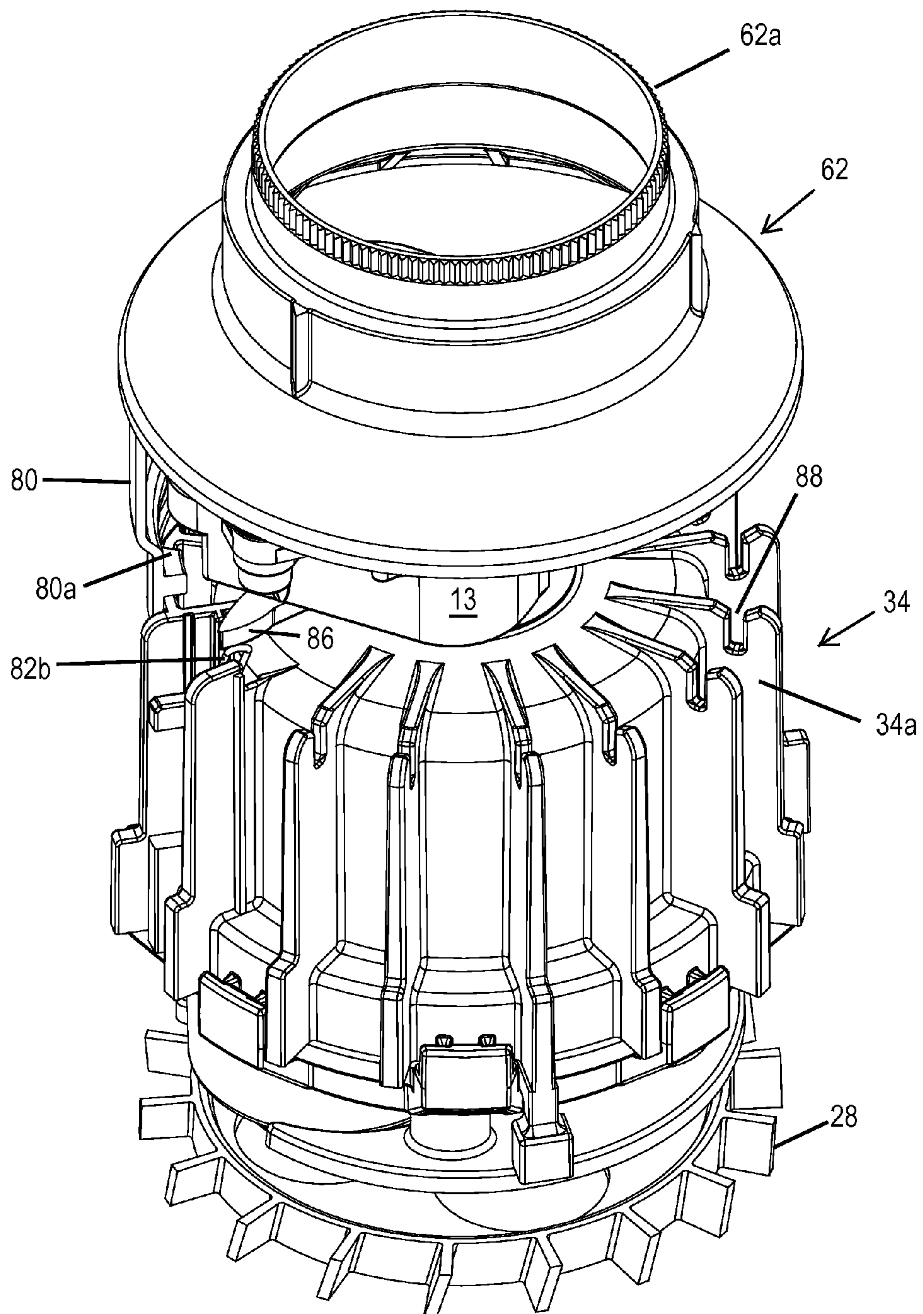
FIG. 15
