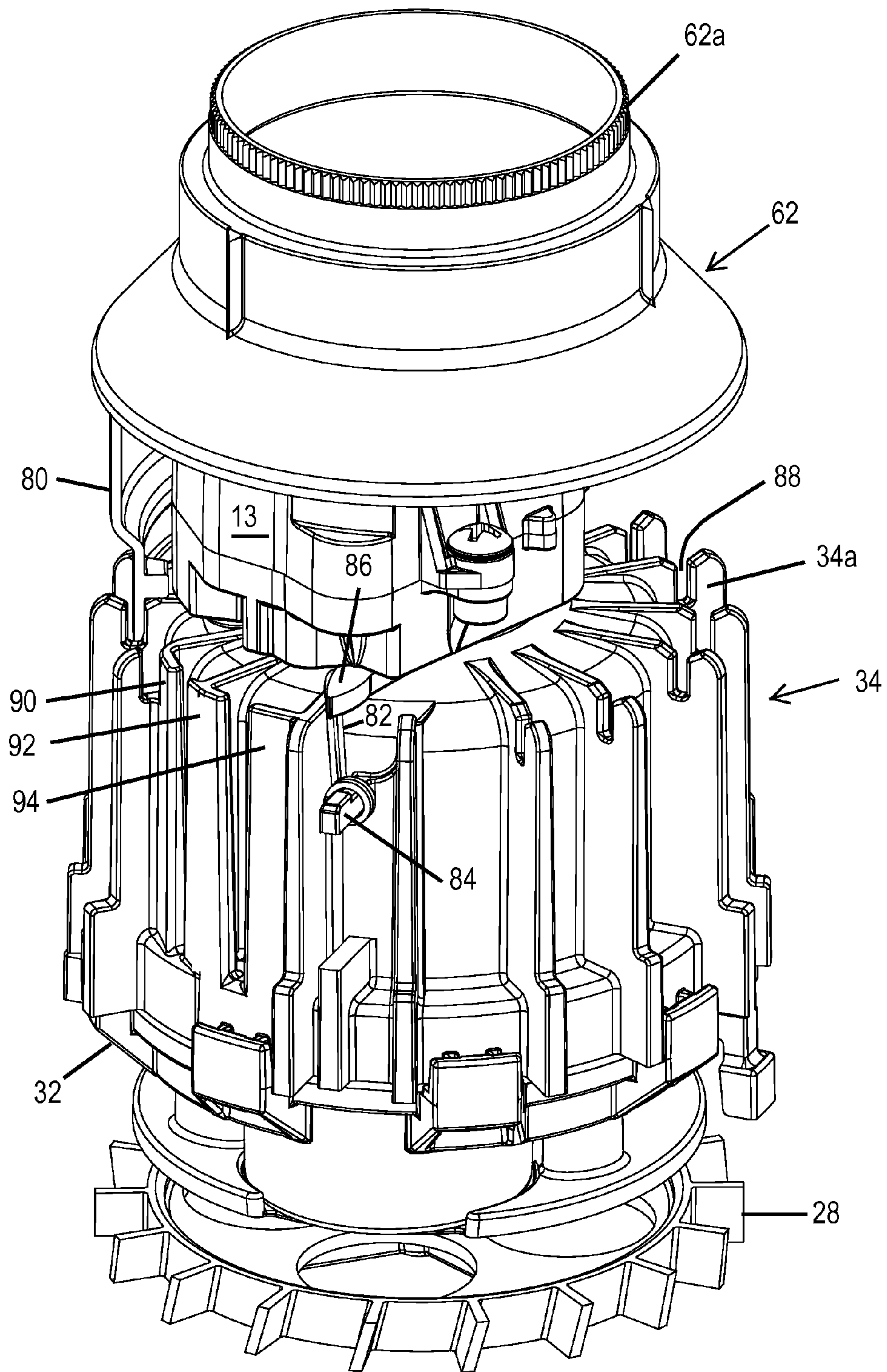
FIG. 10B
