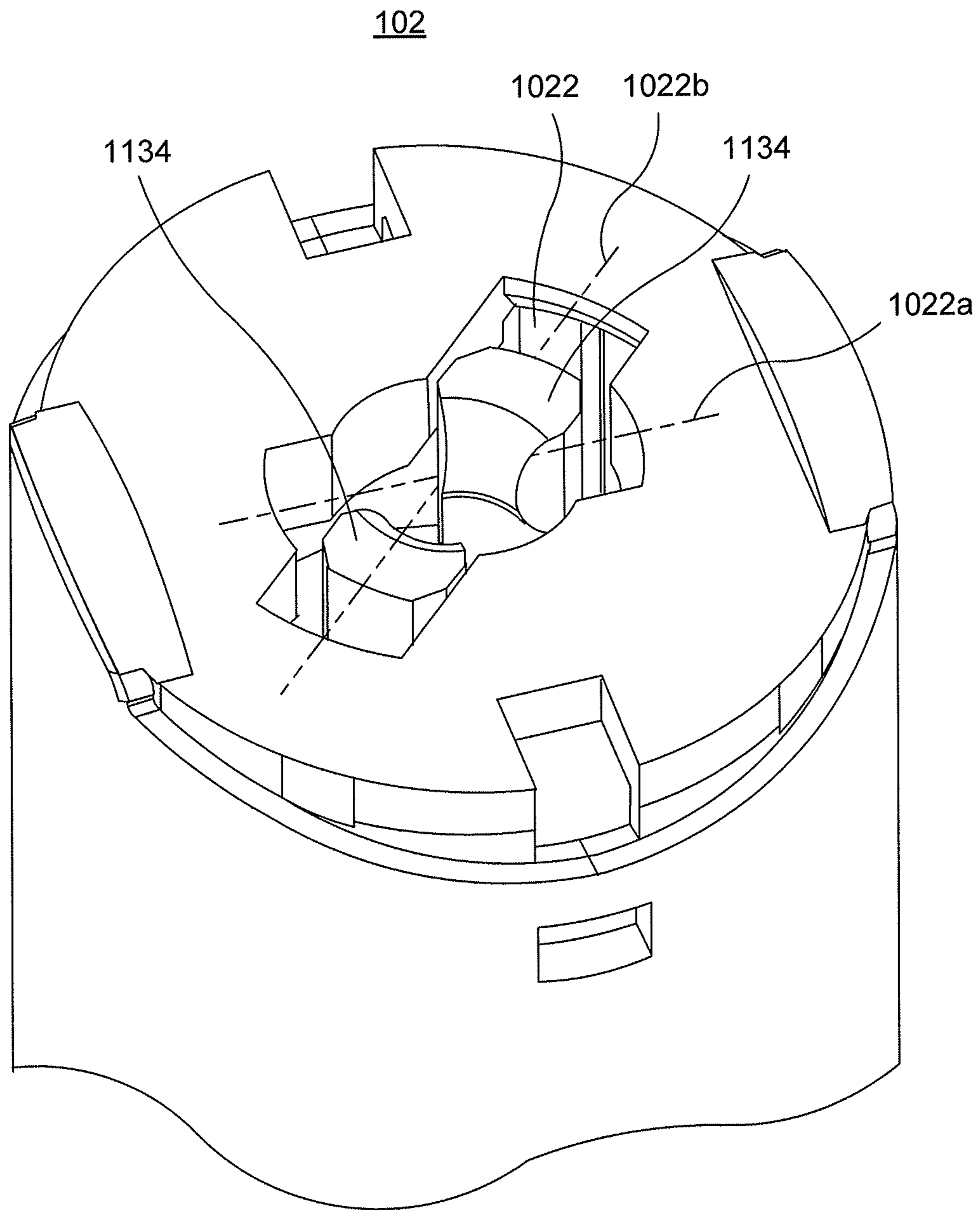
FIG. 2B
