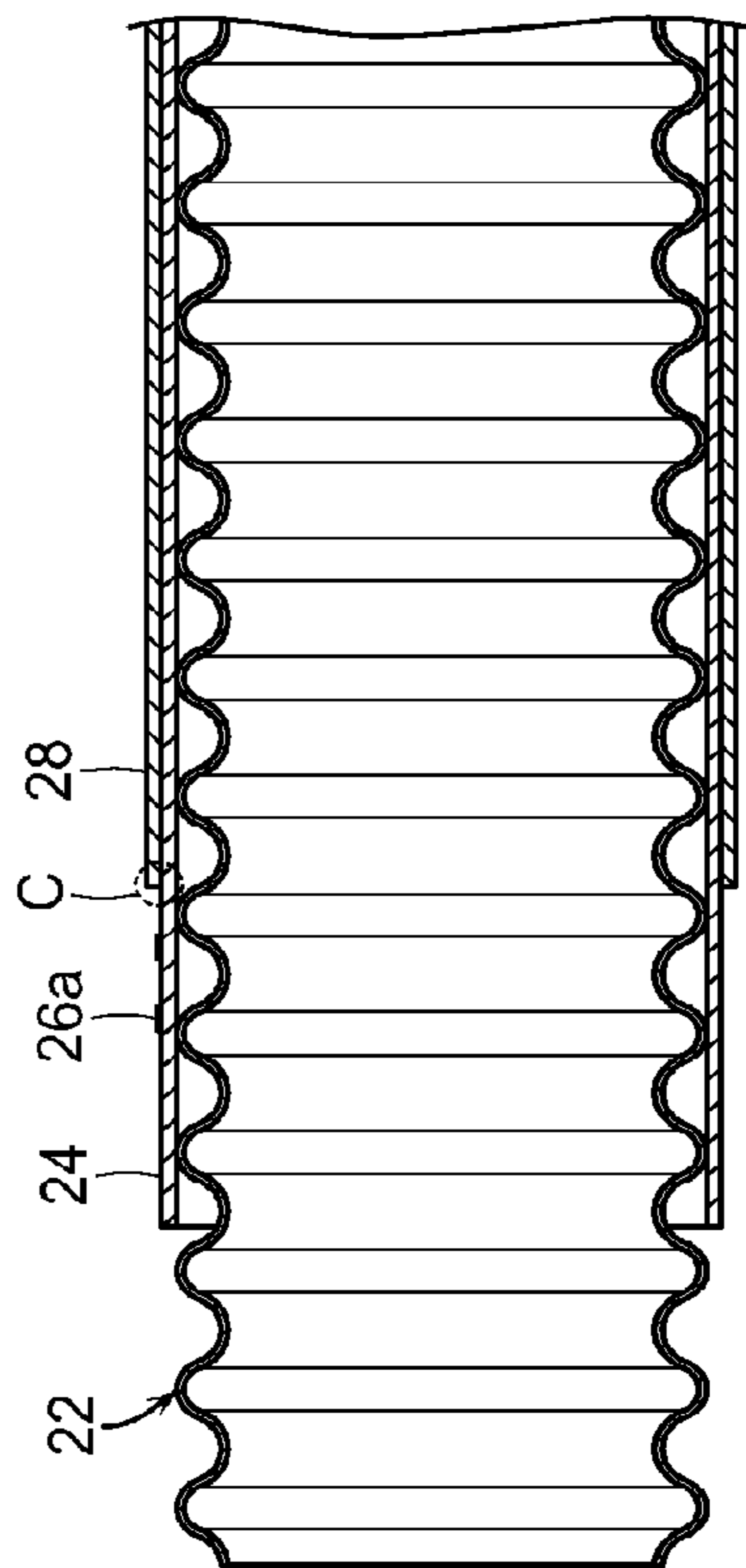
Section A-A
