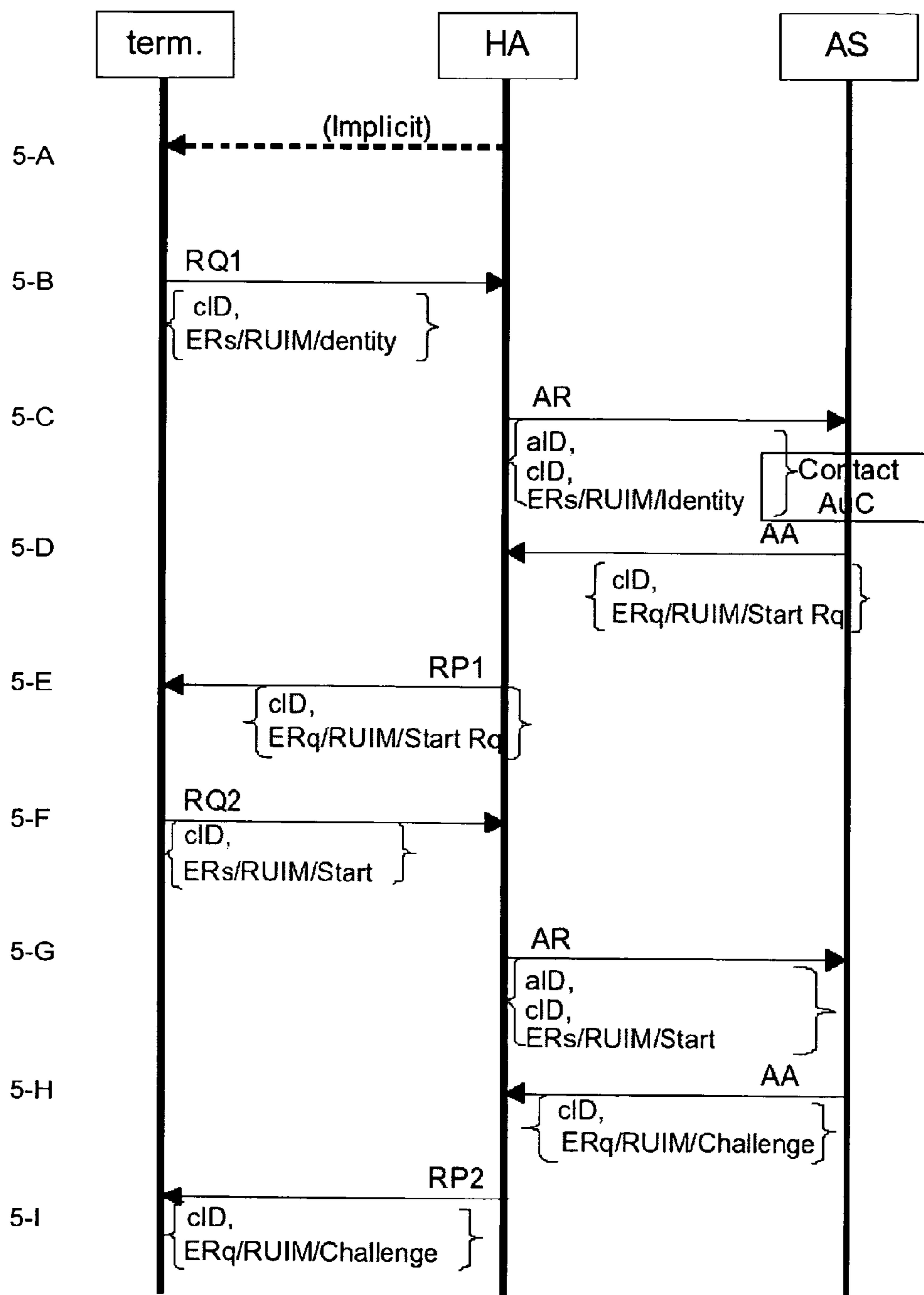
Fig. 5A
