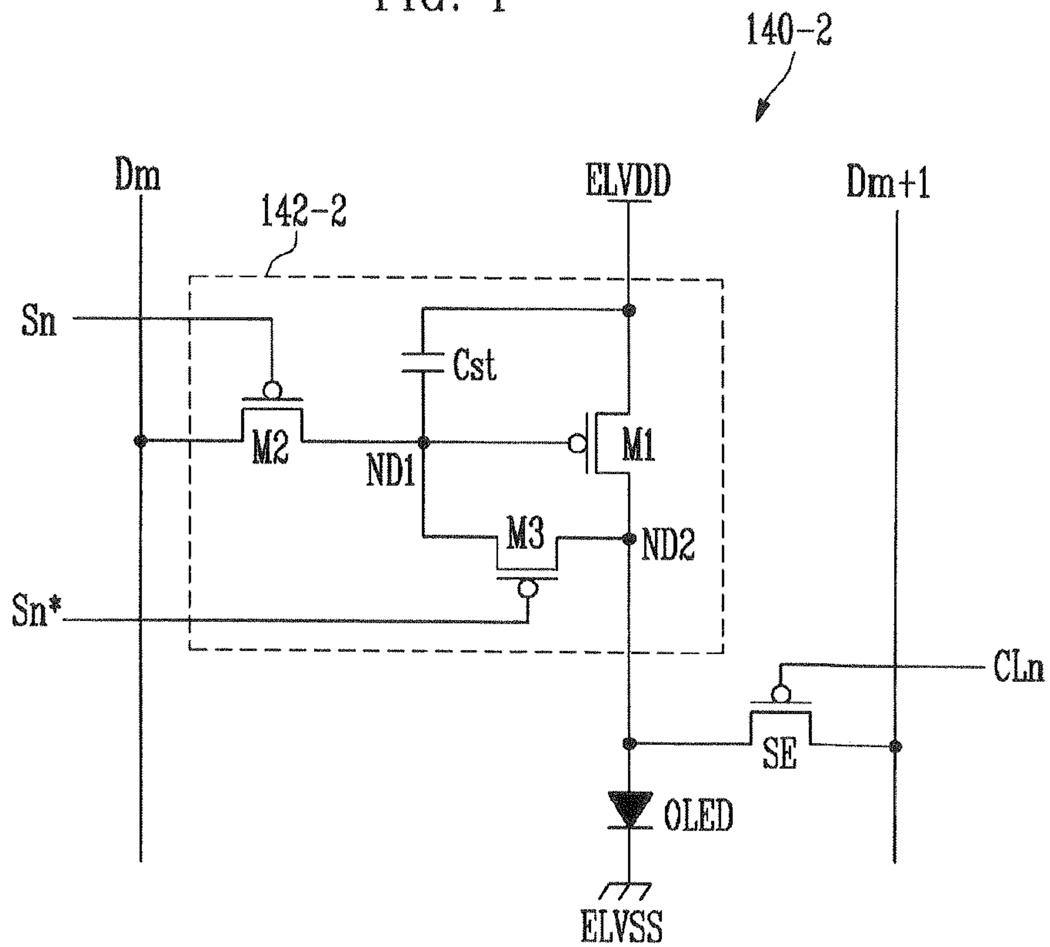
FIG. 4
