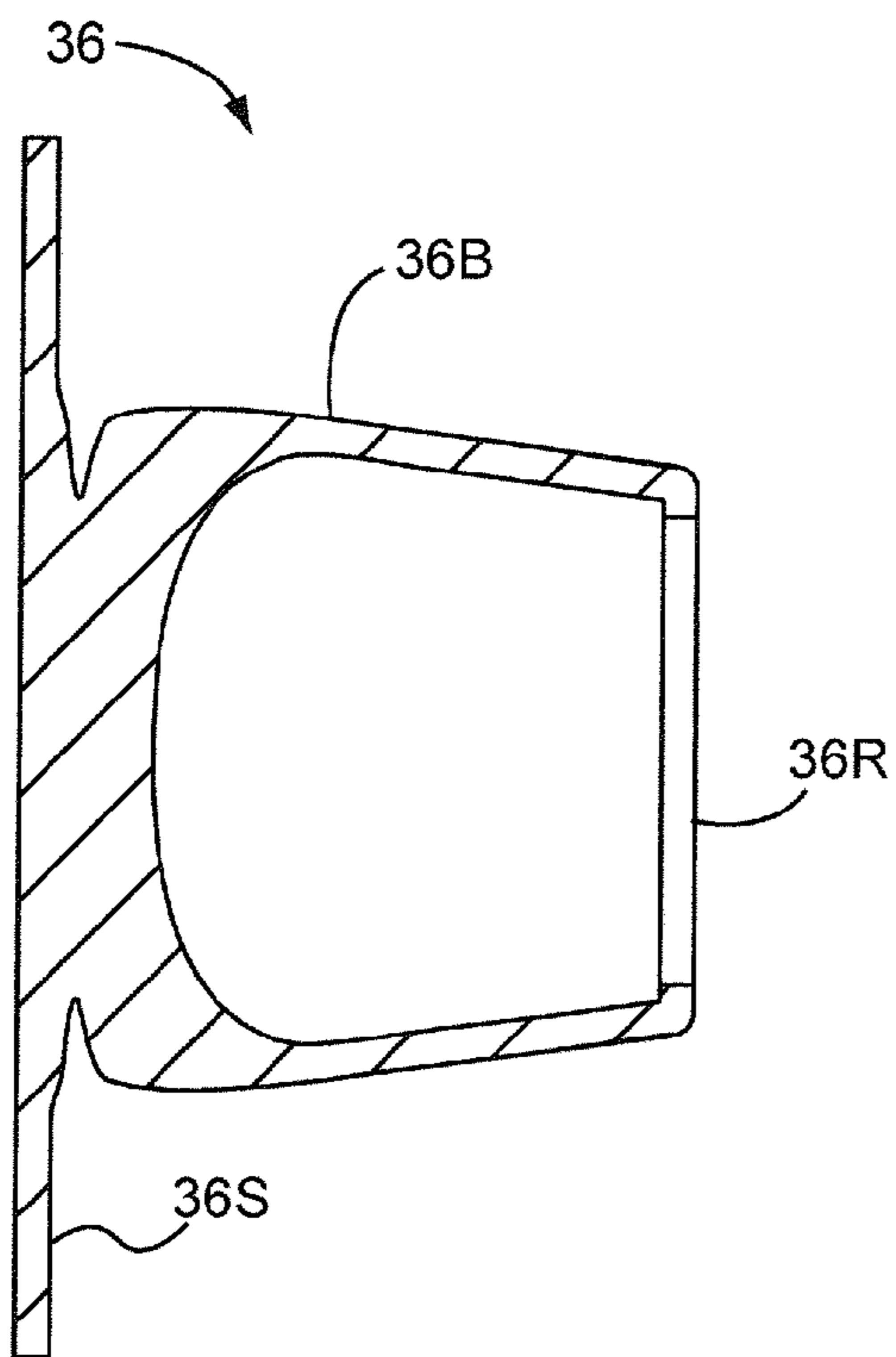
FIG. 12I SECTION E-E
