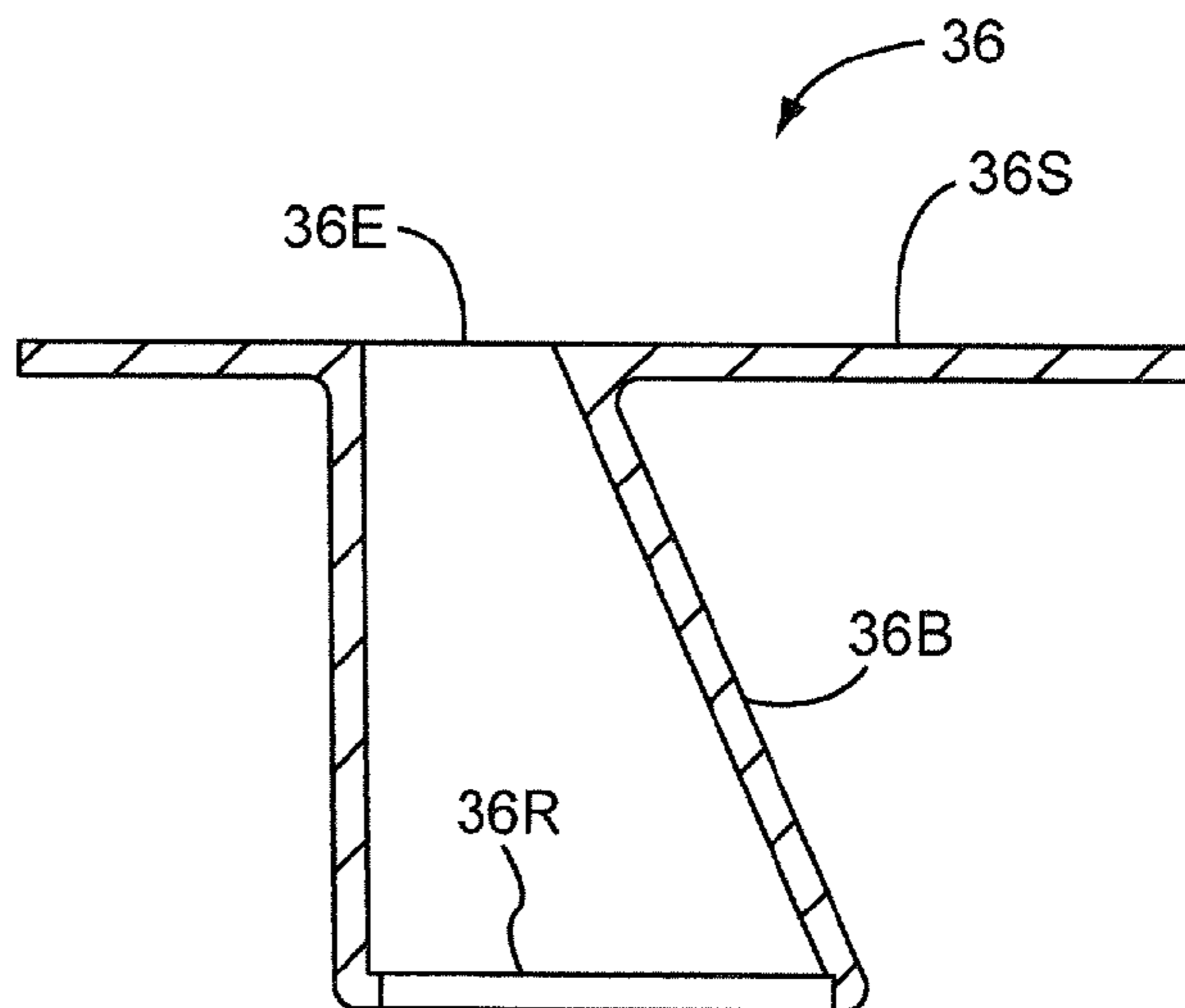
FIG. 12H SECTION D-D
