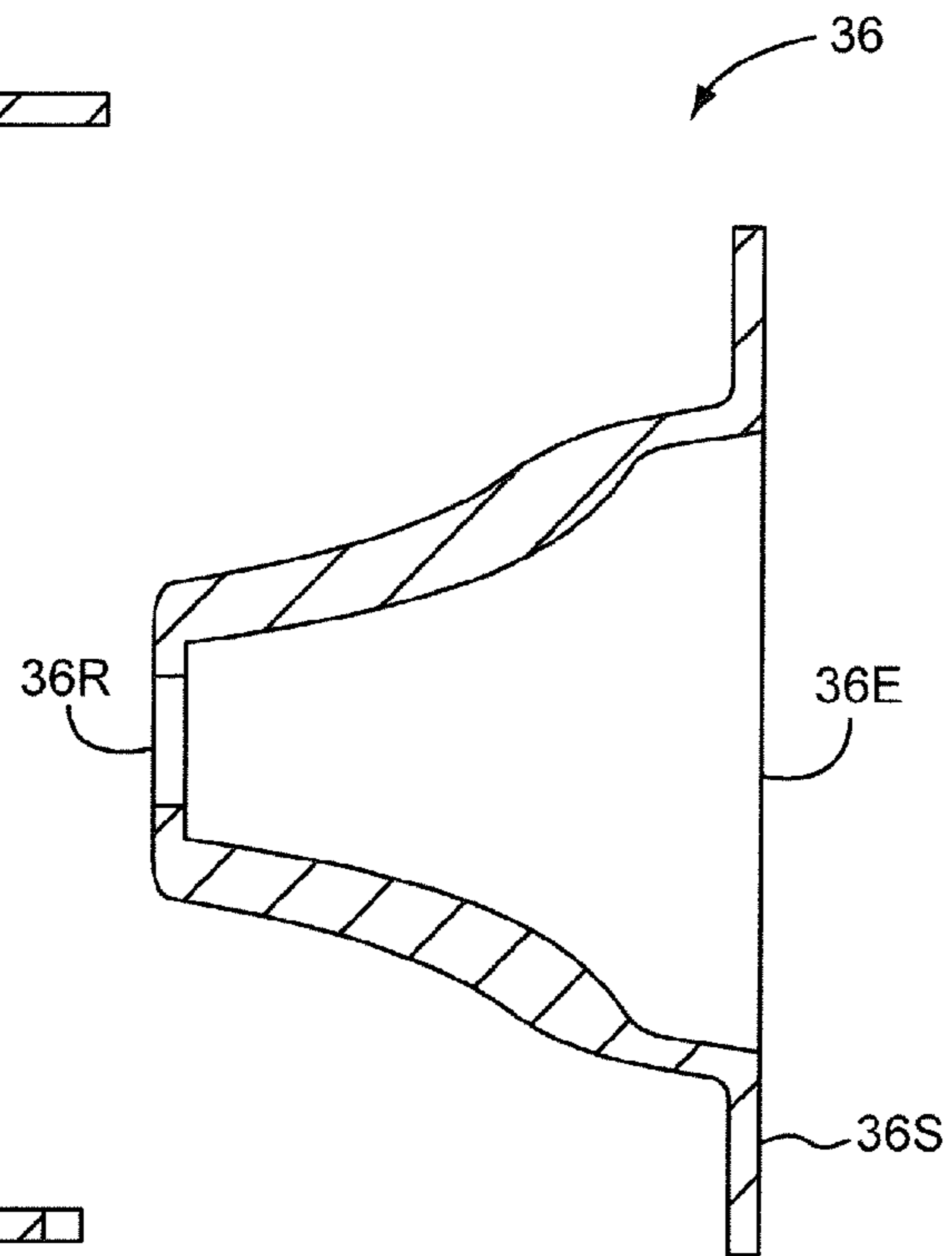
FIG. 12K SECTION G-G
