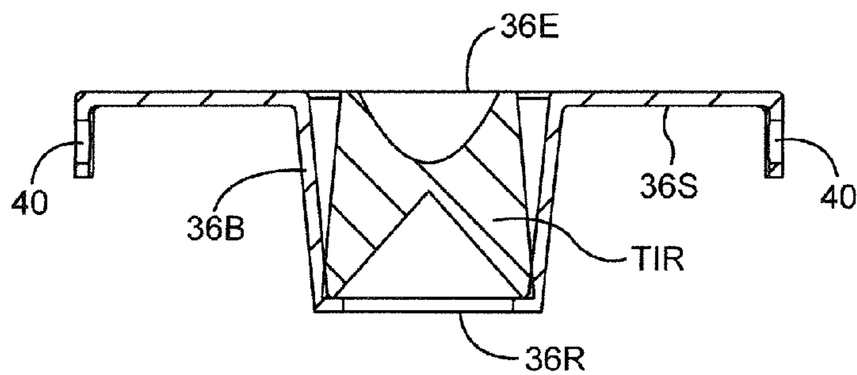
FIG. 21F SECTION A-A
