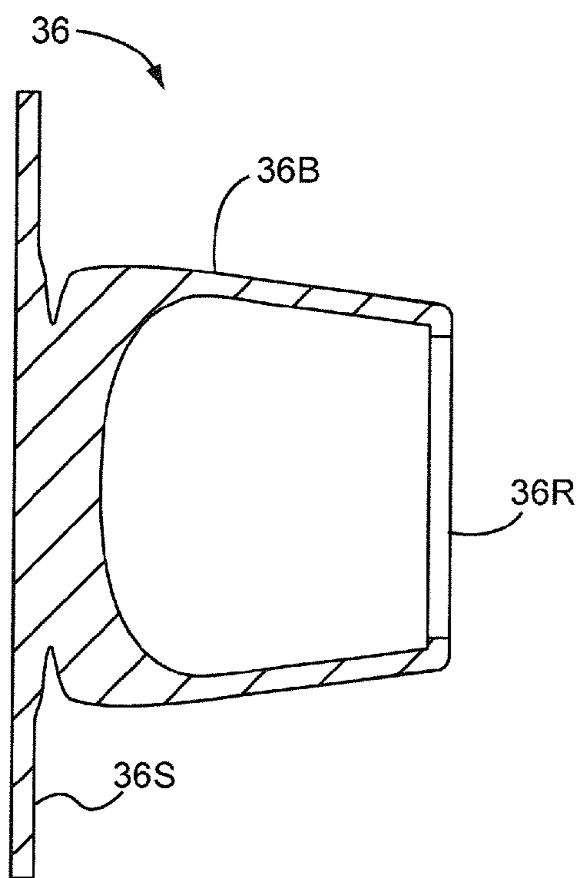
FIG. 12I SECTION E-E
