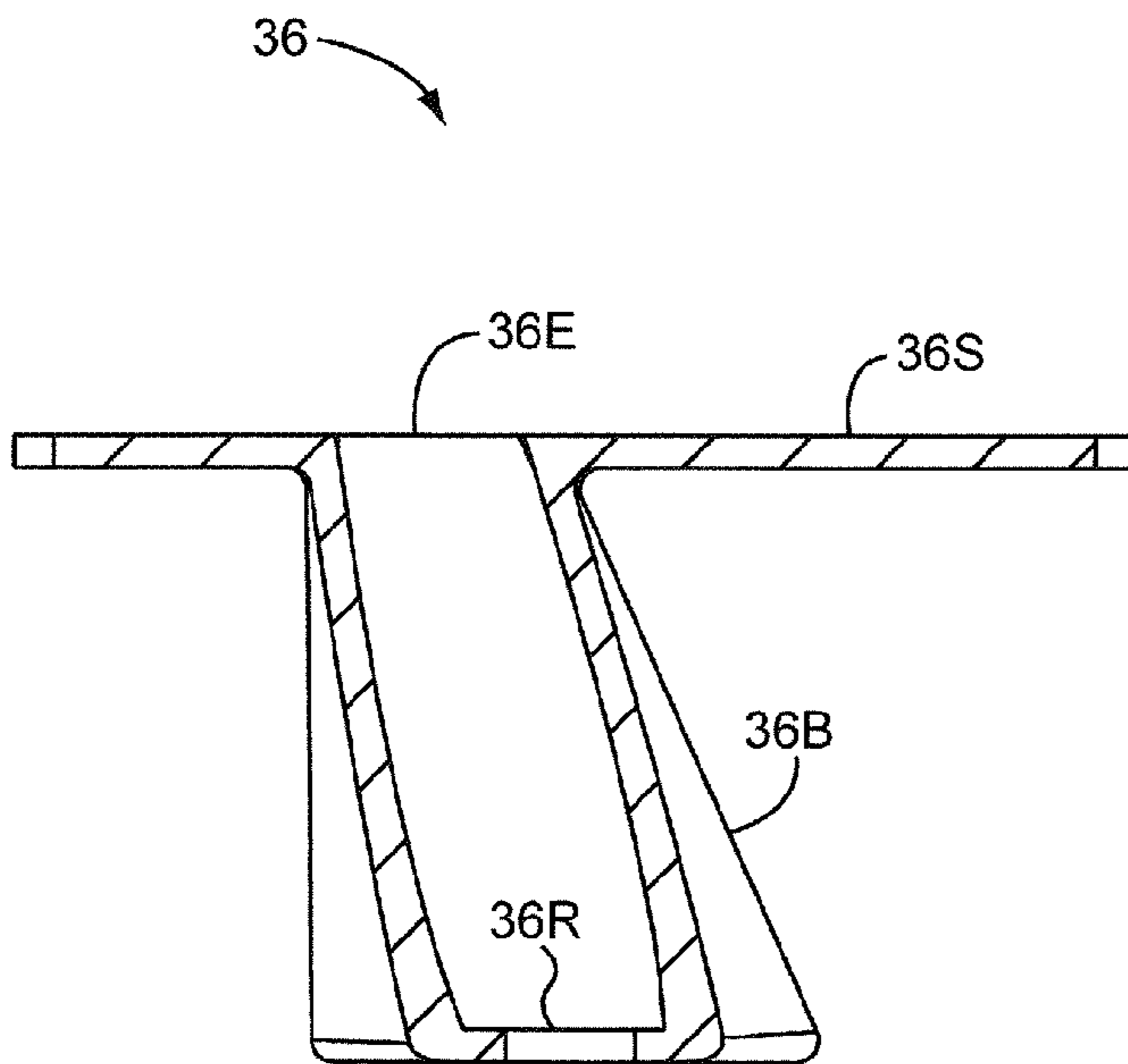
FIG. 12L SECTION H-H
