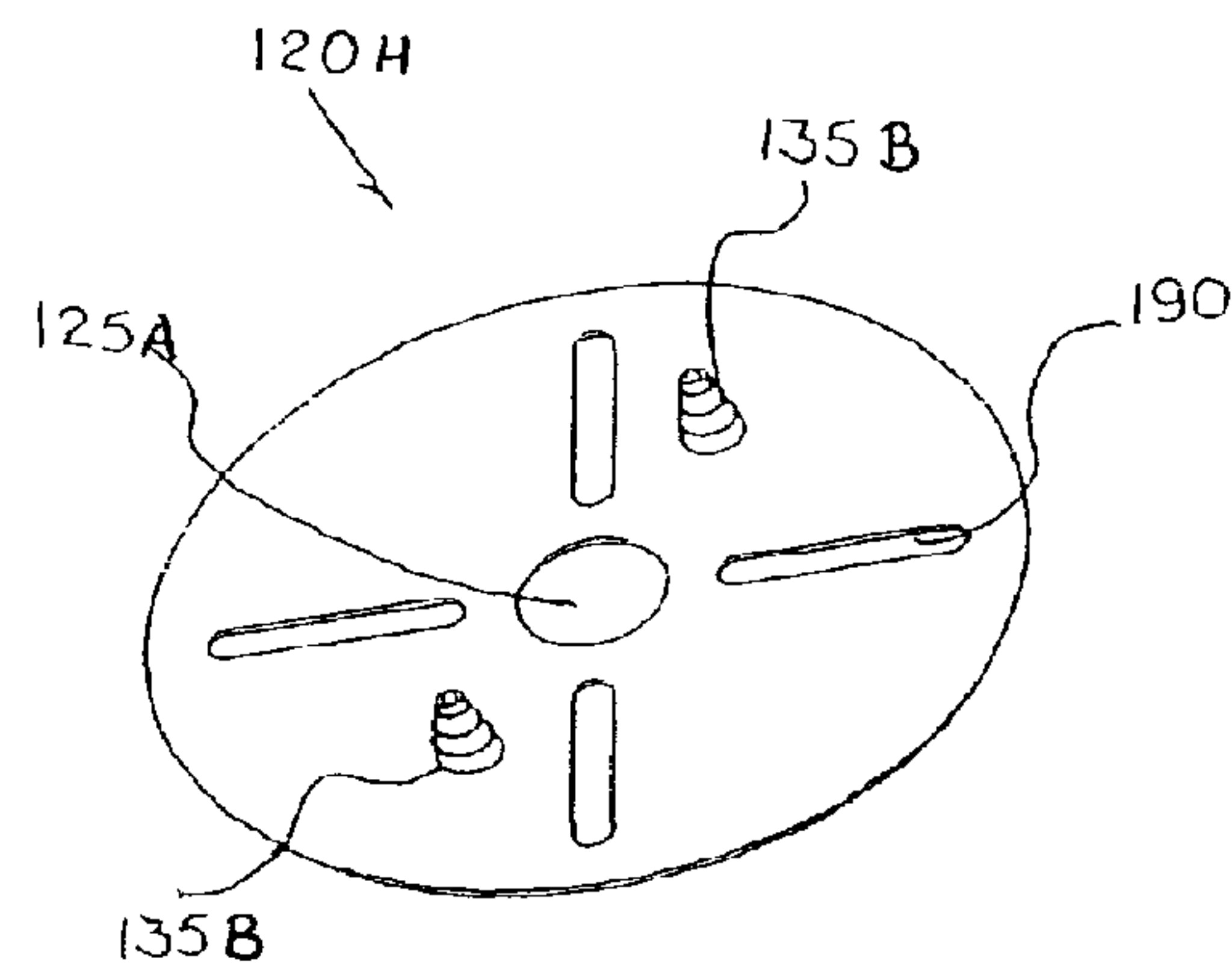
FIG. 19B
