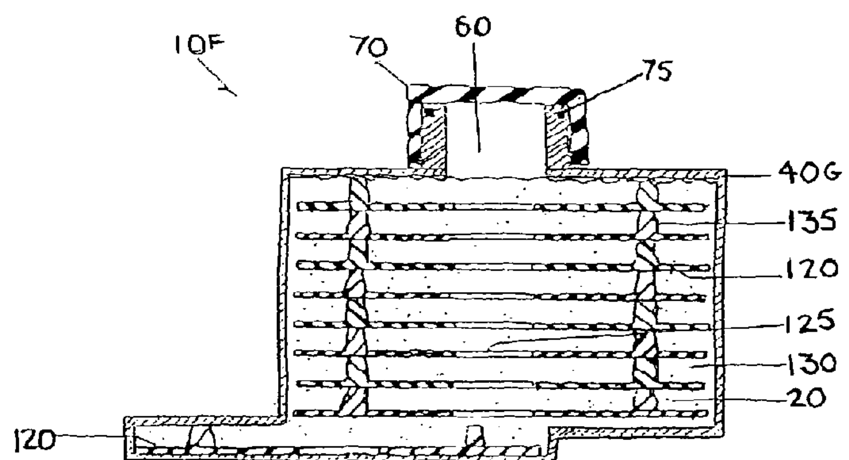
FIG. 11
