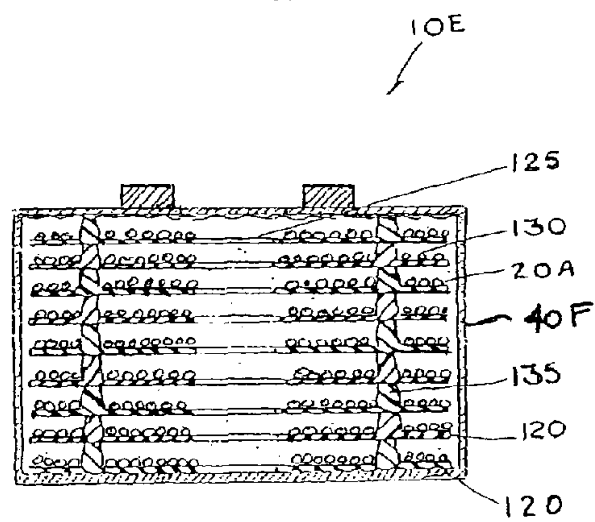
FIG. 10A
