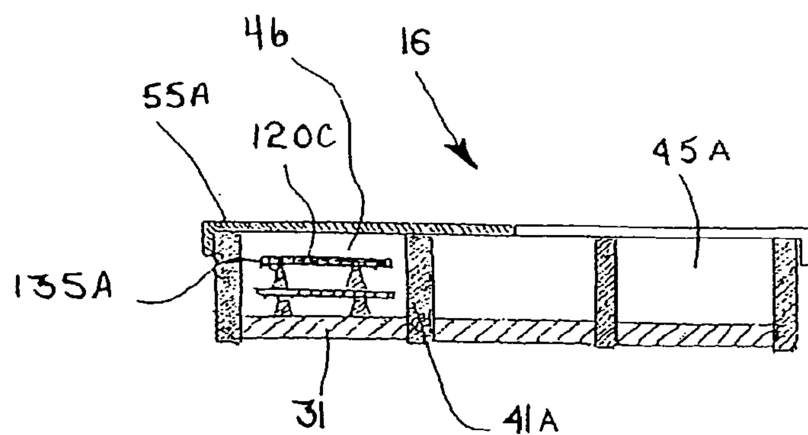
FIG. 9B
