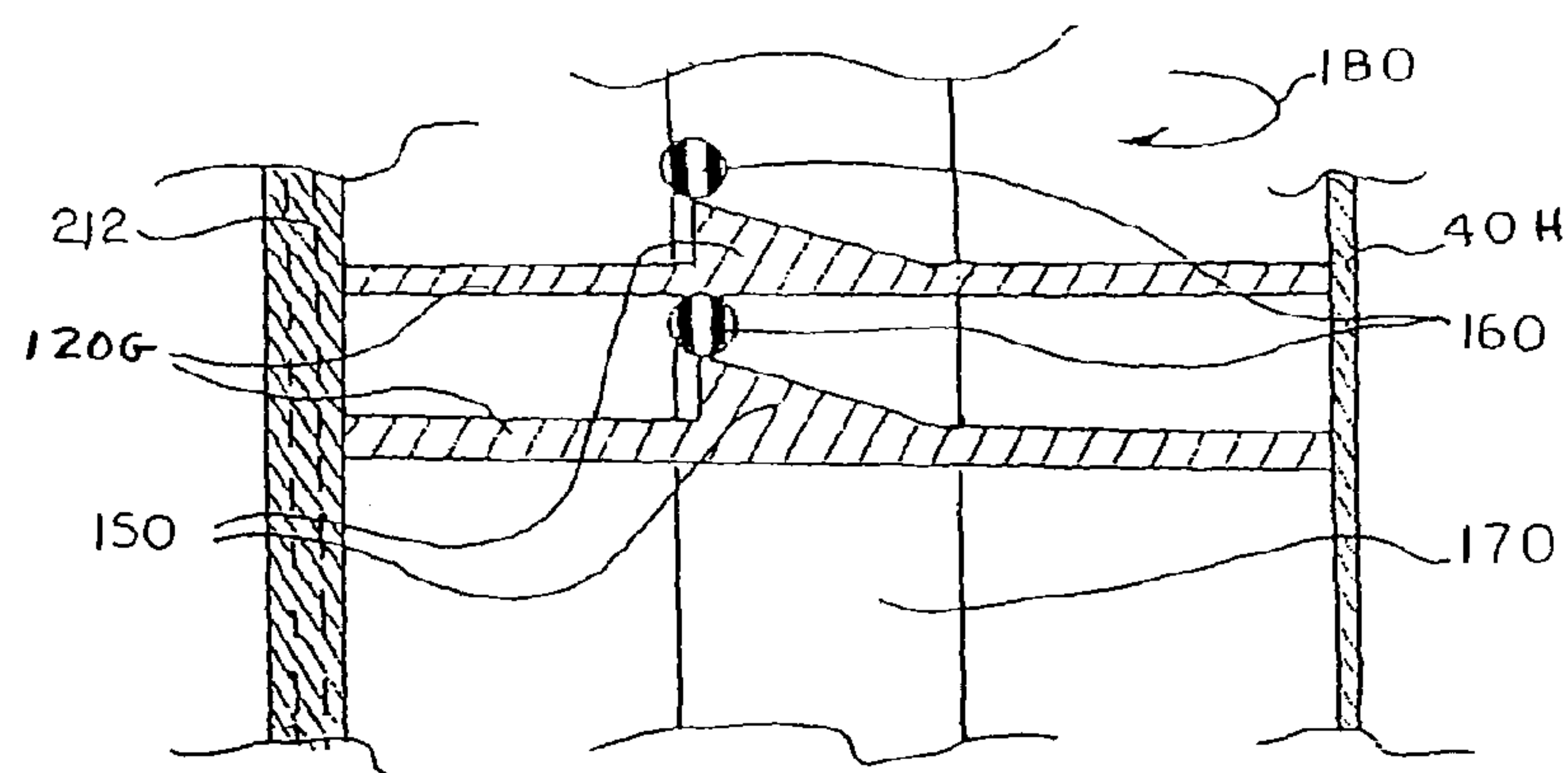
FIG. 15C
