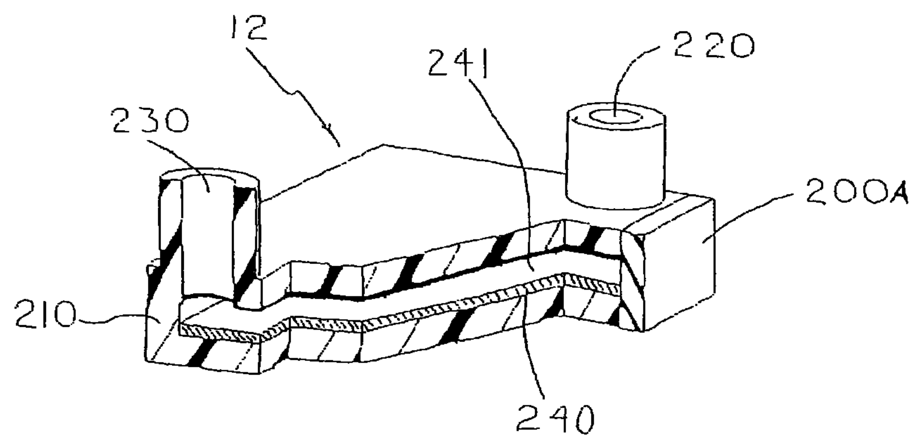
FIG. 18
