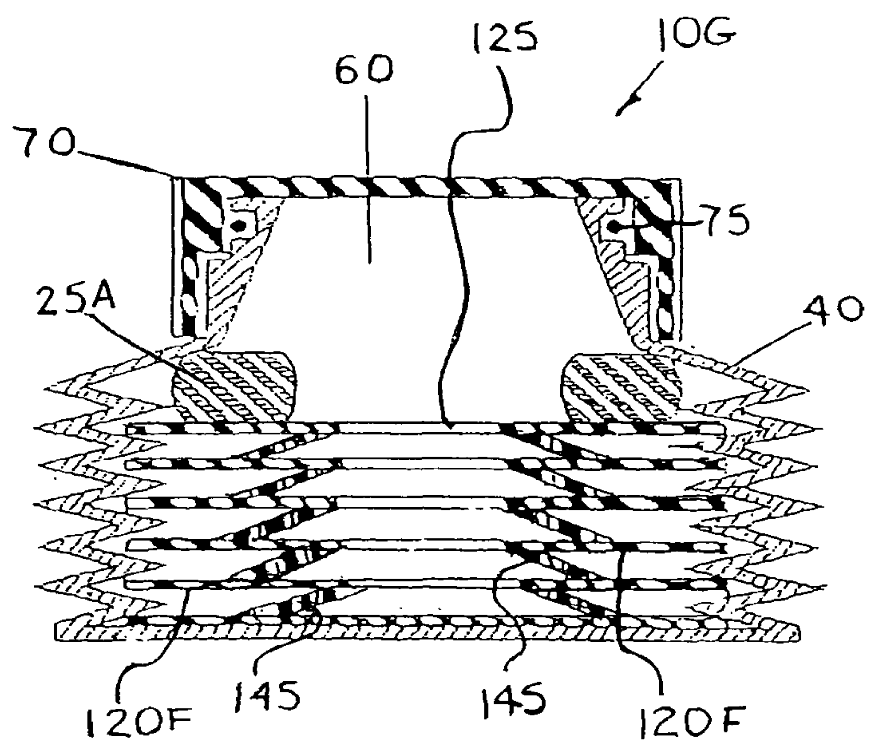
FIG. 14B
