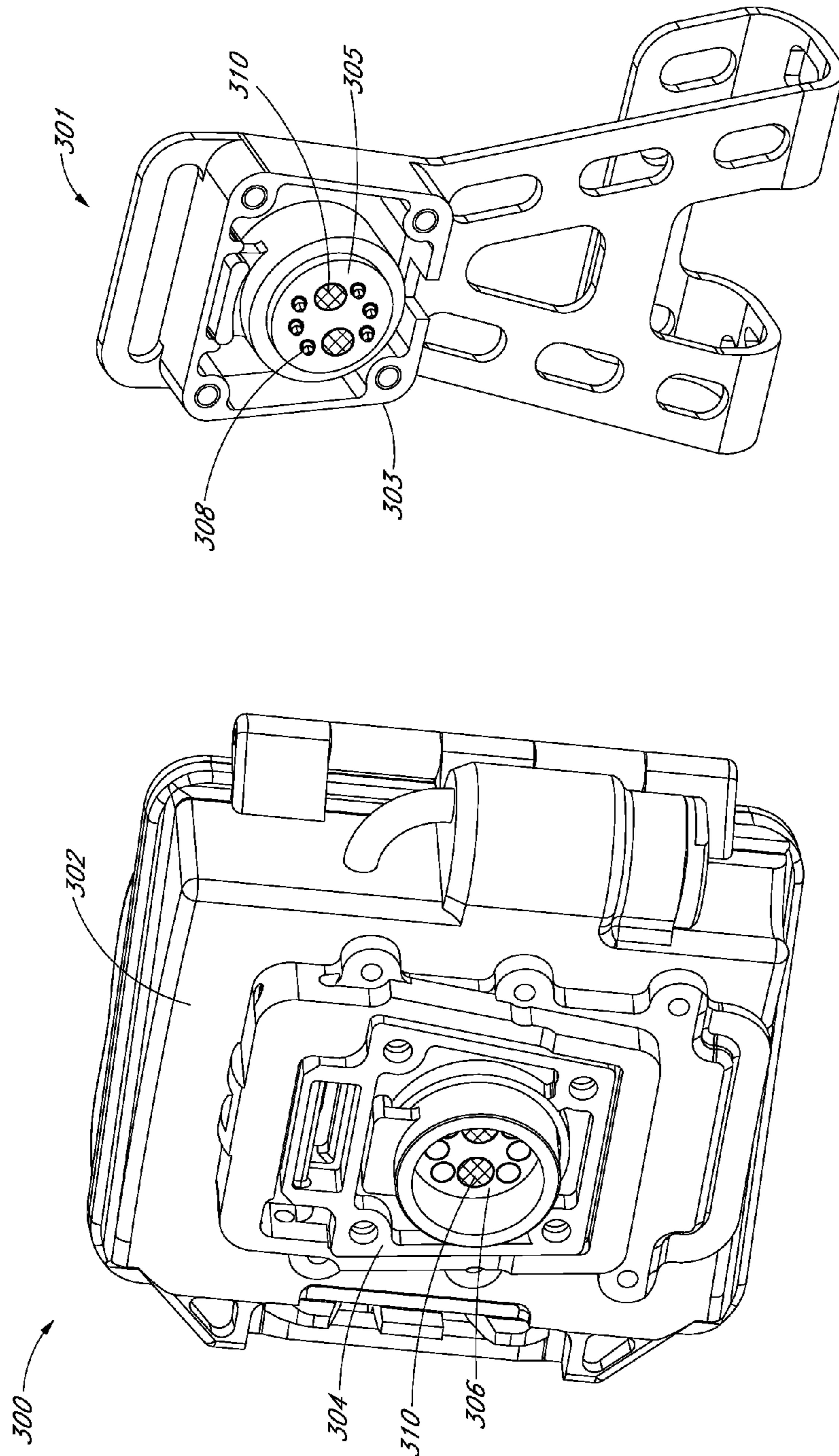
FIG. 3C
