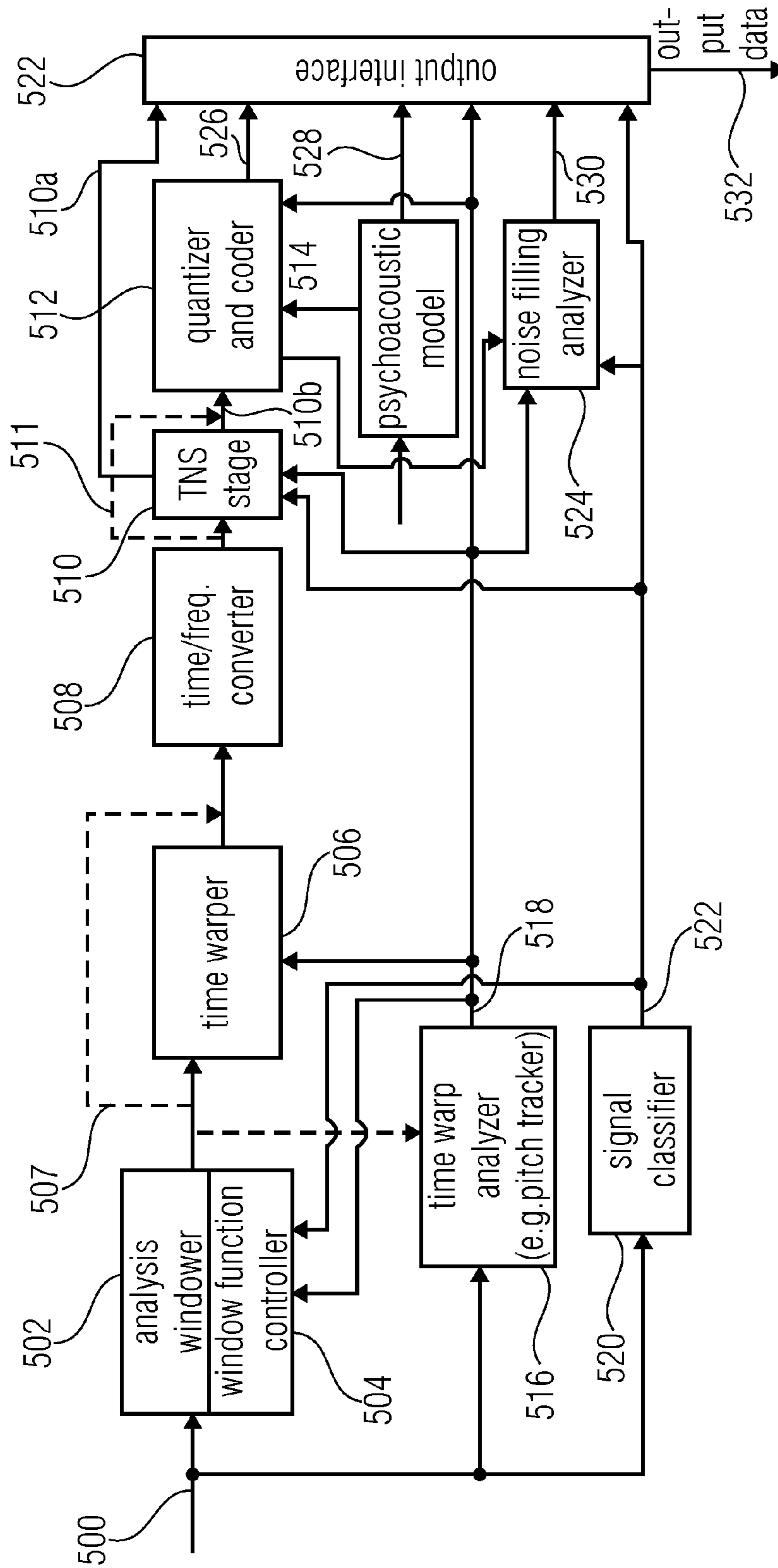
FIG 5A (ENCODER)
