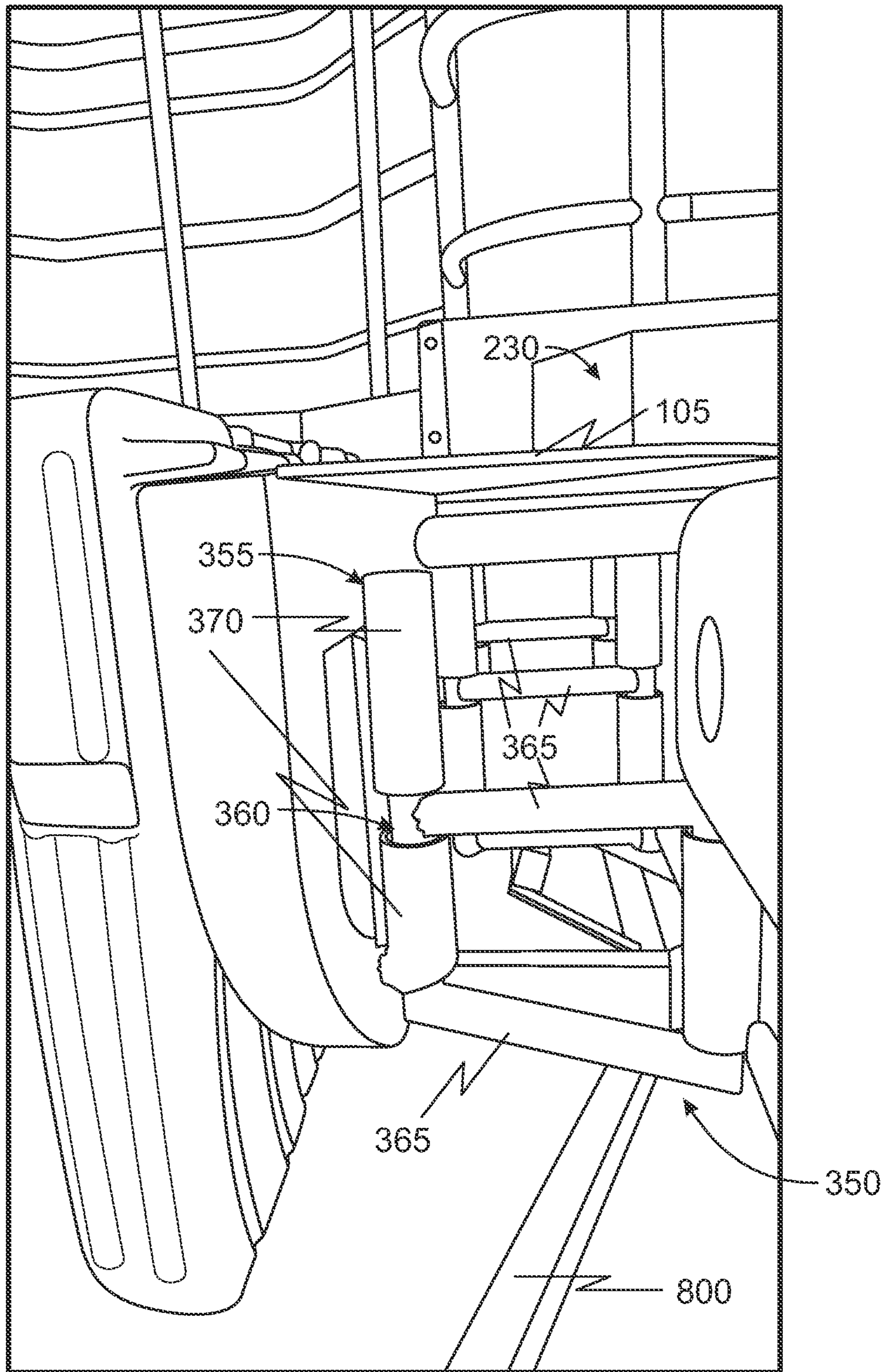
FIG. 3b
