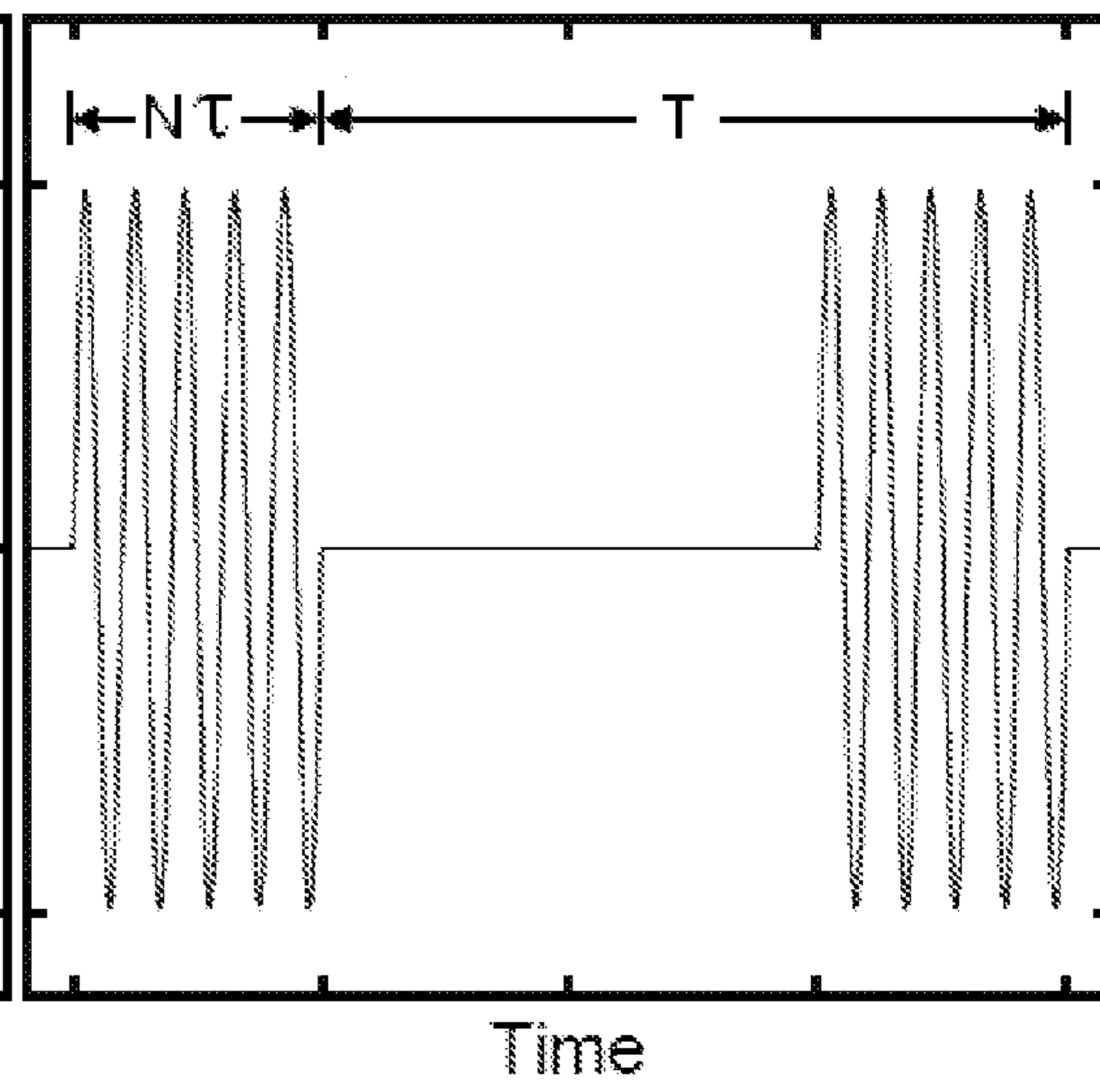
FIG. 11C
