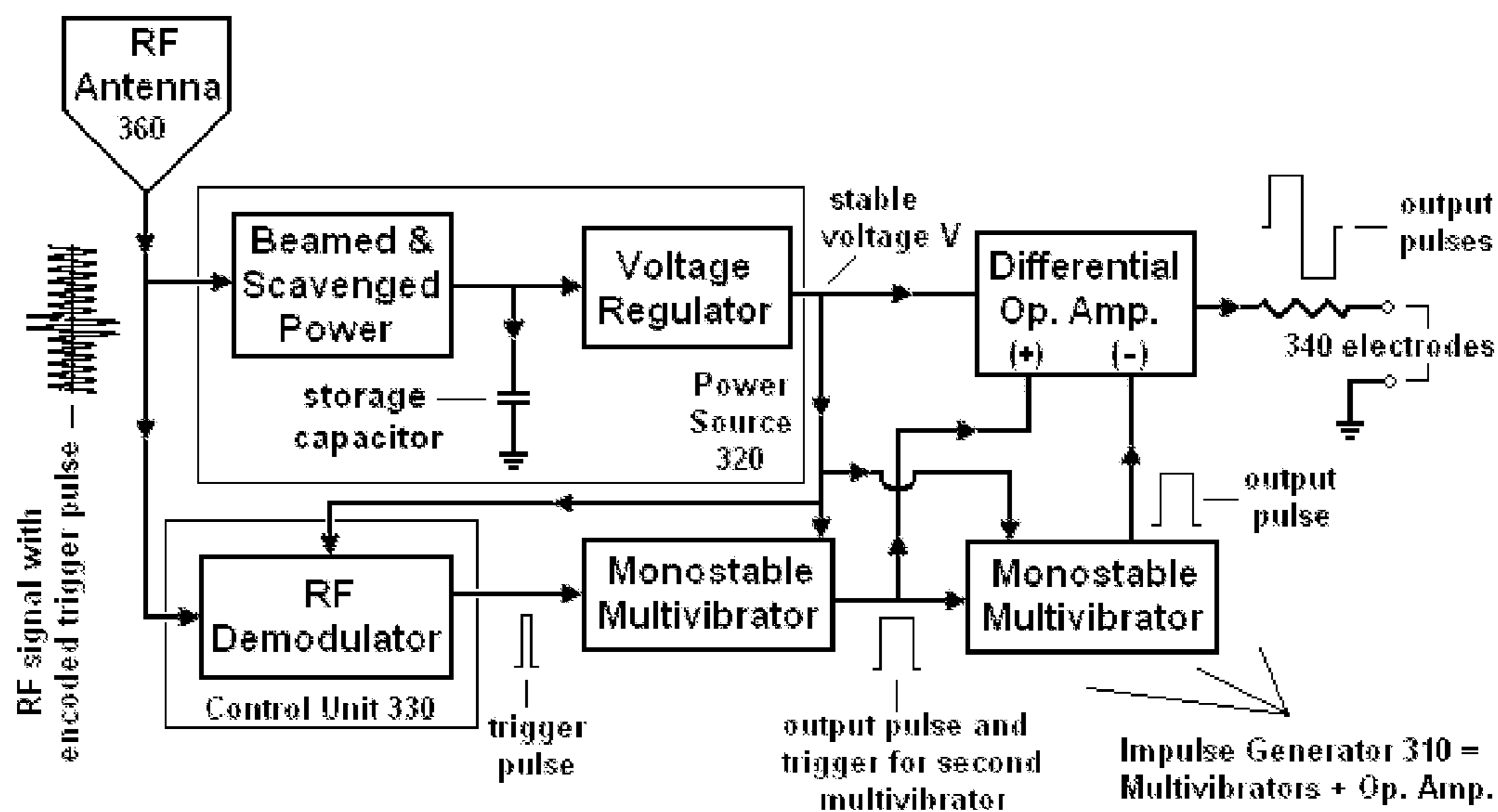
FIG. 15C
