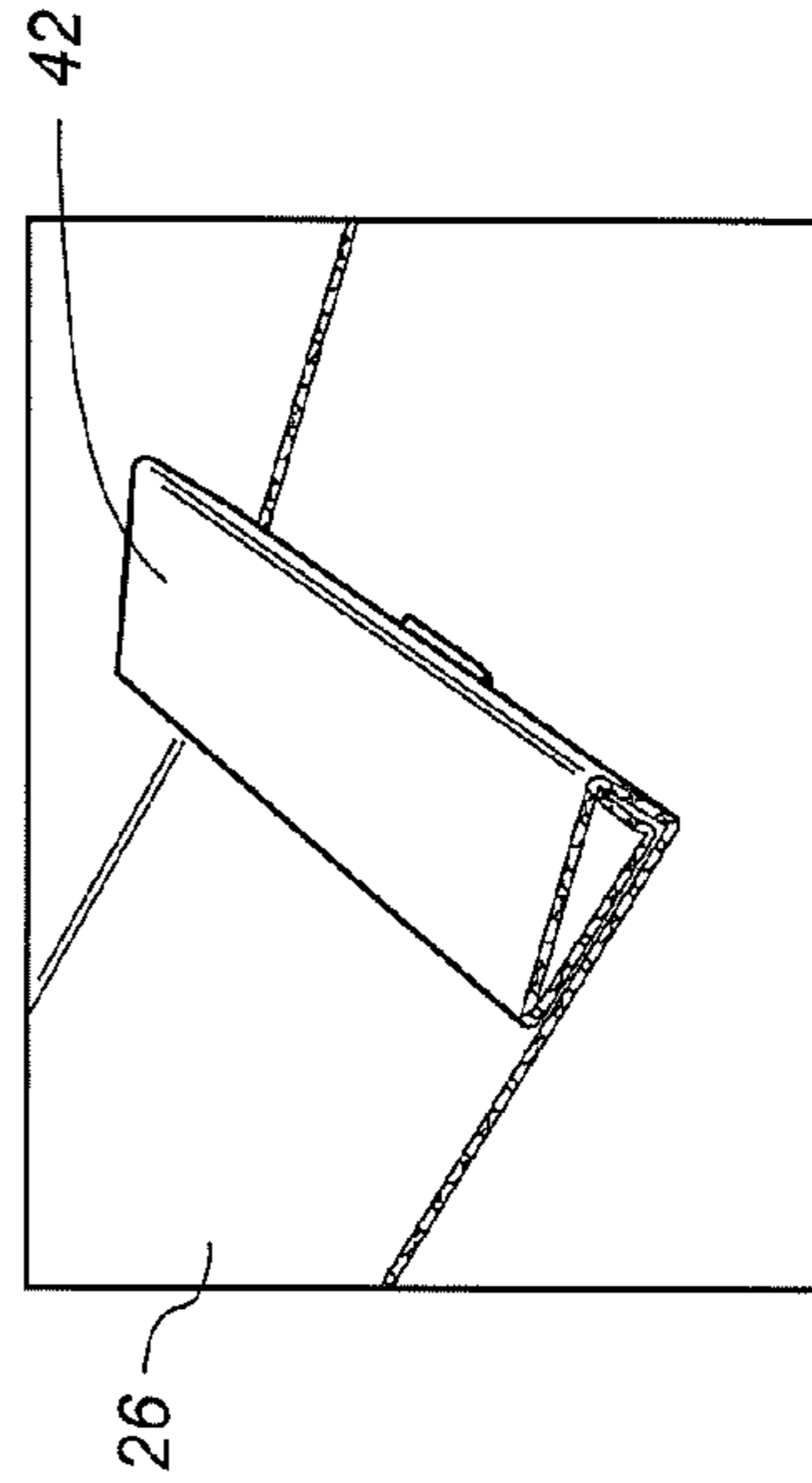
FIG. 5d
