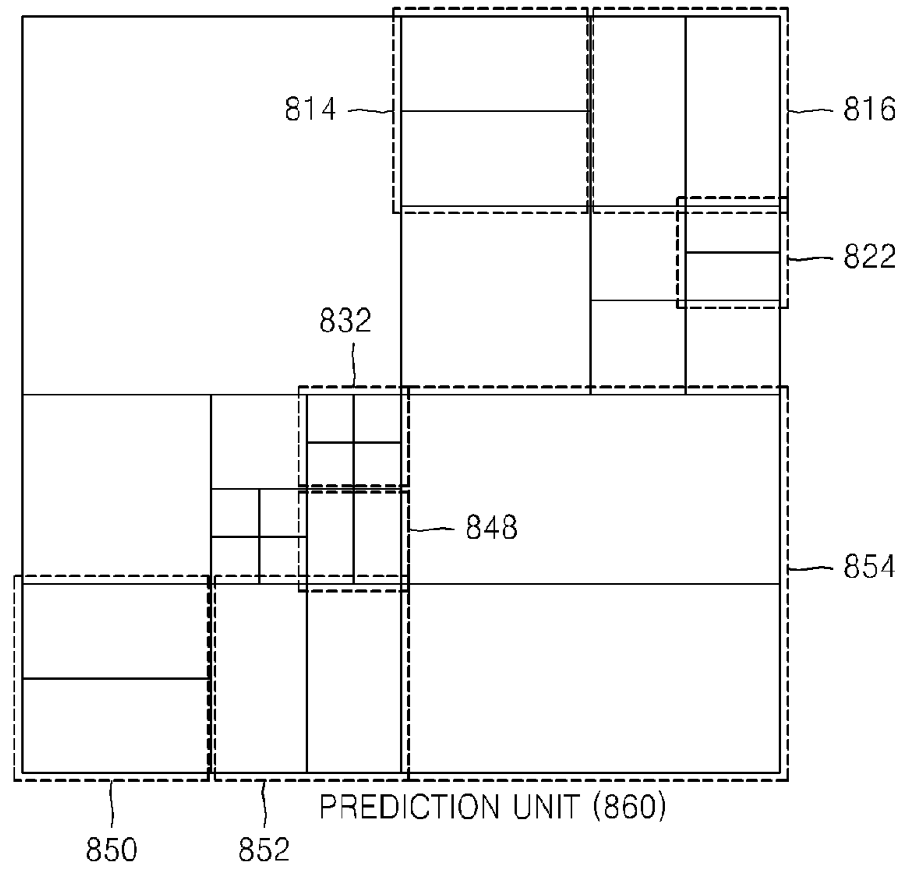
FIG. 8C
