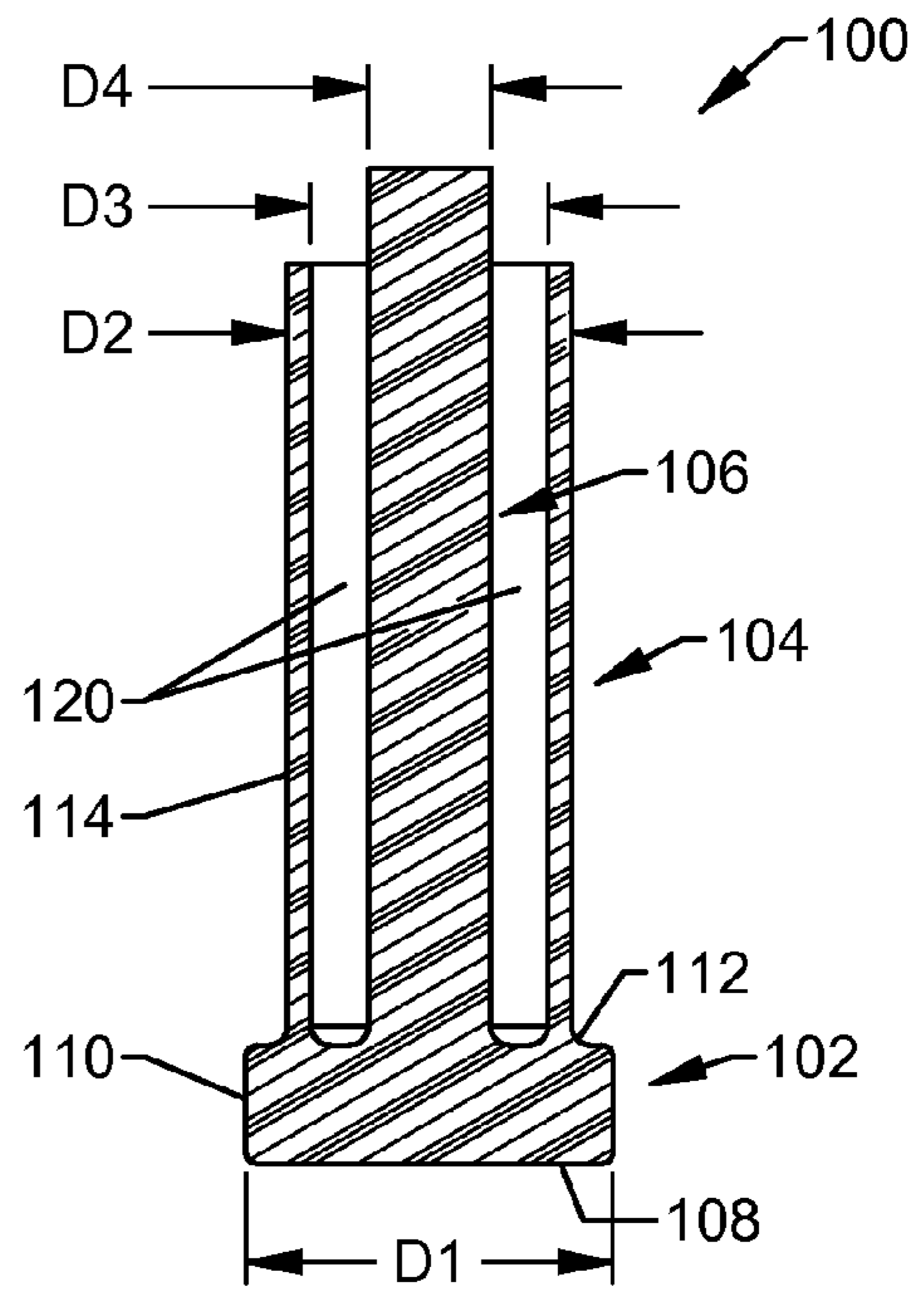
SECTION A-A
