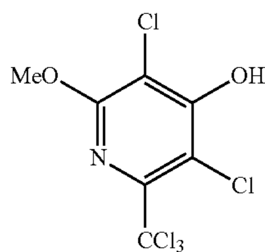
4-demethylpenclomedine (DM-PEN)
