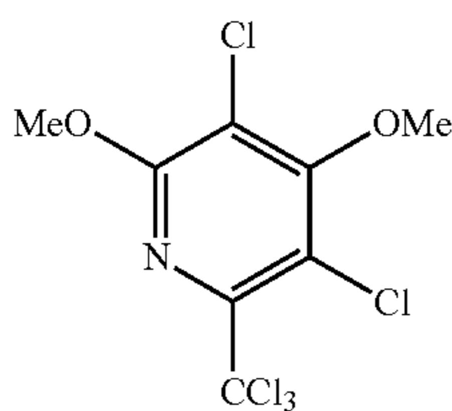
penclomedine (PEN)
