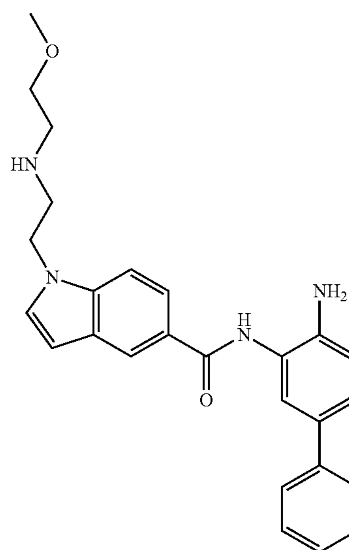
N-(4-amino-[1,1'-biphenyl]-3-yl)-1-(2-((2- methoxyethyl)amino)ethyl)-1H-indole-5- carboxamide
