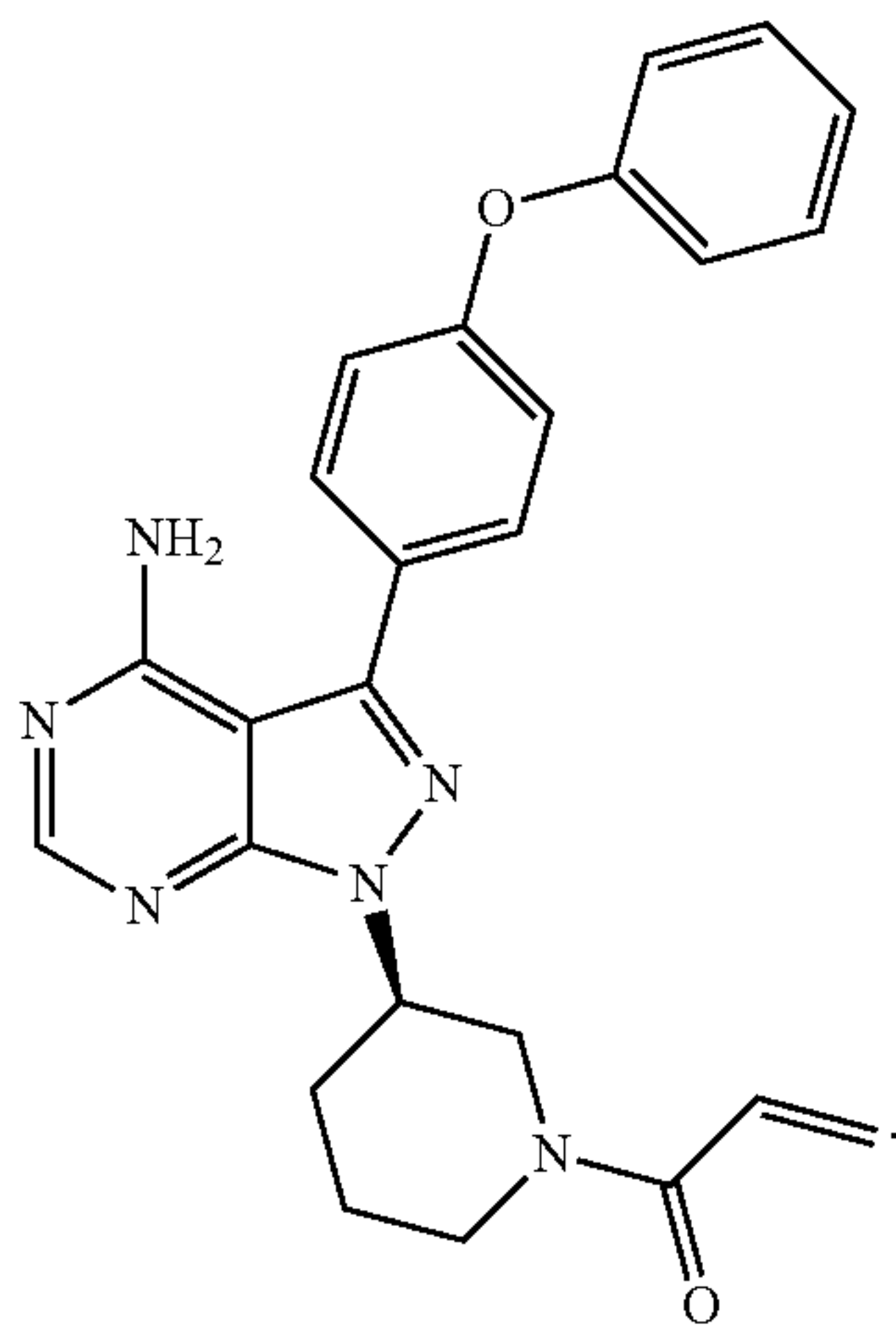
Ibrutinib
