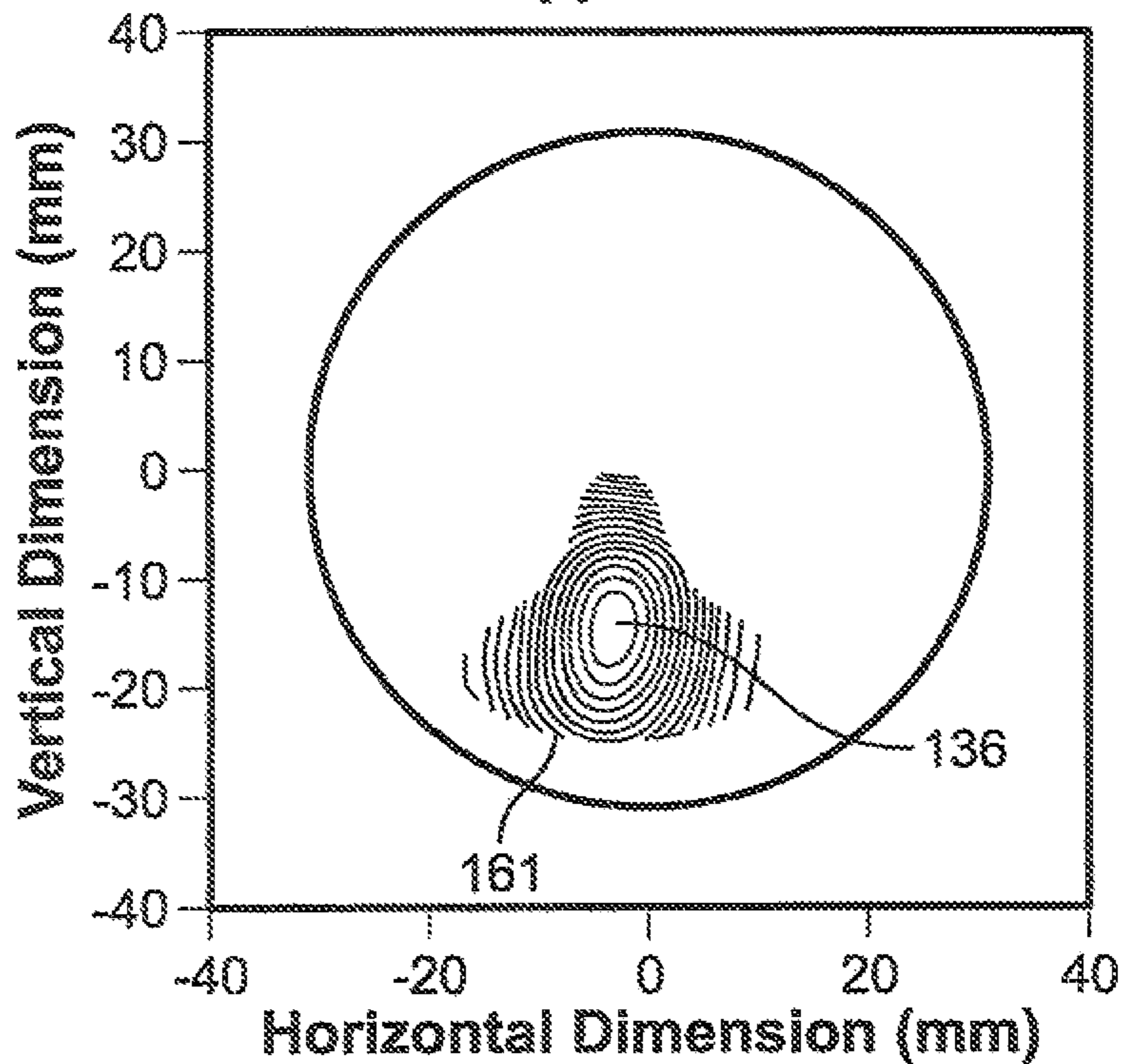
Add Power Plot: Cropped +1.00D Diffractive PAR
