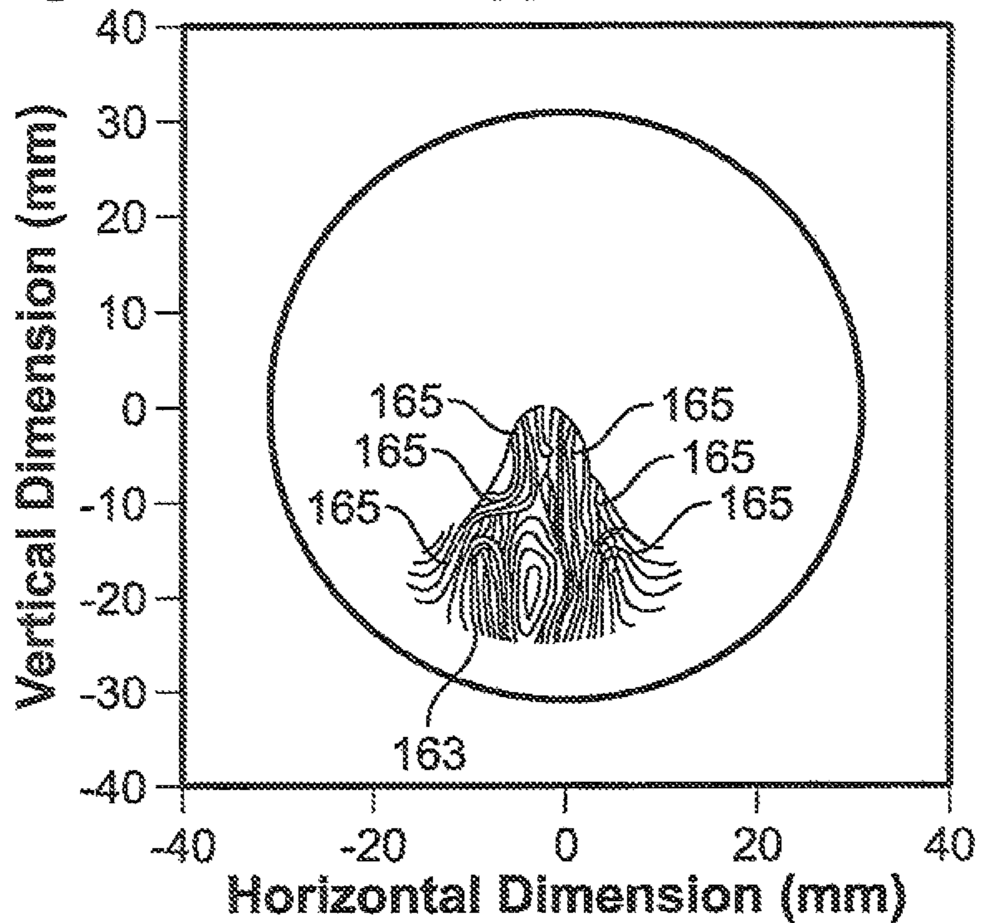
Astigmatism Plot: Cropped +1.00D Diffractive PAR
