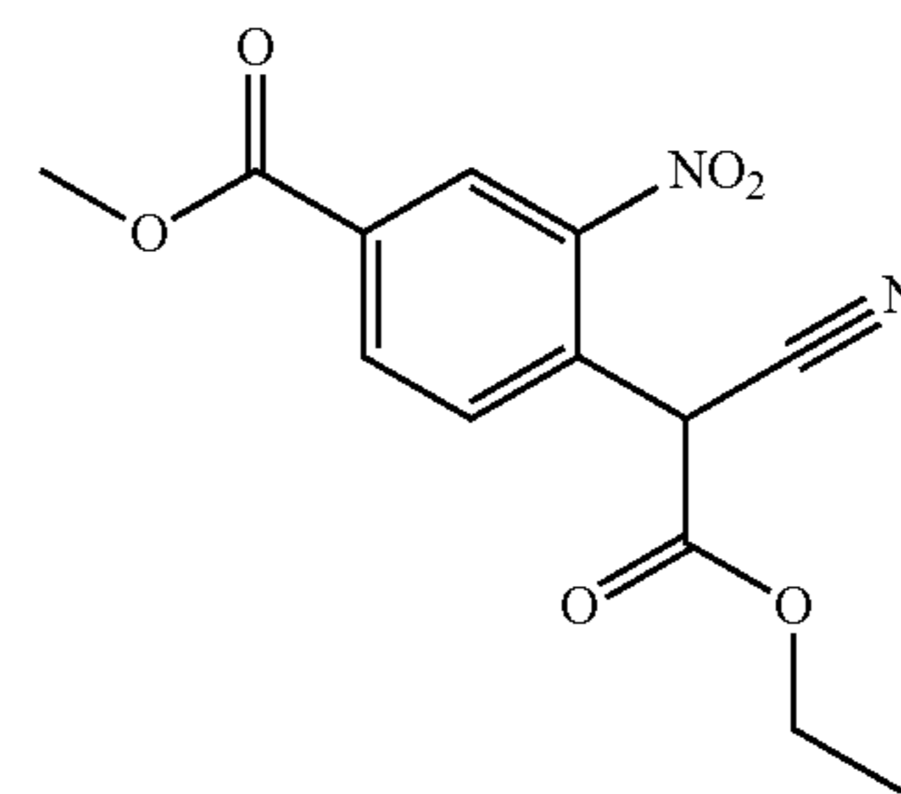
methyl 4-(1-cyano-2-ethoxy-2-oxoethyl)-3-nitrobenzoate
