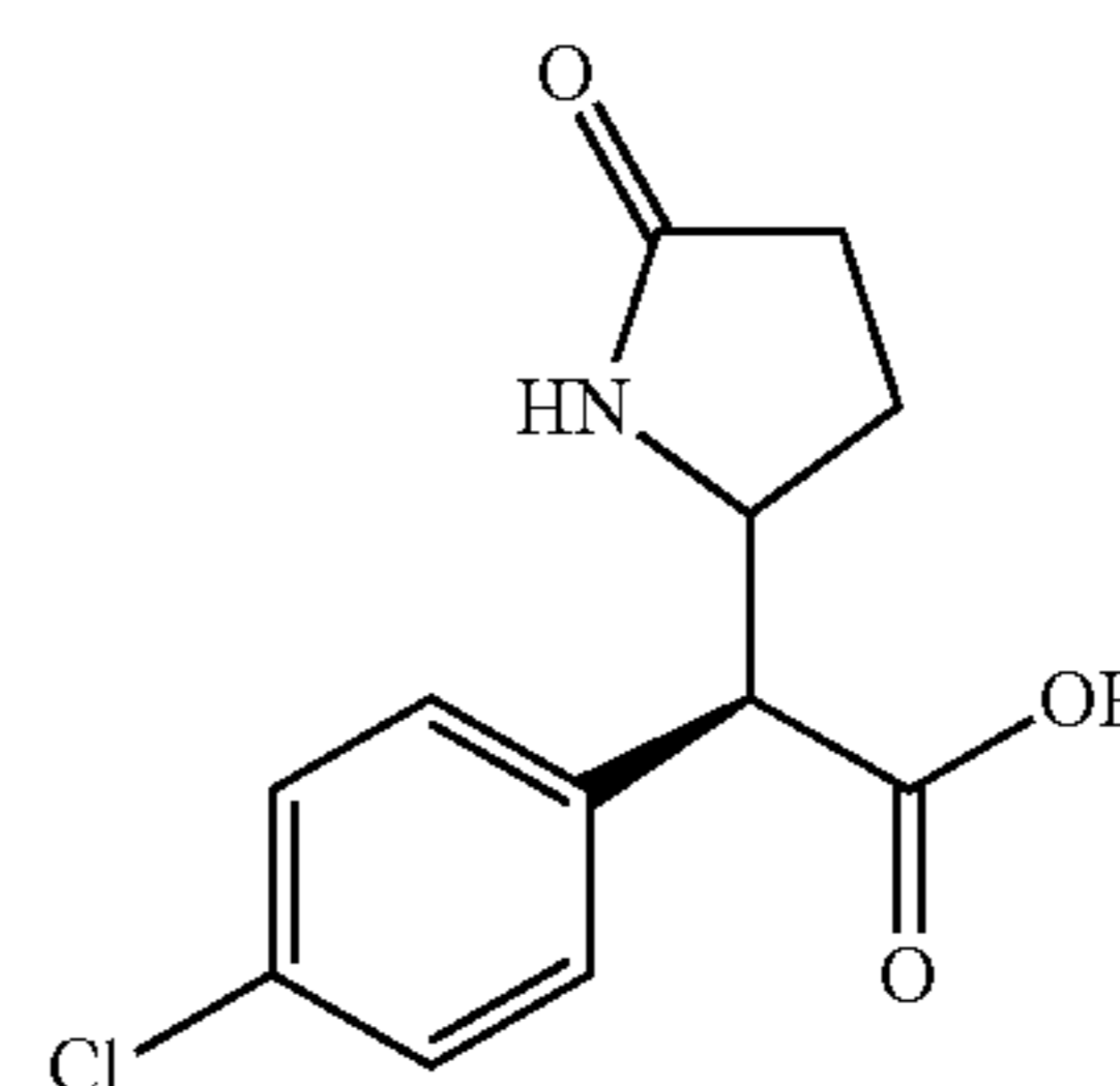
(2S)-2-(4-chlorophenyl)-2-(5-oxopyrrolidin-2-yl)acetic acid
