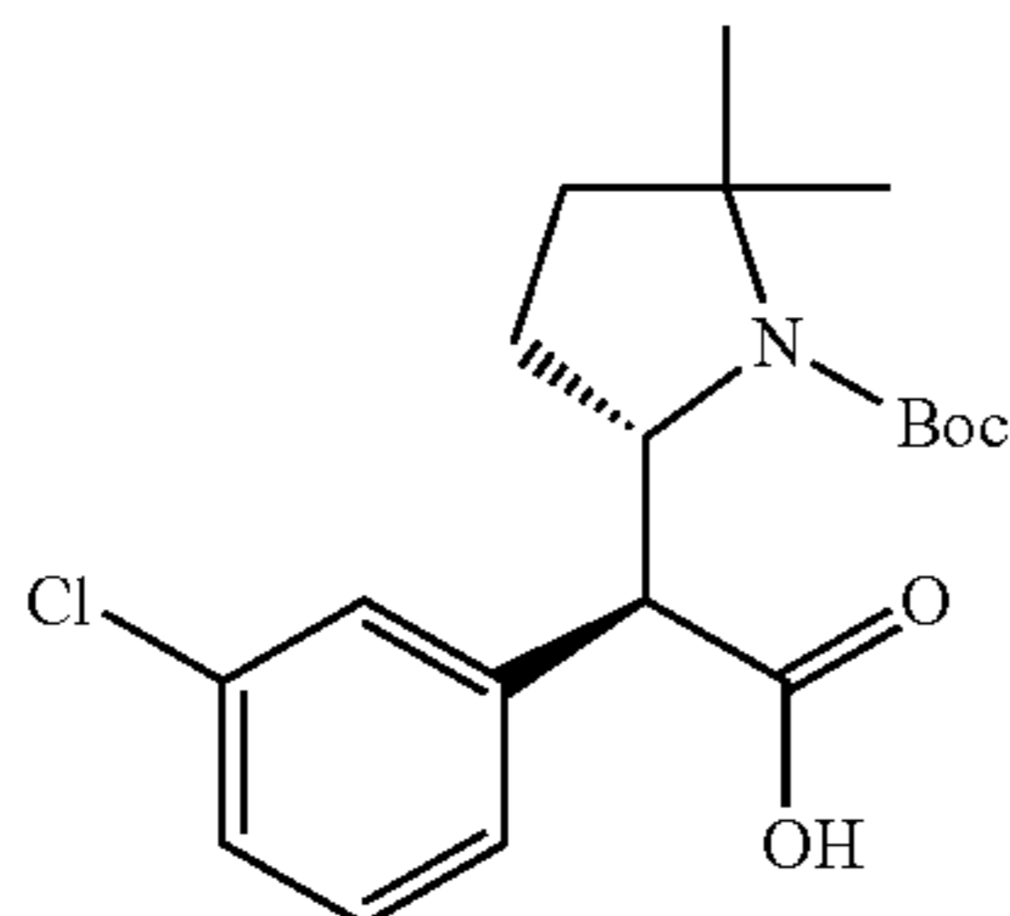
(S)-2-((S)-1-(tert-butoxycarbonyl)-5,5-dimethylpyrrolidin-2-yl)-2-(3-chlorophenyl)acetic acid
