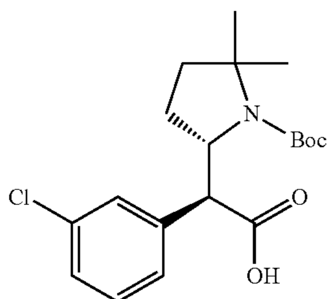
(S)-2-((S)-1-(tert-butoxycarbonyl)-5,5-dimethylpyrrolidin-2-yl)-2-(3-chlorophenyl)acetic acid
