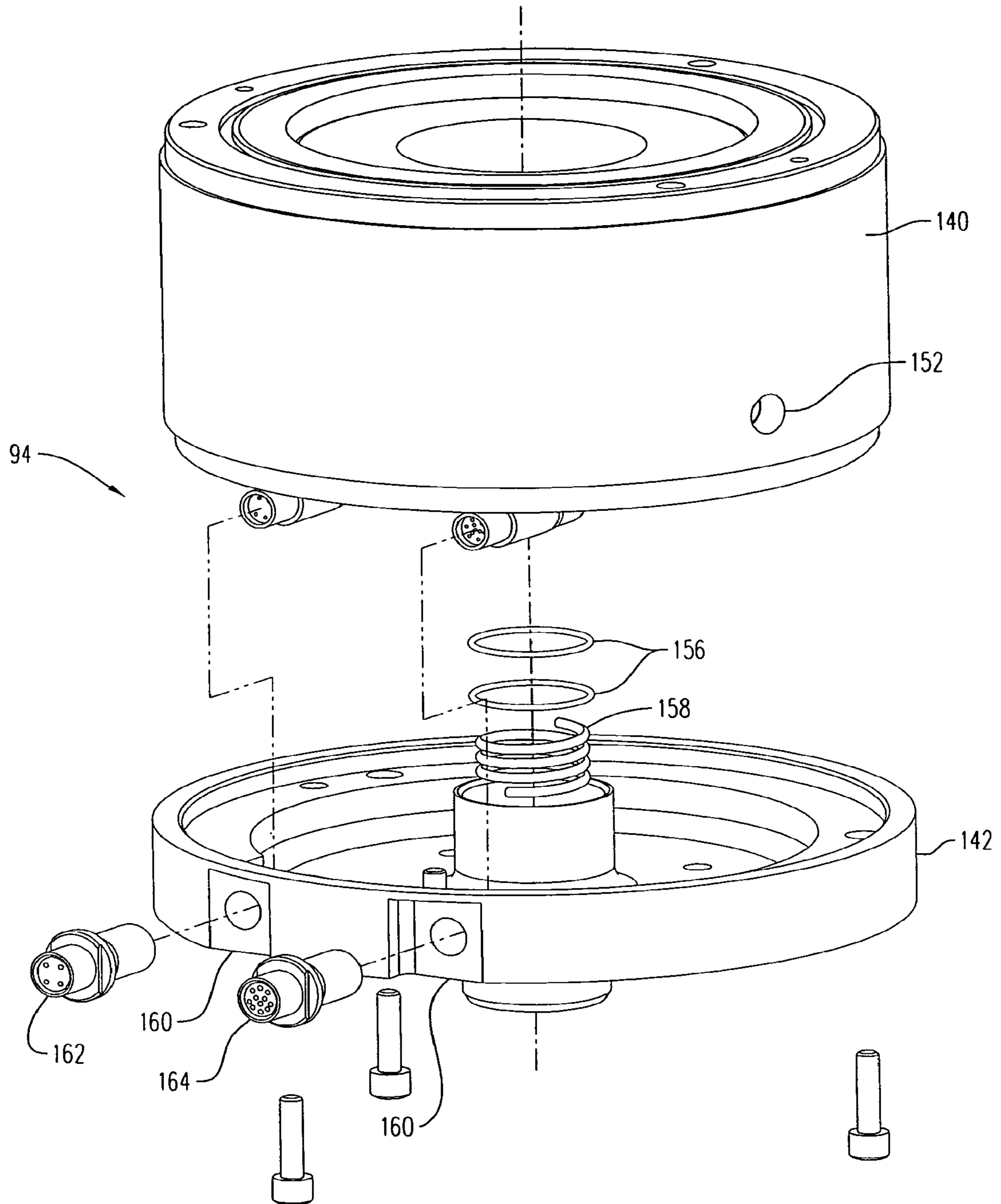
FIG. 16
