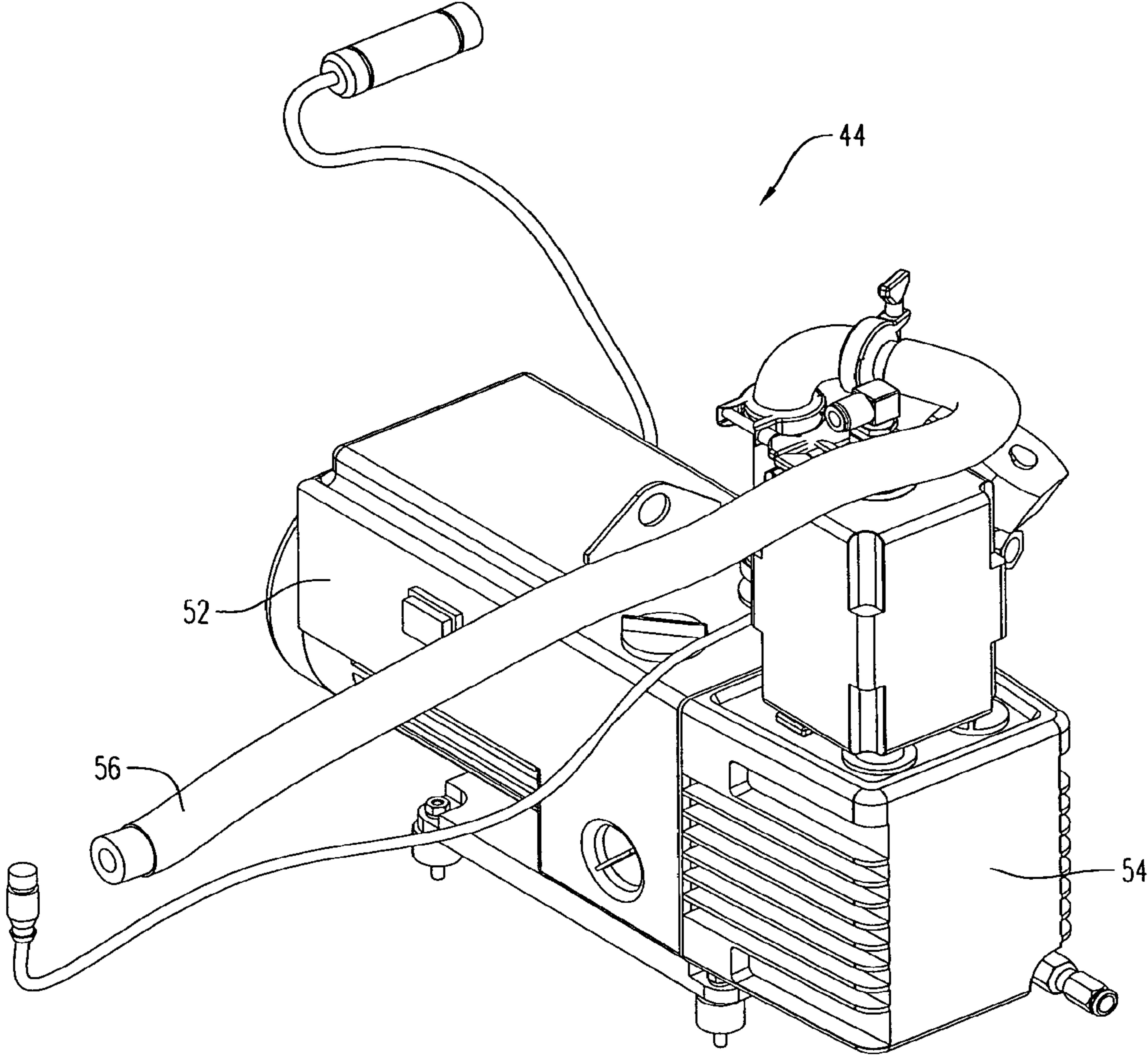
FIG. 6
