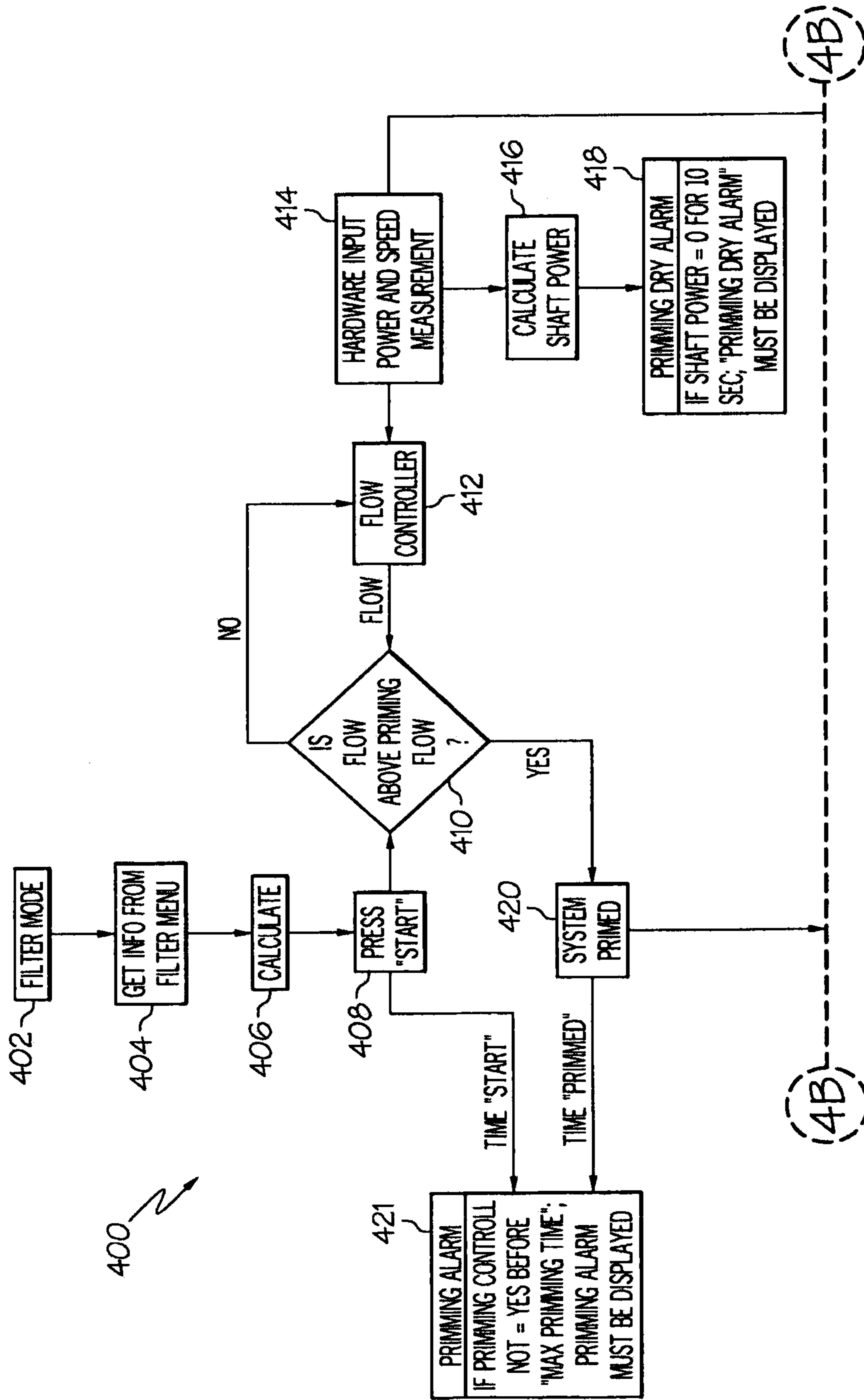
FIG. 4A
