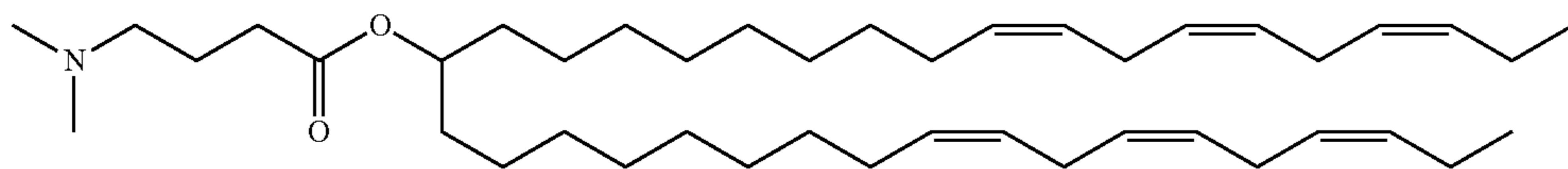
LenMC3
