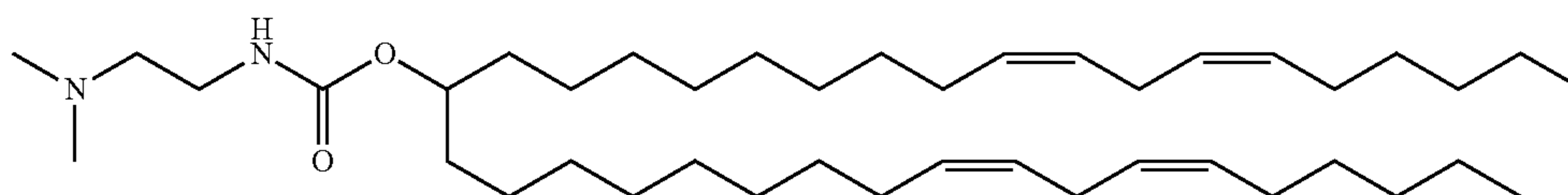
MC2C
