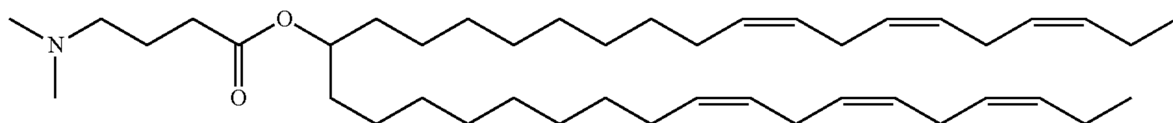
LenMC3
