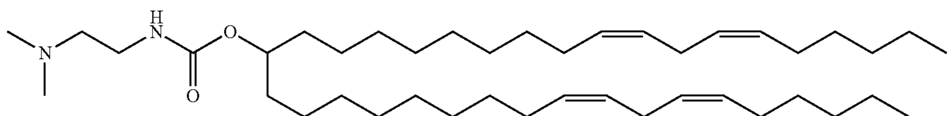
MC2C
