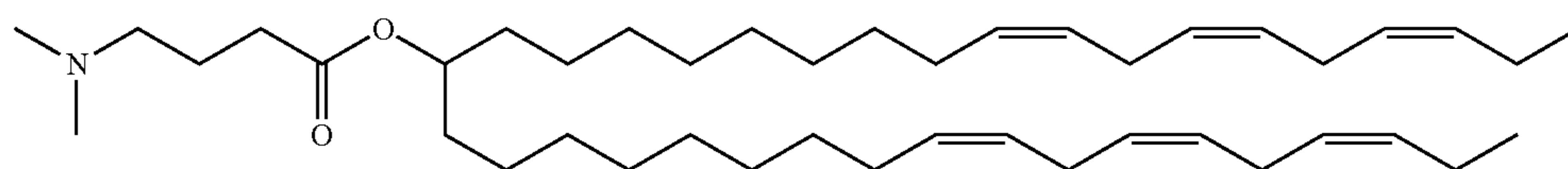
LenMC3
