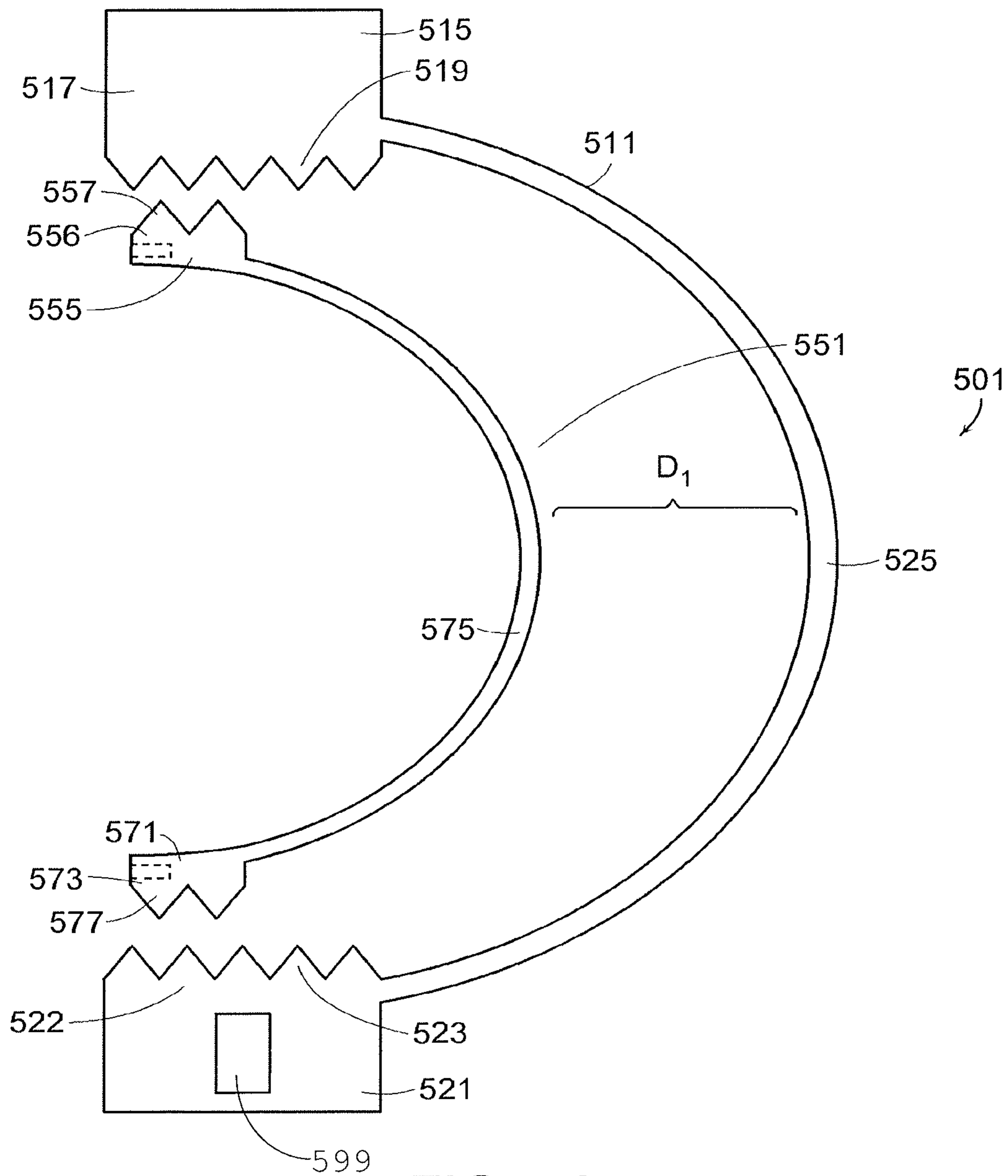
FIG. 5A
