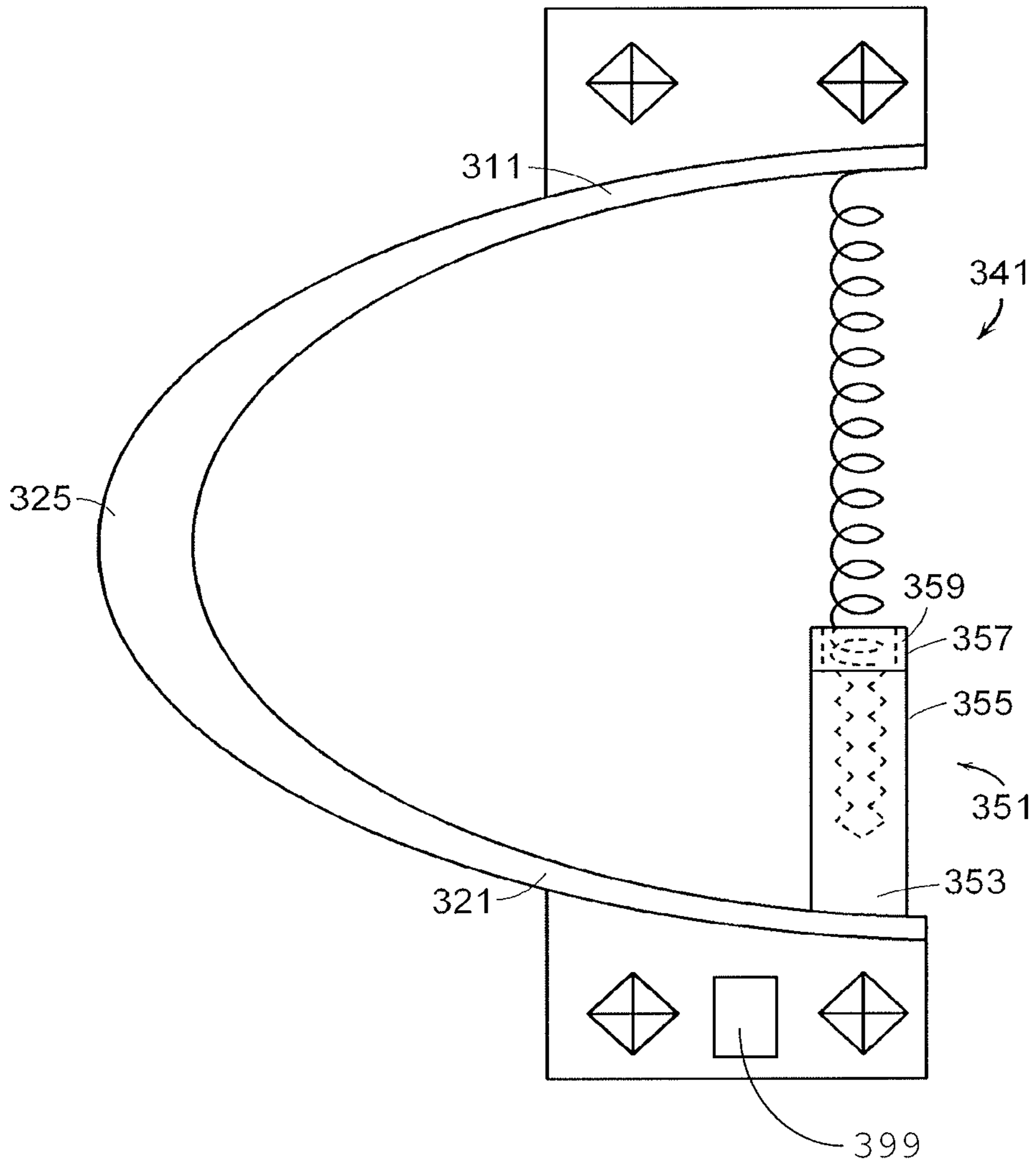
FIG. 3B
