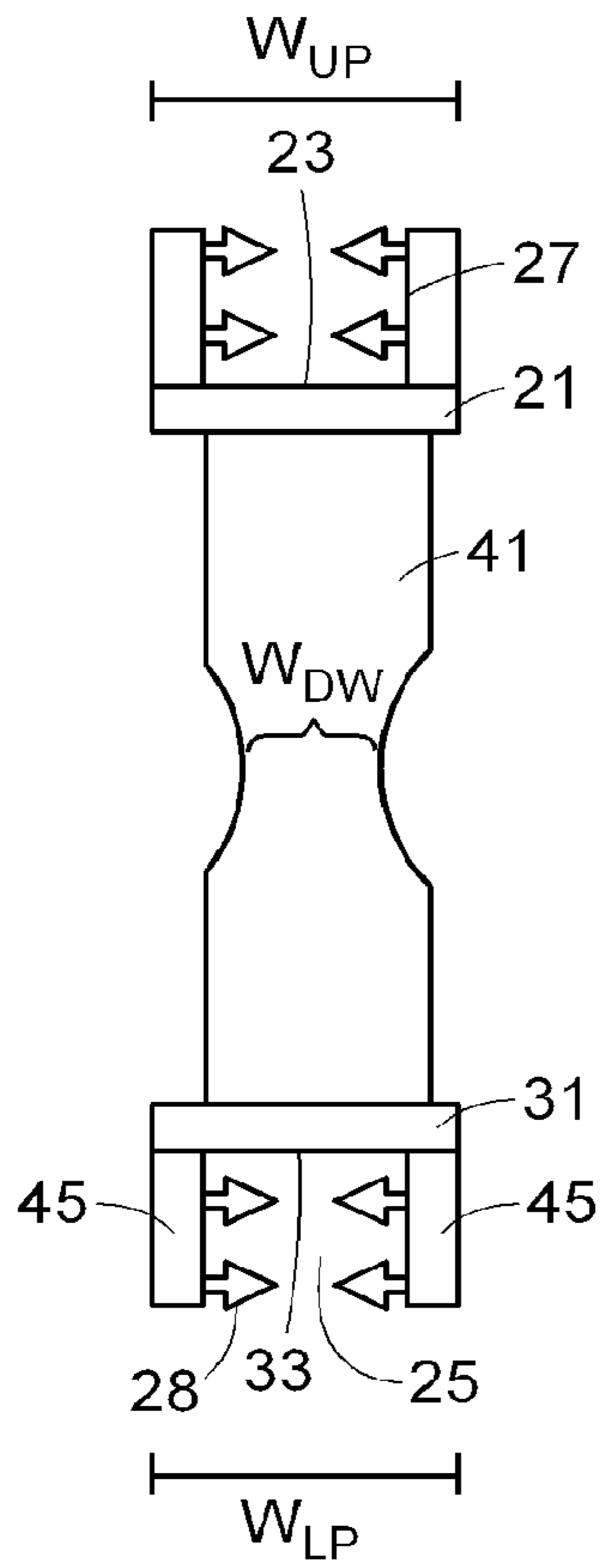
FIG. 1A
