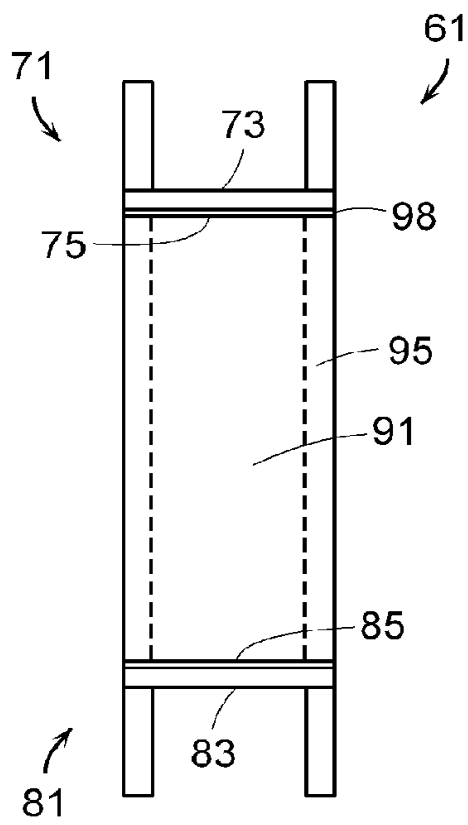
FIG. 2A
