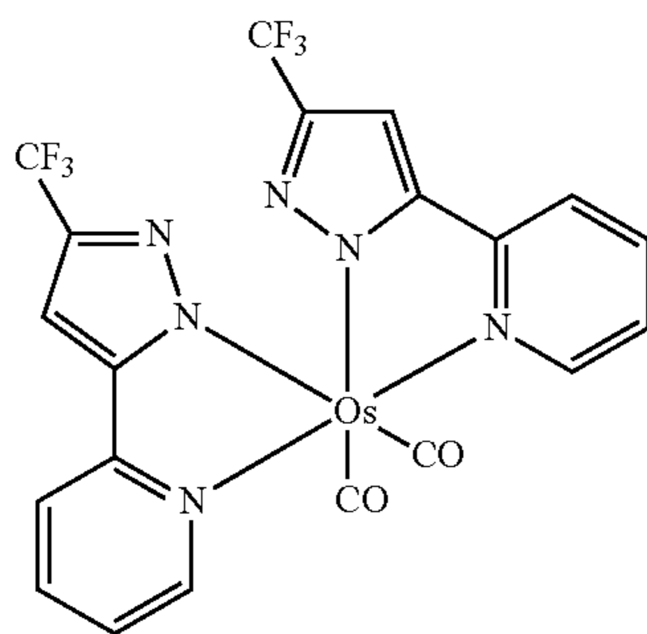
Os(fppz) 2 (CO) 2
