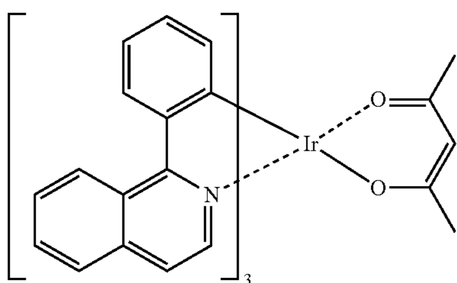
Btp 2 Ir(acac)
