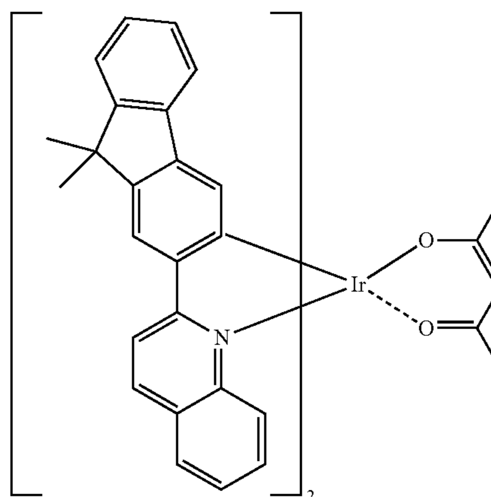
Ir(flq) 2 (acac)
