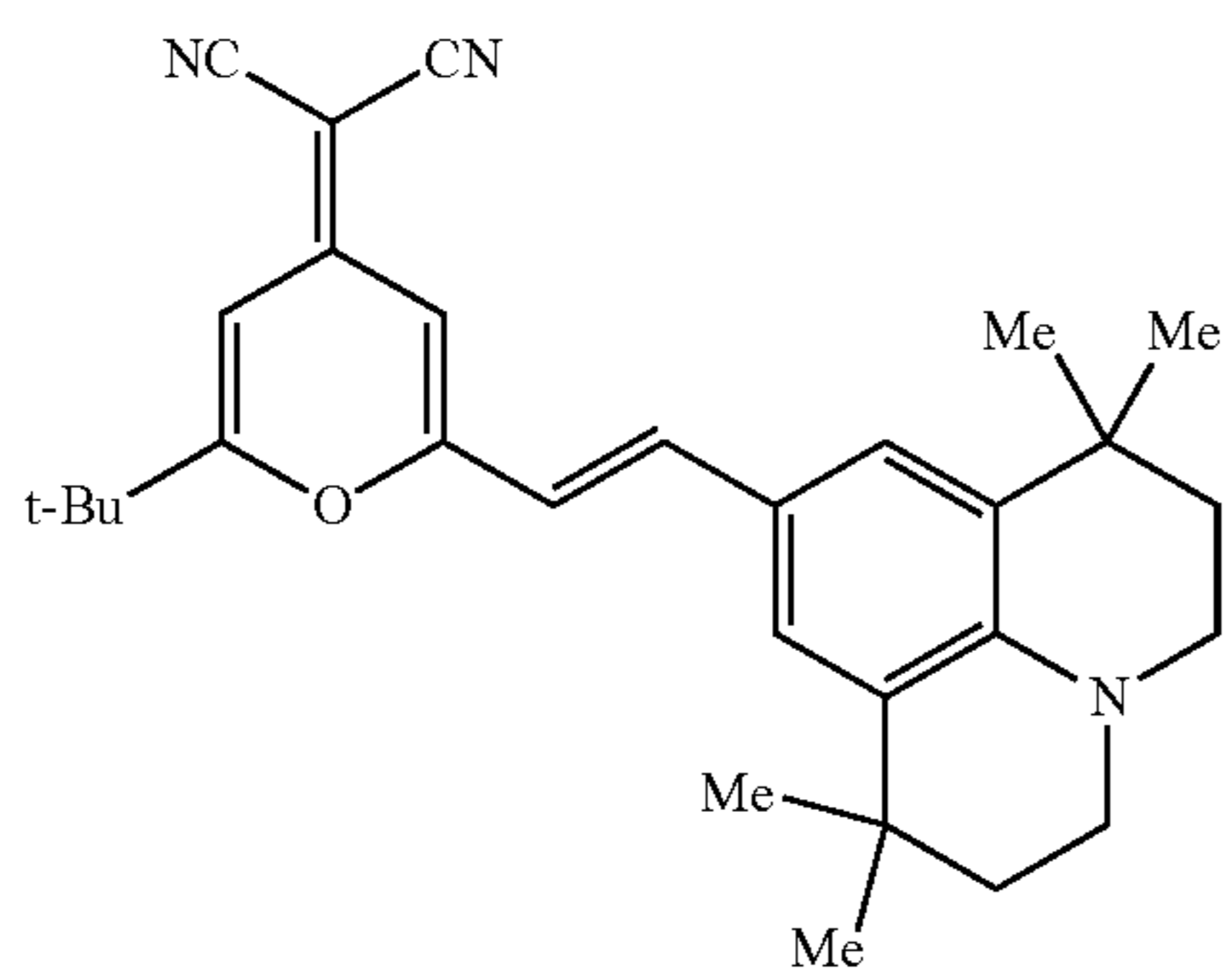
DCJTb
