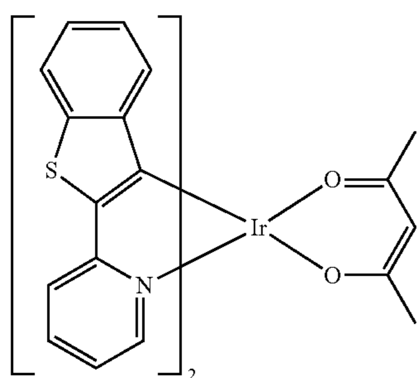
Btp 2 Ir(acac)
