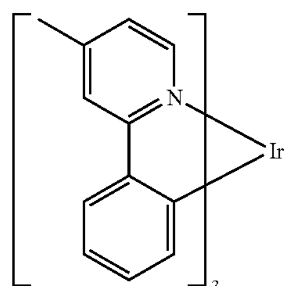
Ir(mppy) 3
