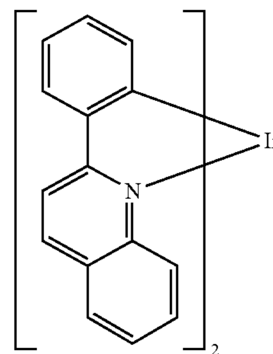
Ir(2-phq) 3
