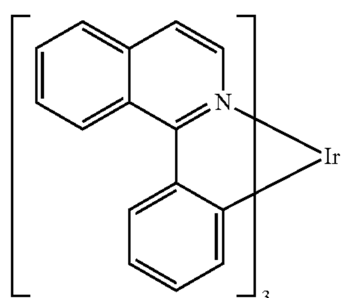
Ir(piq) 3
