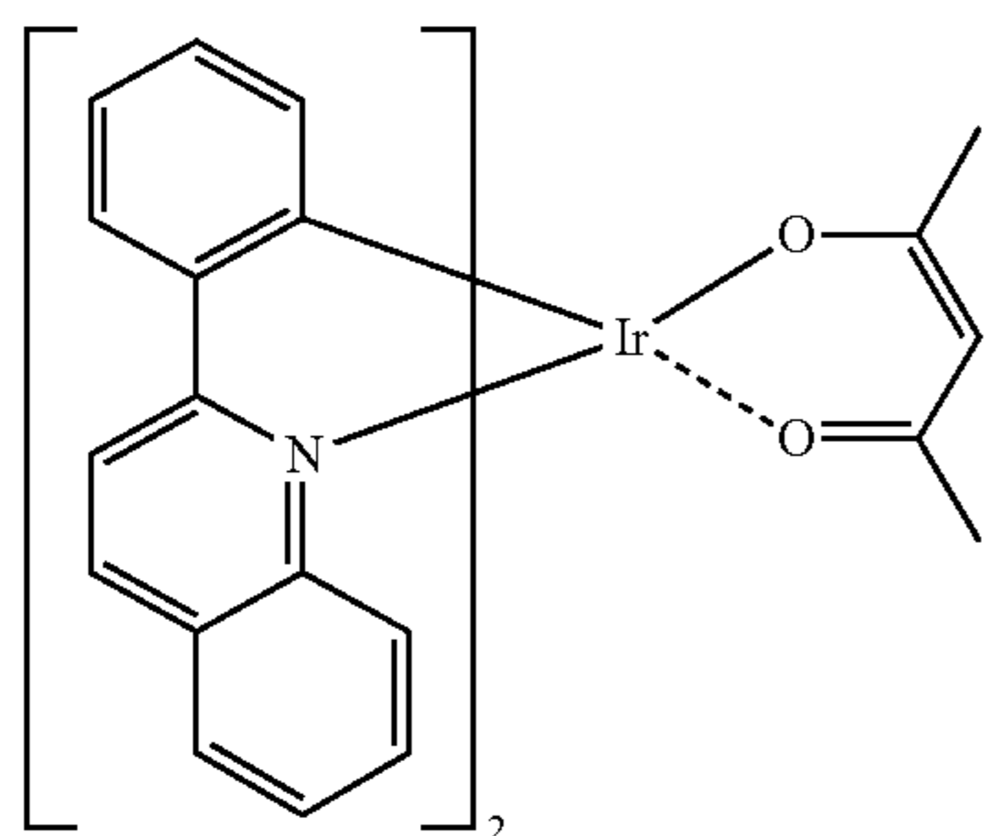
Ir(pq) 2 (acac)
