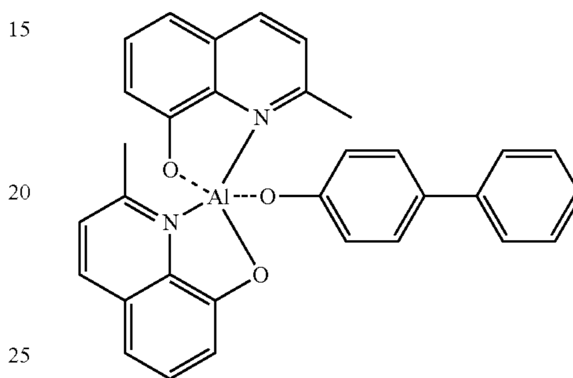
BALq
