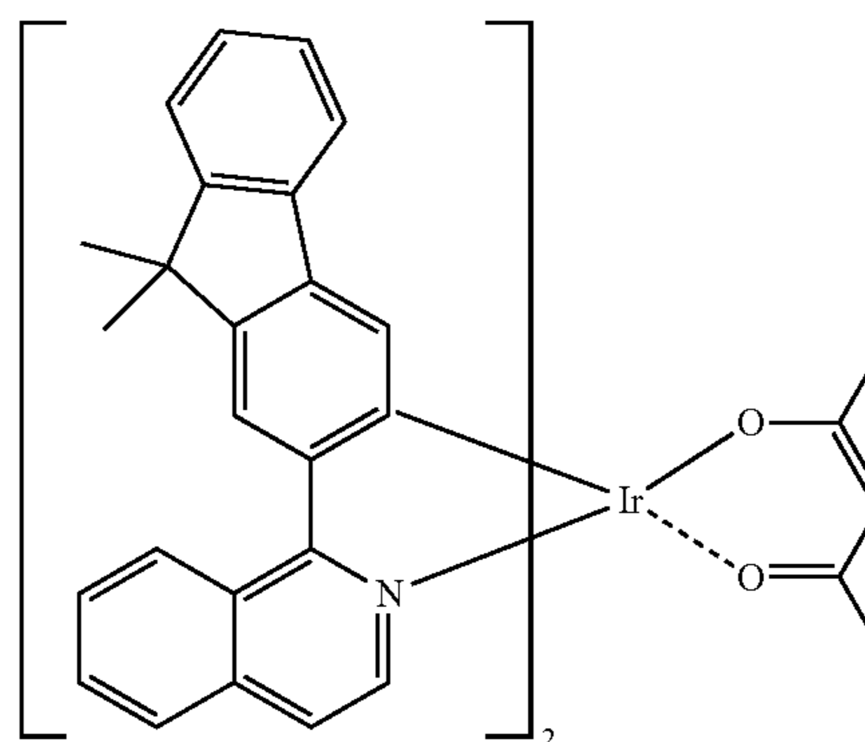
Ir(flq) 2 (acac)
