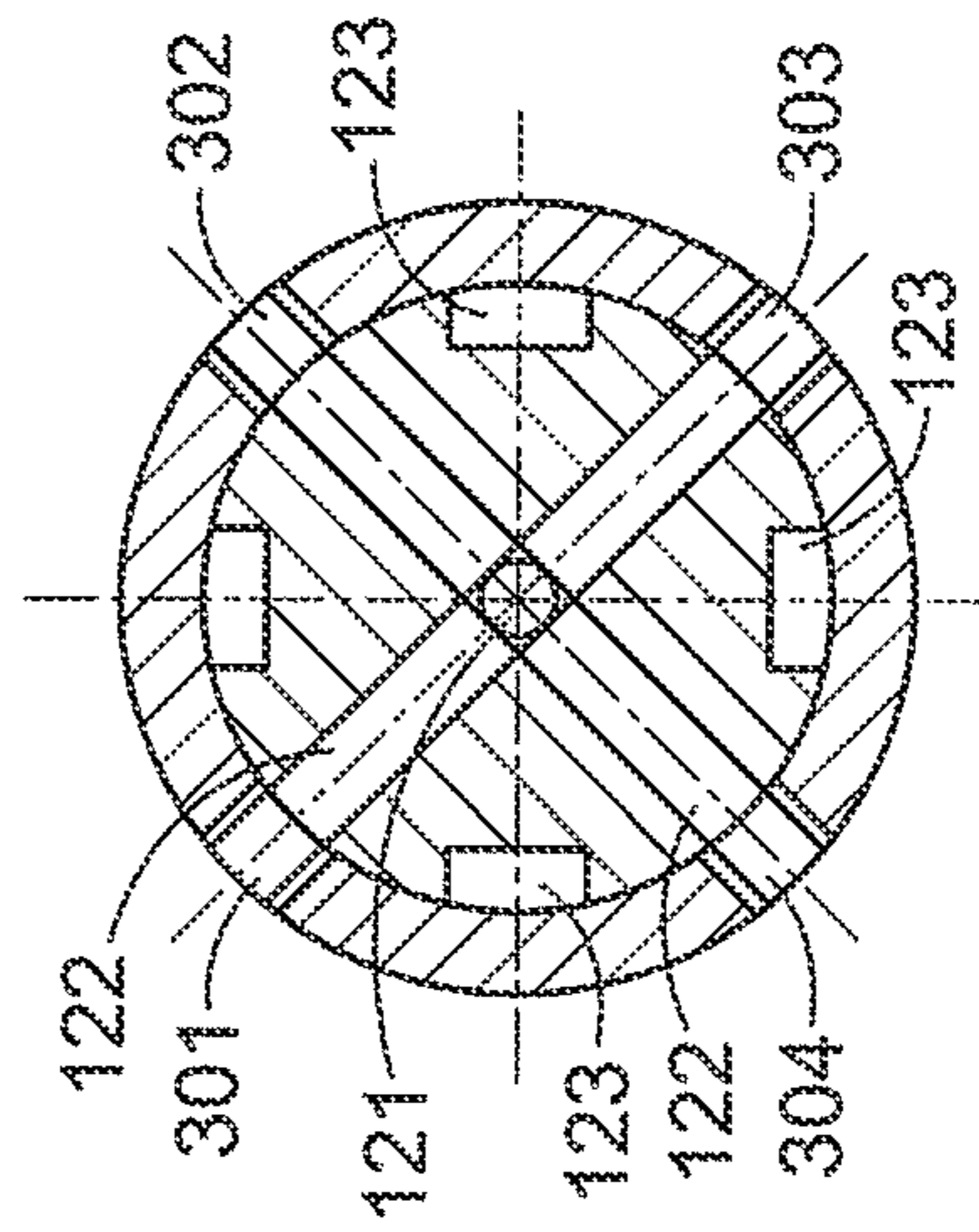
FIG. 3A
