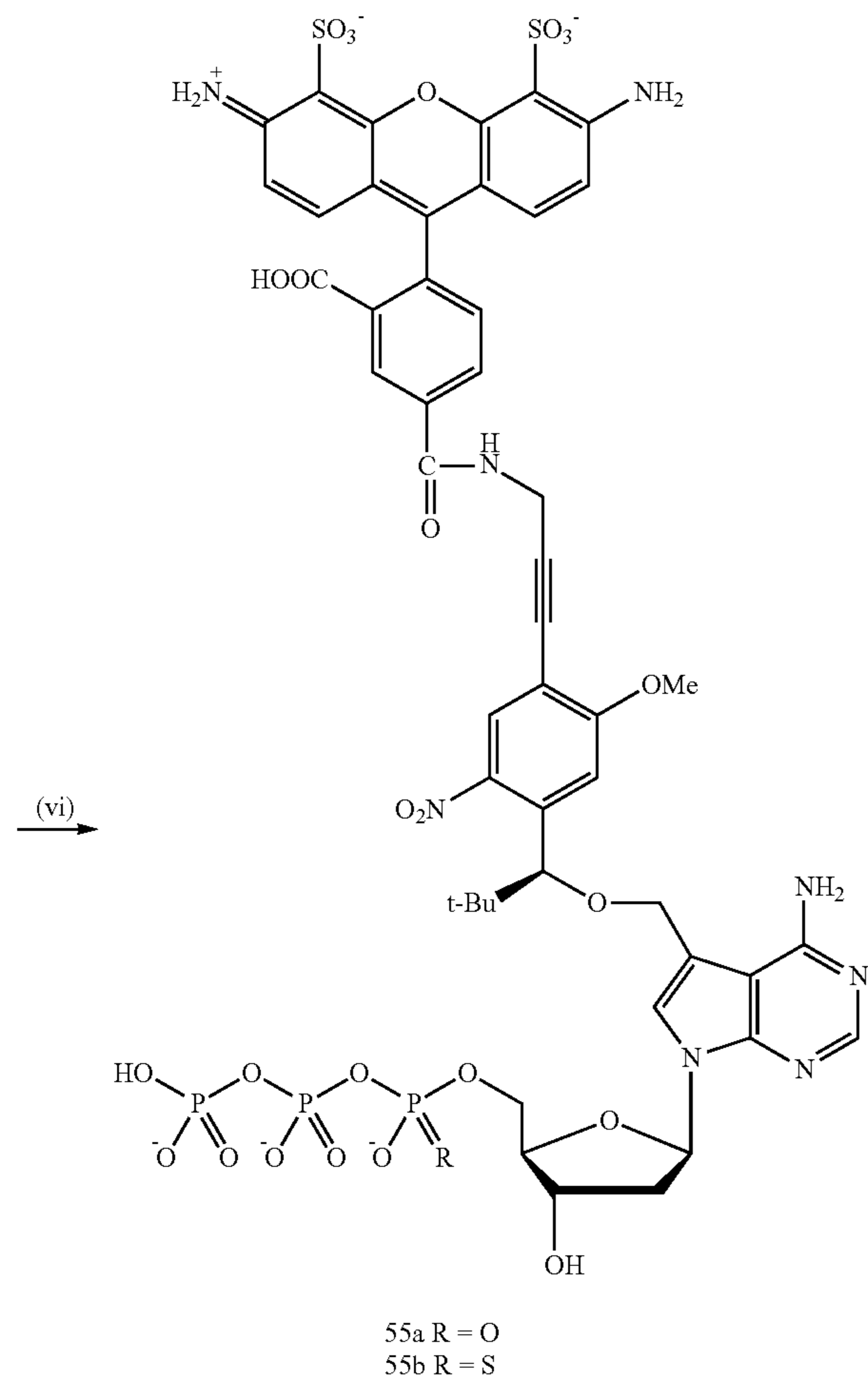
Scheme S25b.
