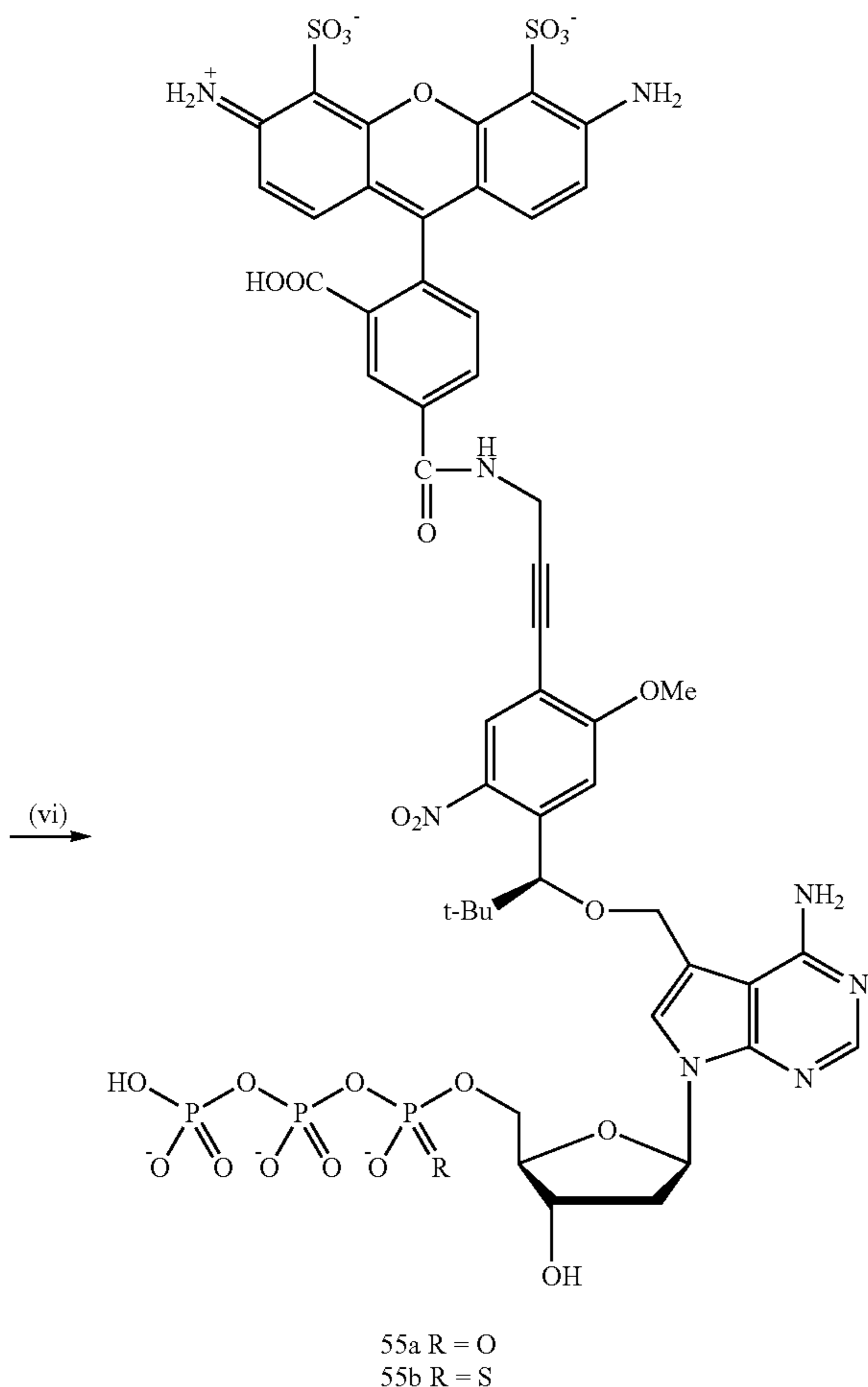
Scheme S25b.
