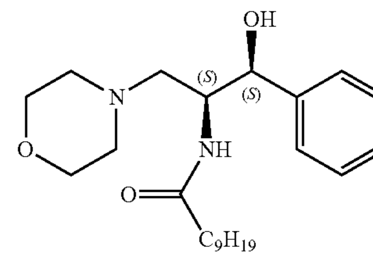
L-threo-PDMP
