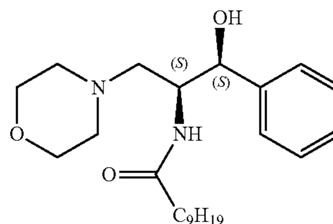
L-threo-PDMP
