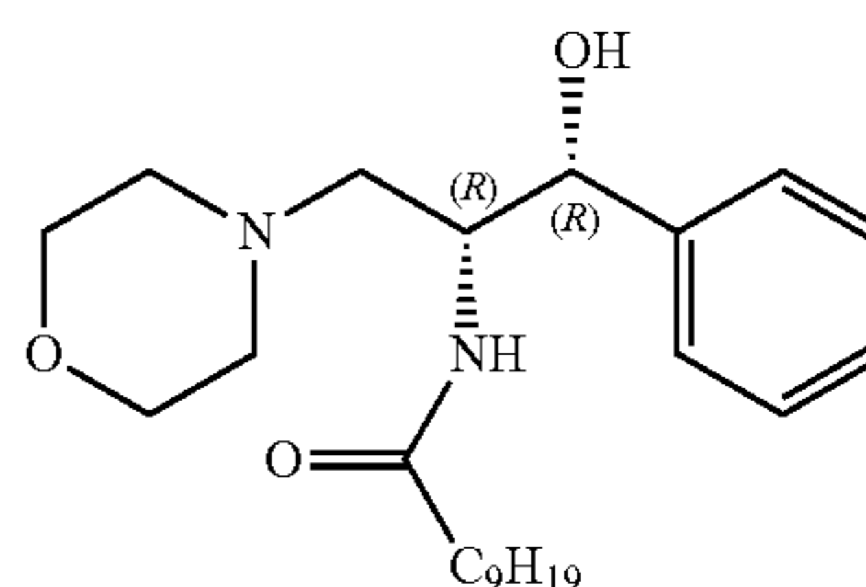
L-threo-PDMP
