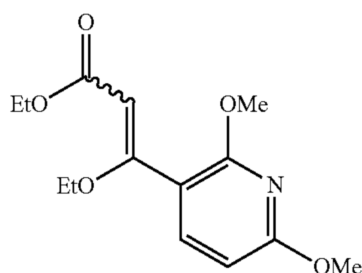
(Z,E)-Ethyl 3-(2,6-dimethoxypyridin-3-yl)-3-ethoxyacrylate
