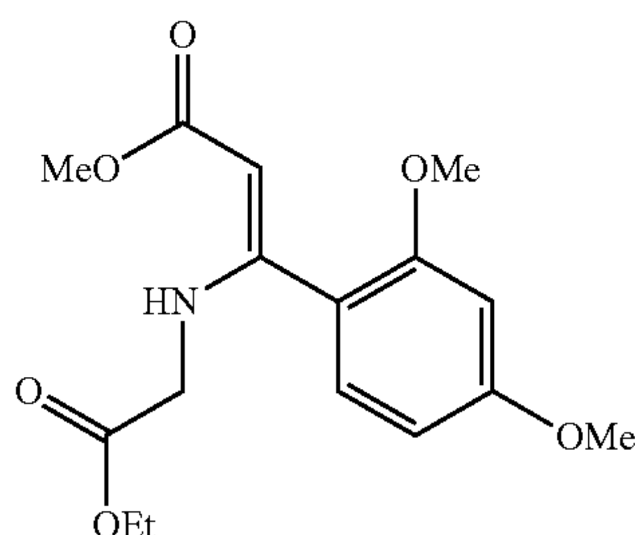
(Z)-Methyl 3-(2,4-dimethoxyphenyl)-3-((2-ethoxy-2-oxoethyl)amino)acrylate
