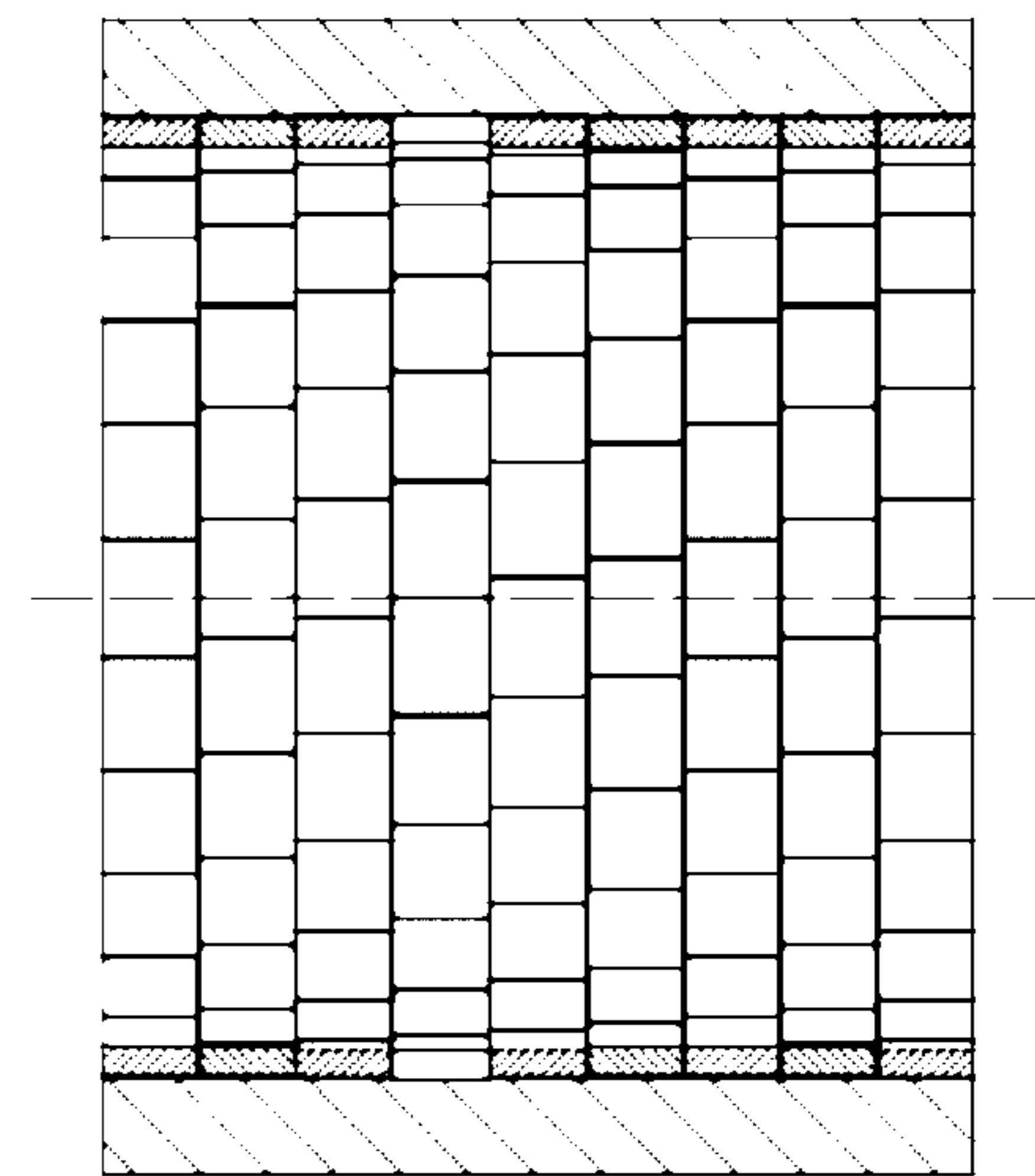
Section A-A
