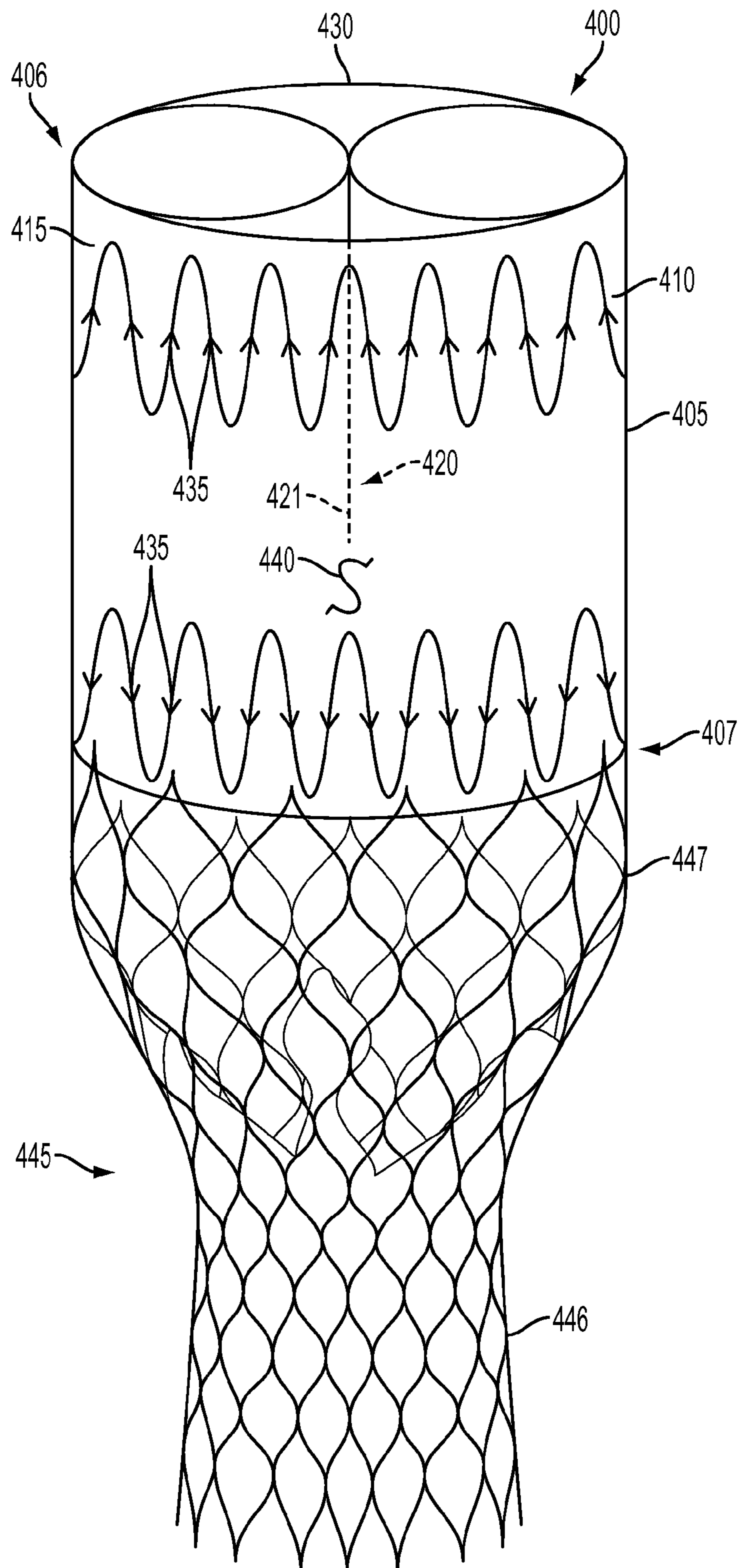
FIG. 5B
