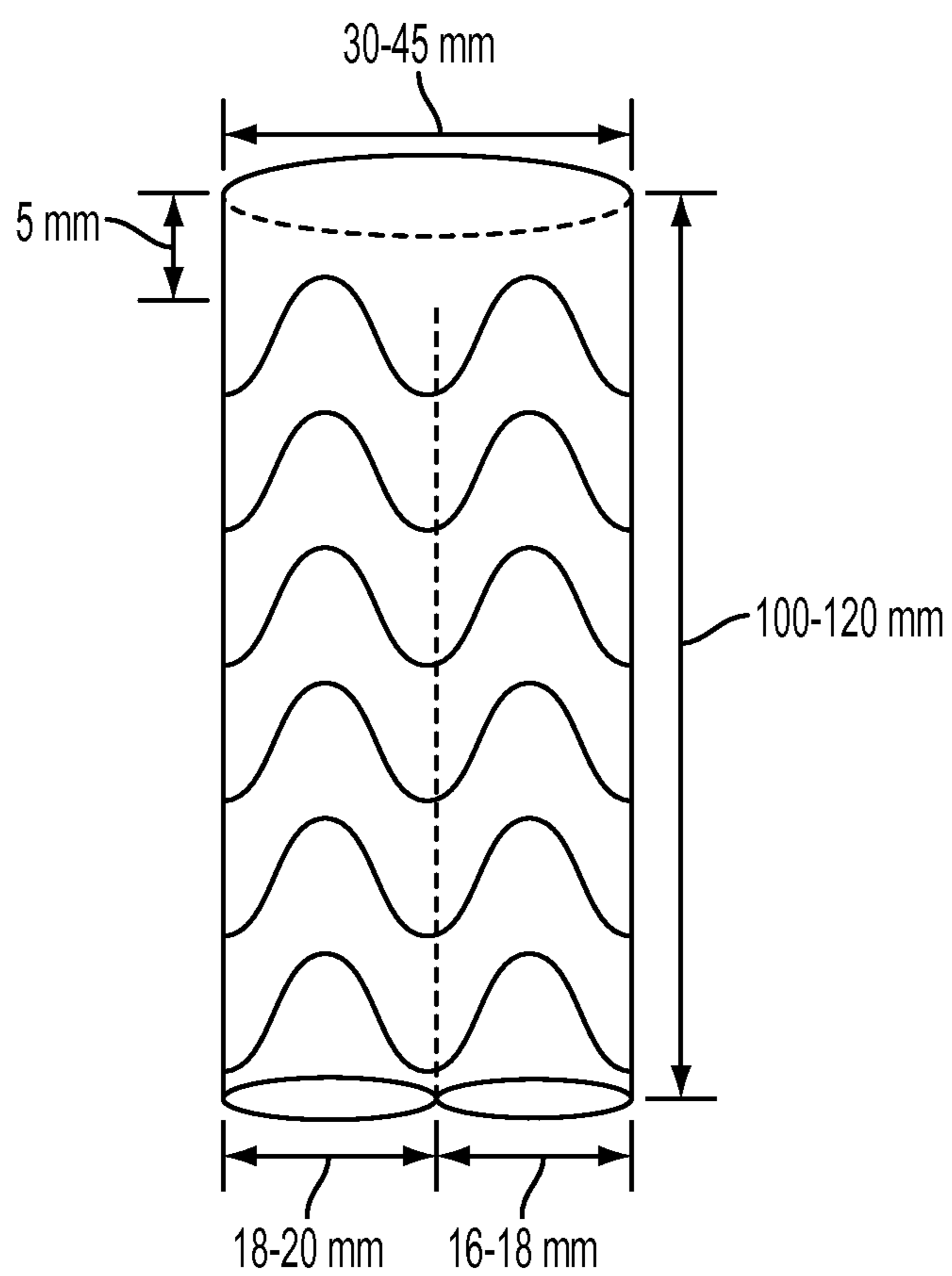
FIG. 2A
