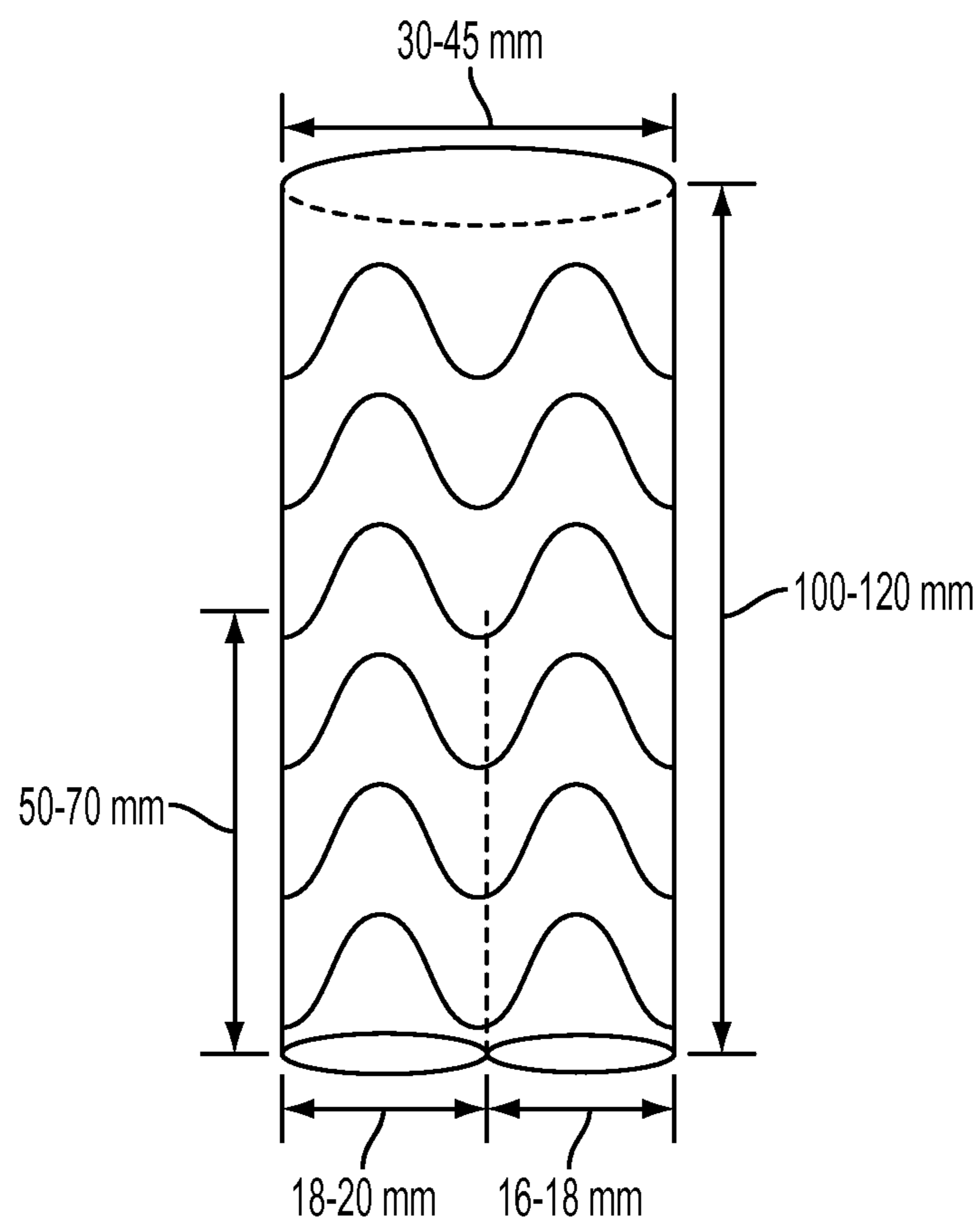
FIG. 1A
