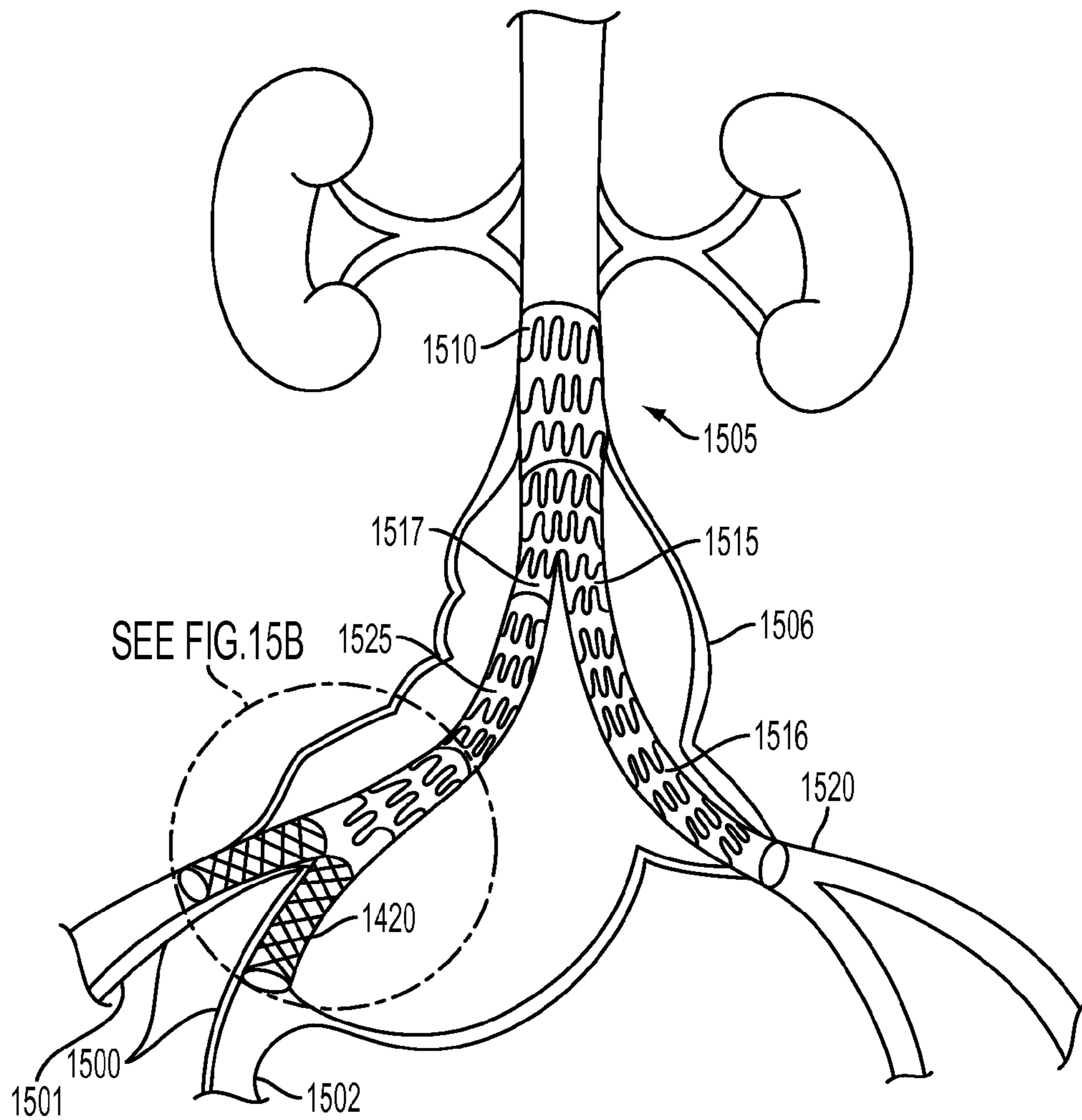
FIG. 15A
