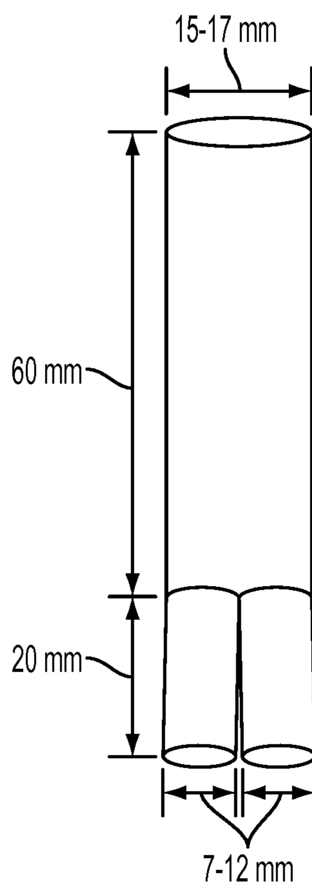
FIG. 13A
