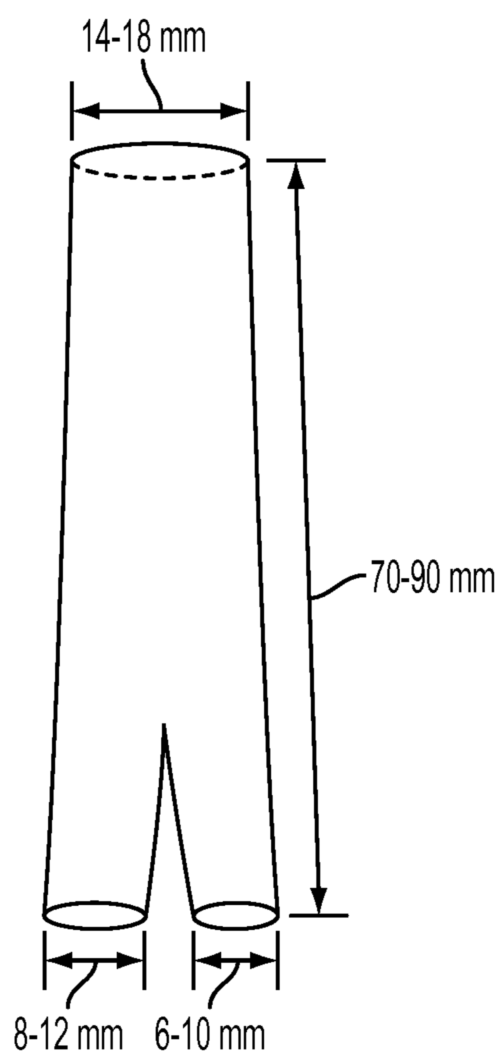
FIG. 14A
