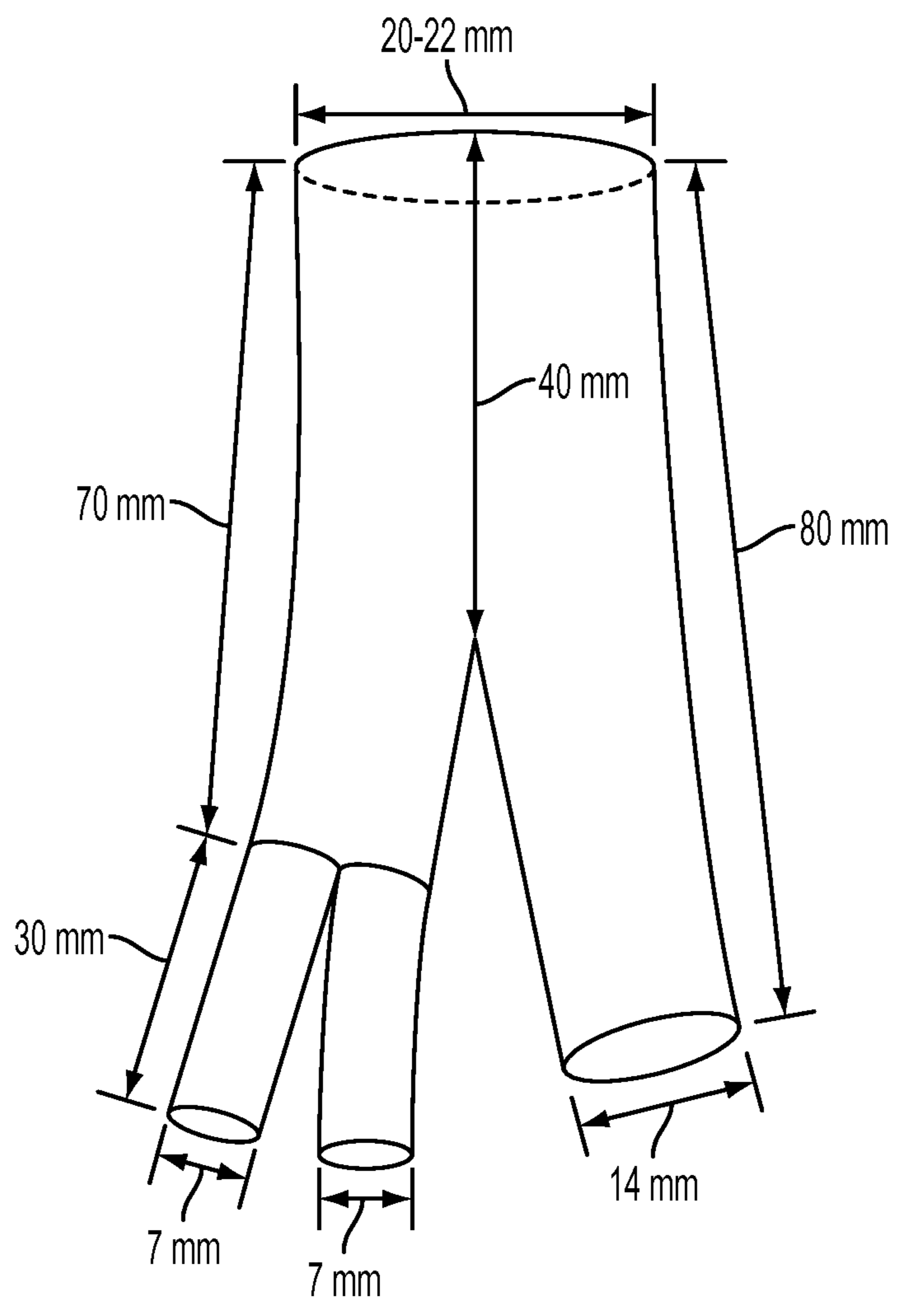
FIG. 9A
