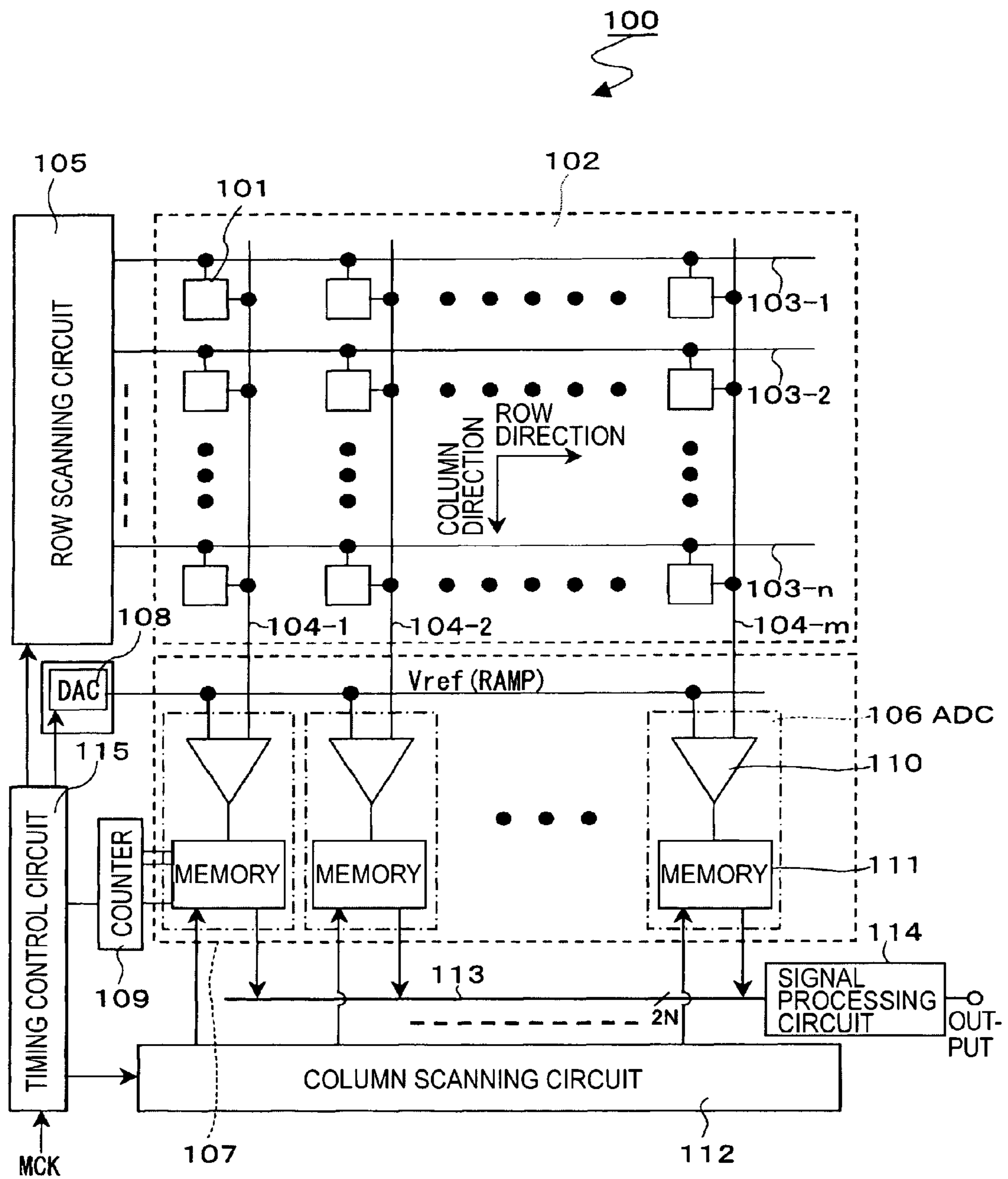
FIG. 15
