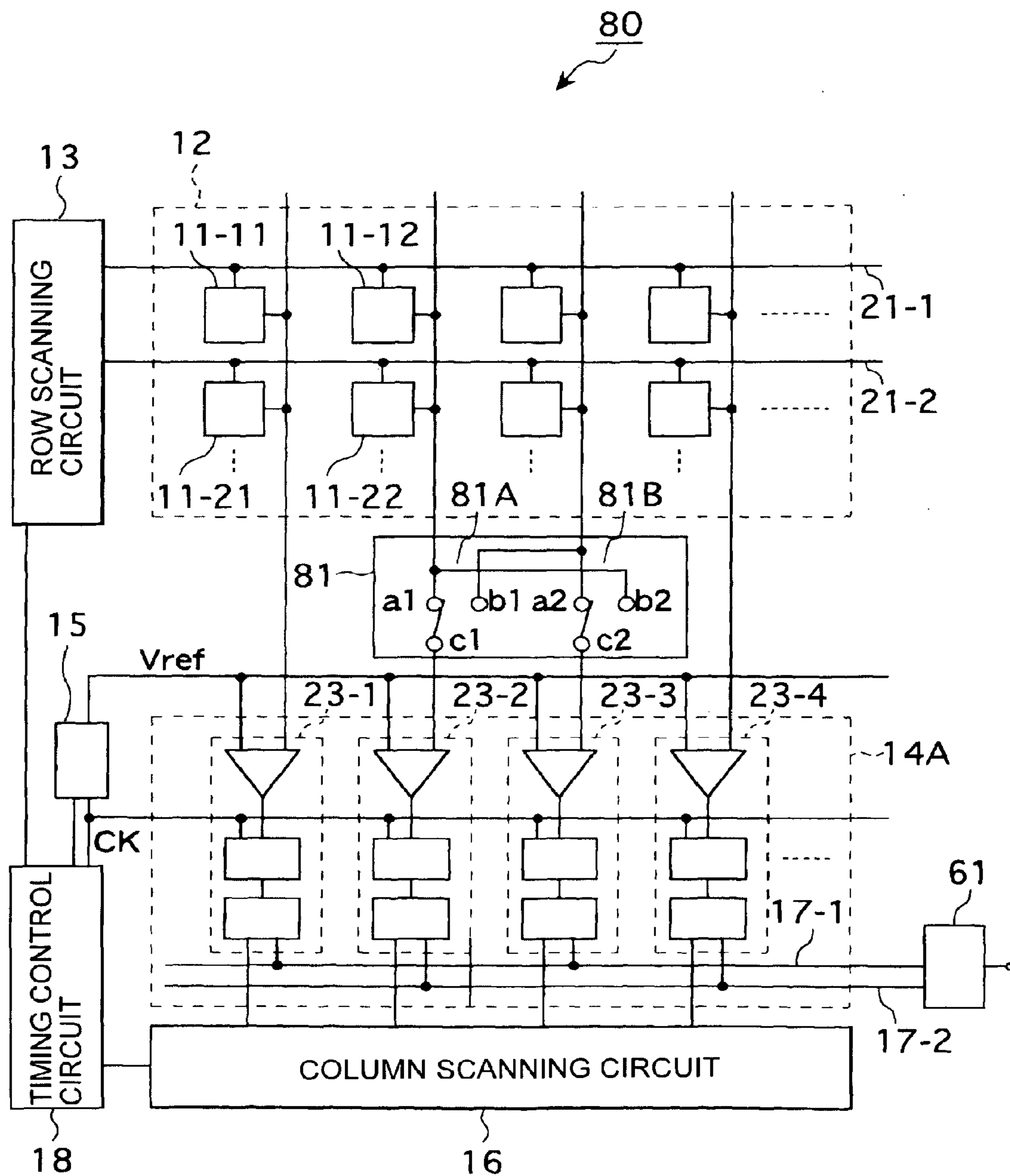
FIG. 14
