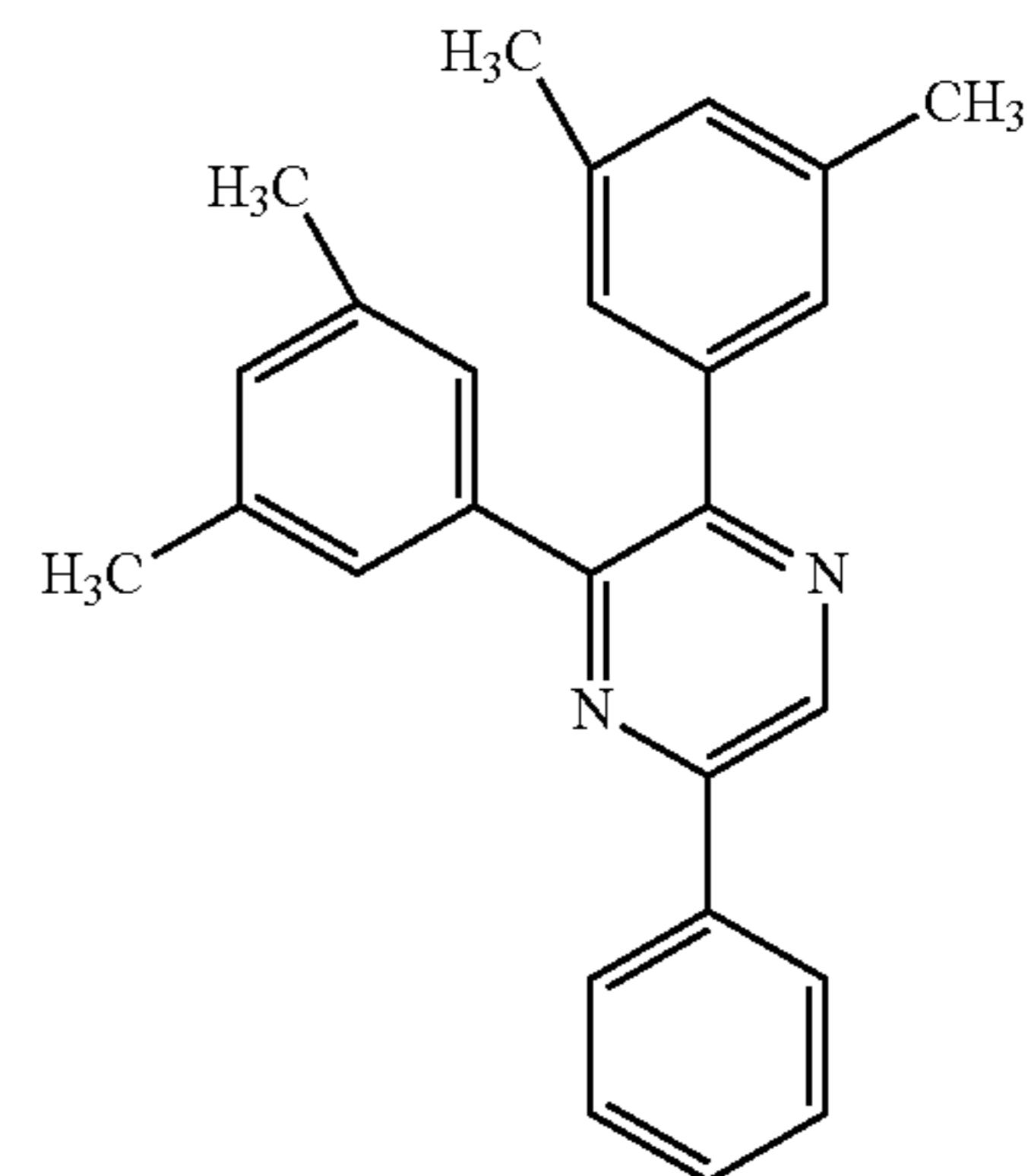
Hdmdppr-P
