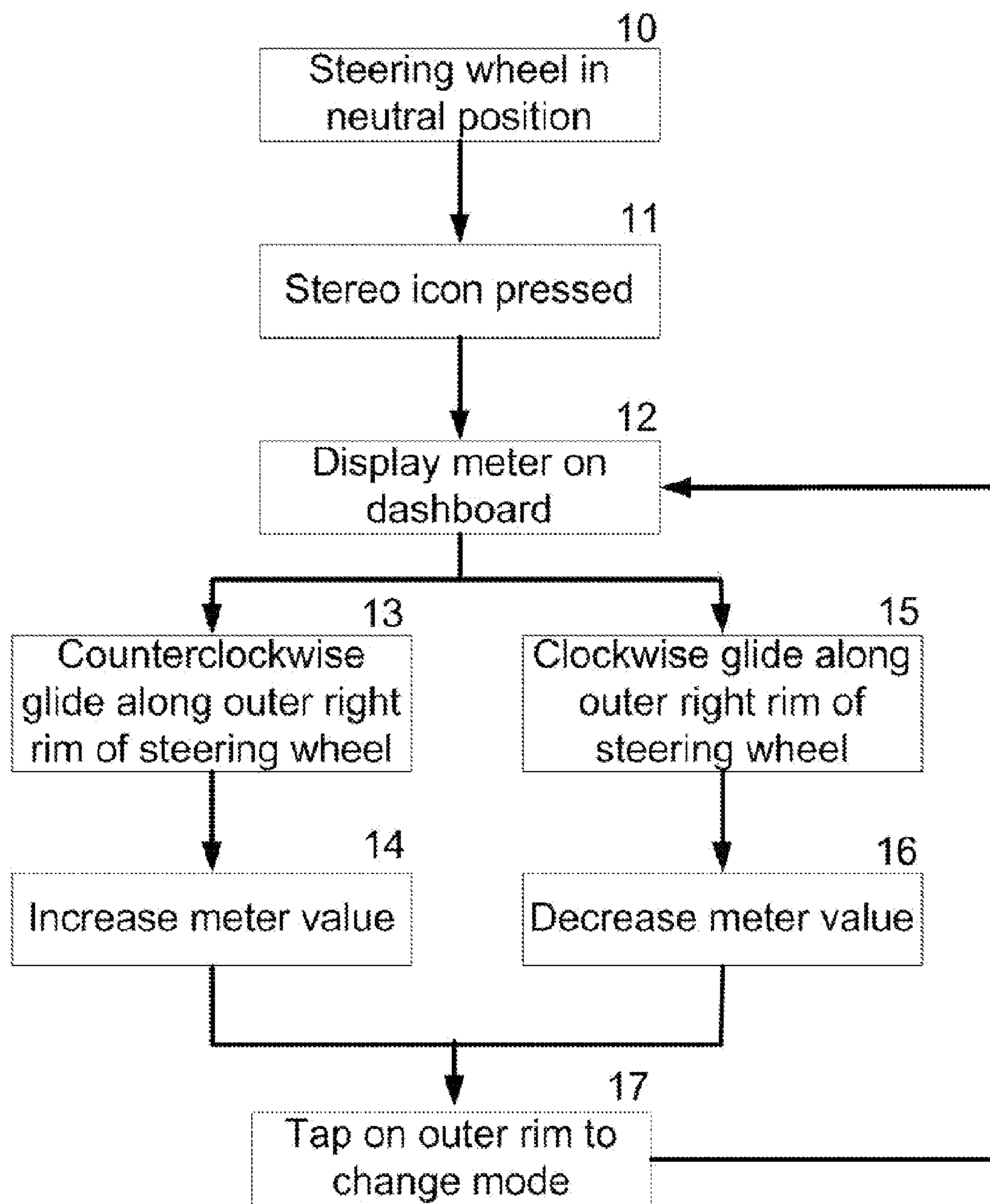
FIG. 6
