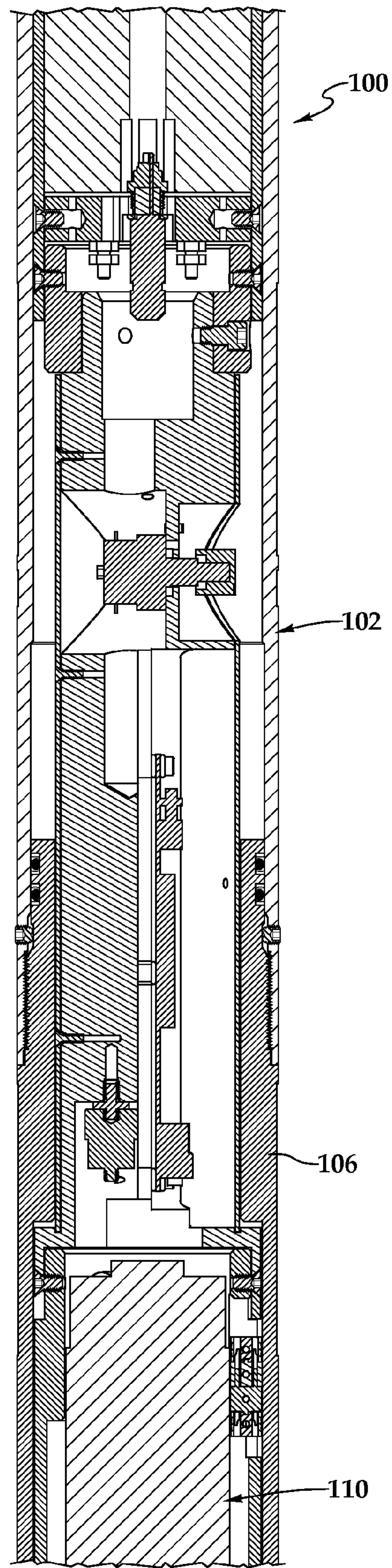
Fig.2B
