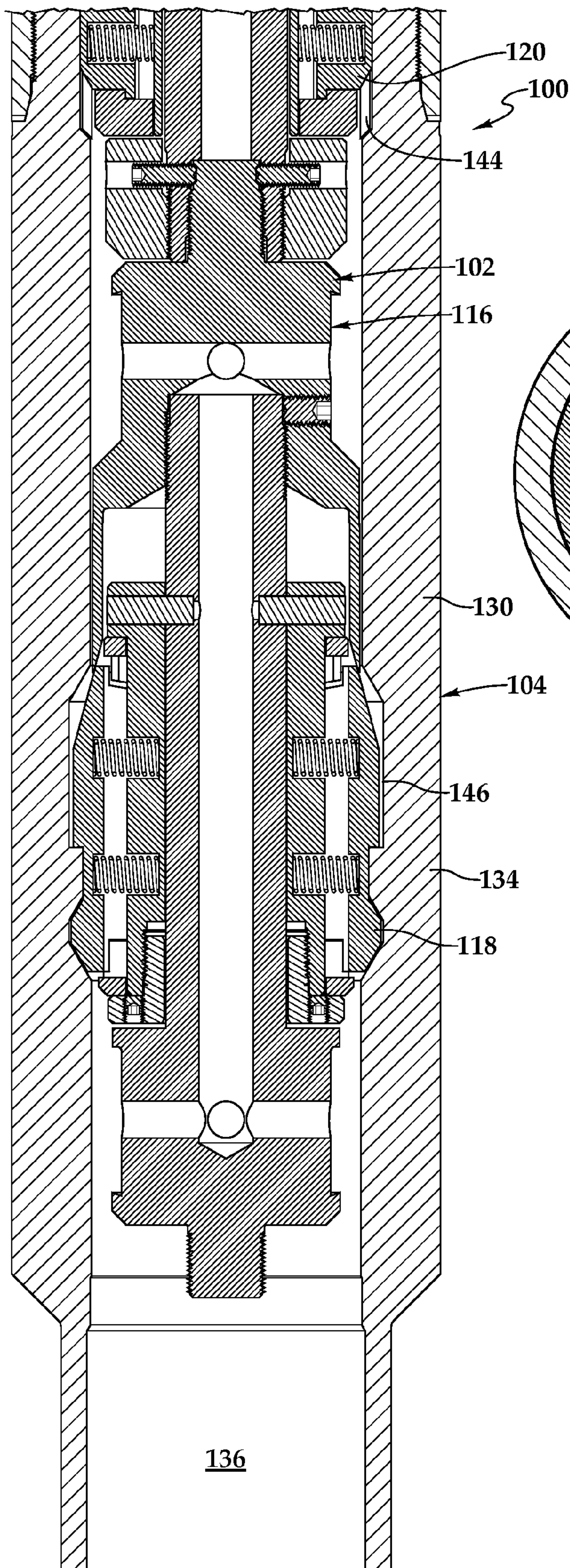
Fig.2E
