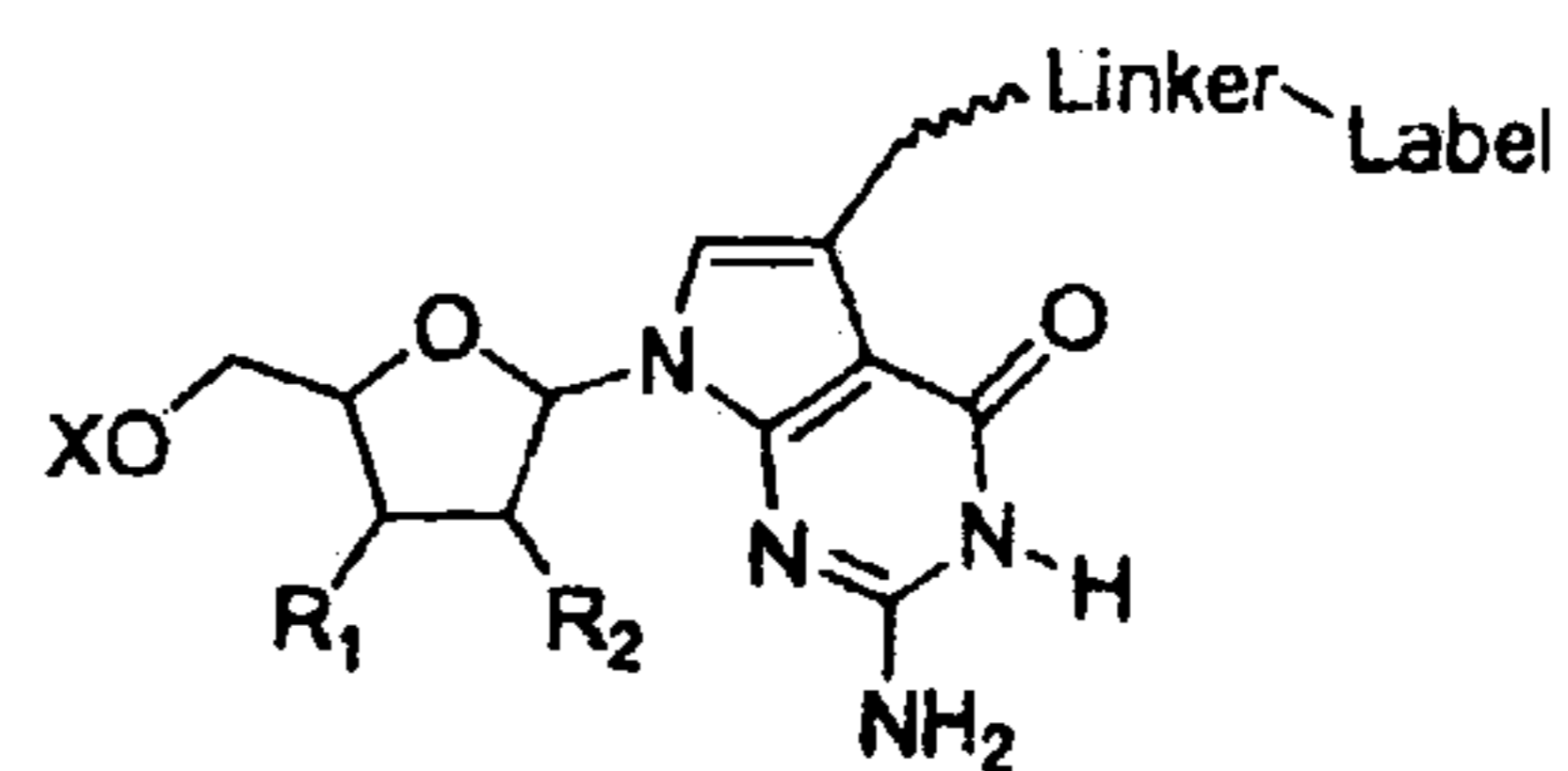
N7 Dezaguanosine C7-linker
