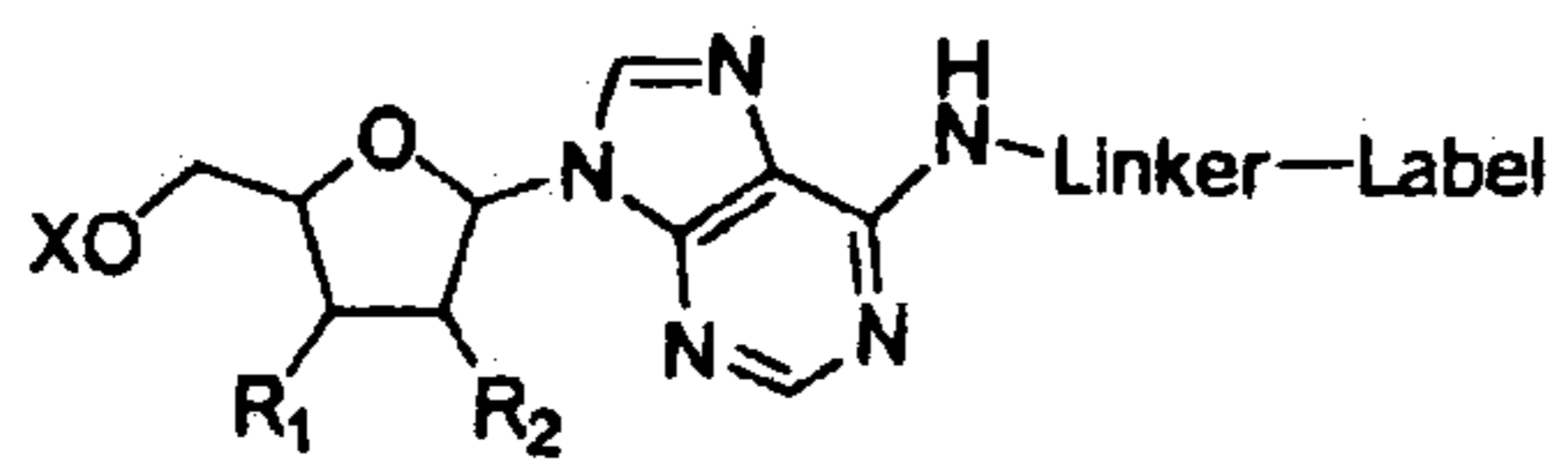
Adenosine N6-linker
