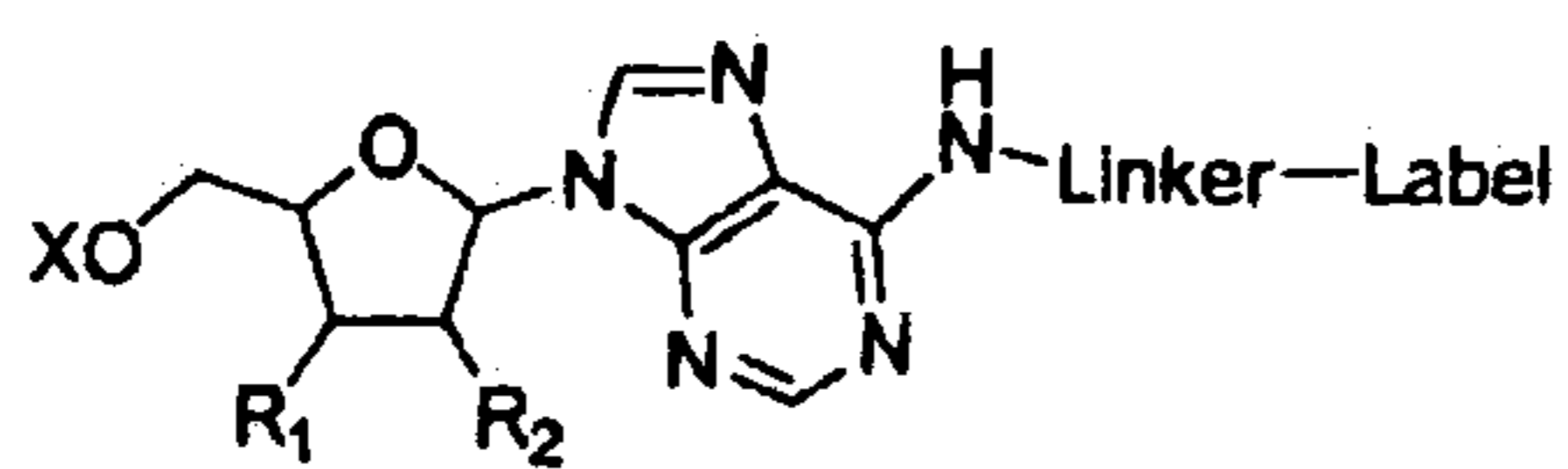
Adenosine N6-linker
