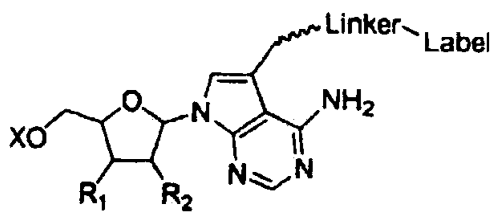
N7 Dezaadenosine C7-linker
