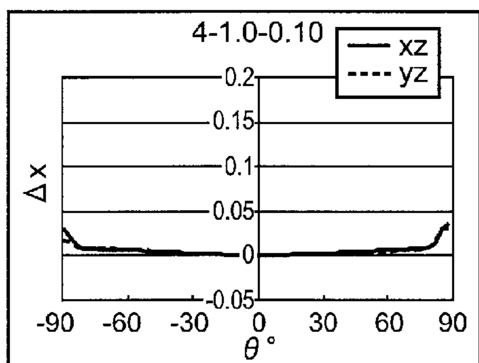
Fig. 13A \Delta_n
