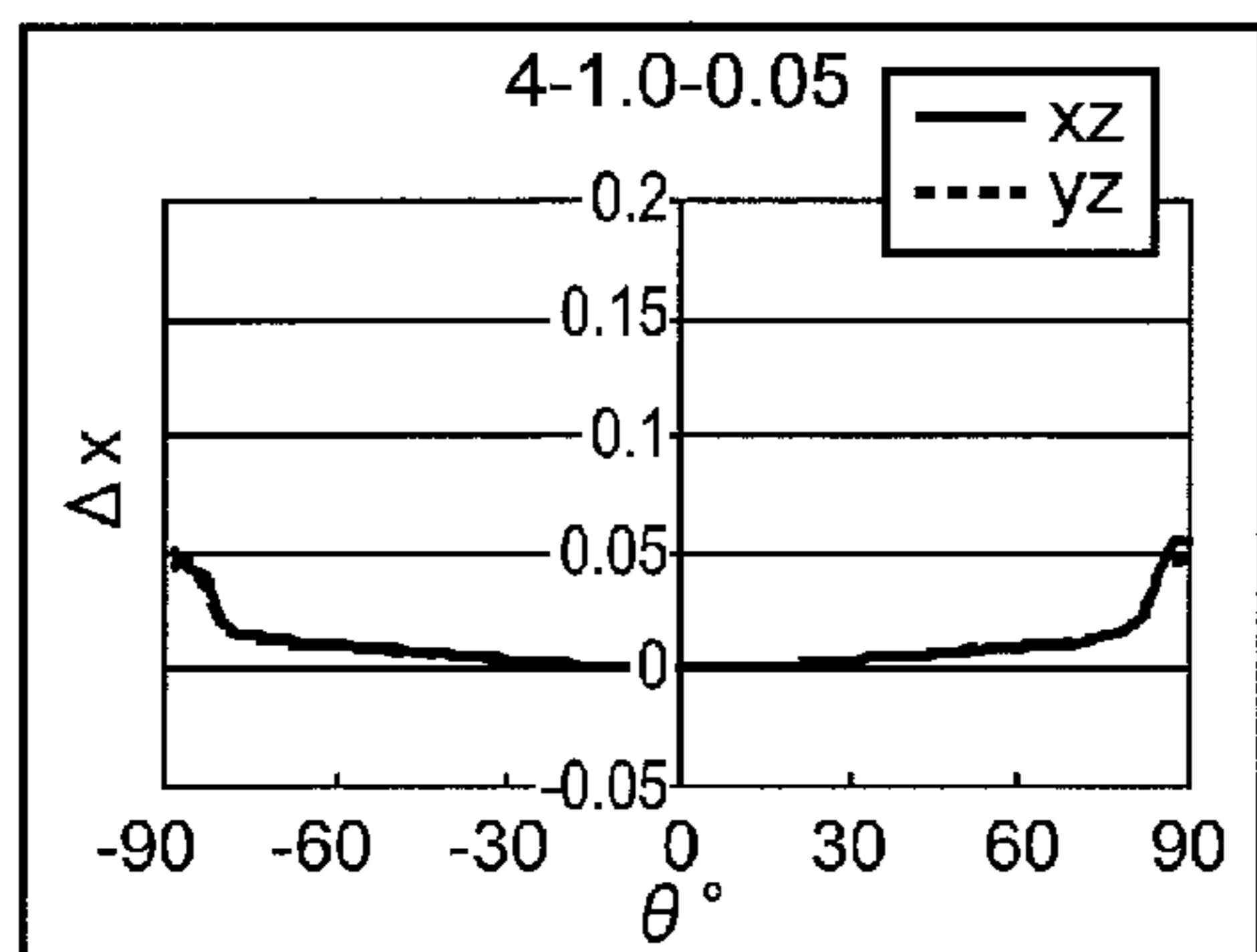
Fig. 12A \Delta_x
