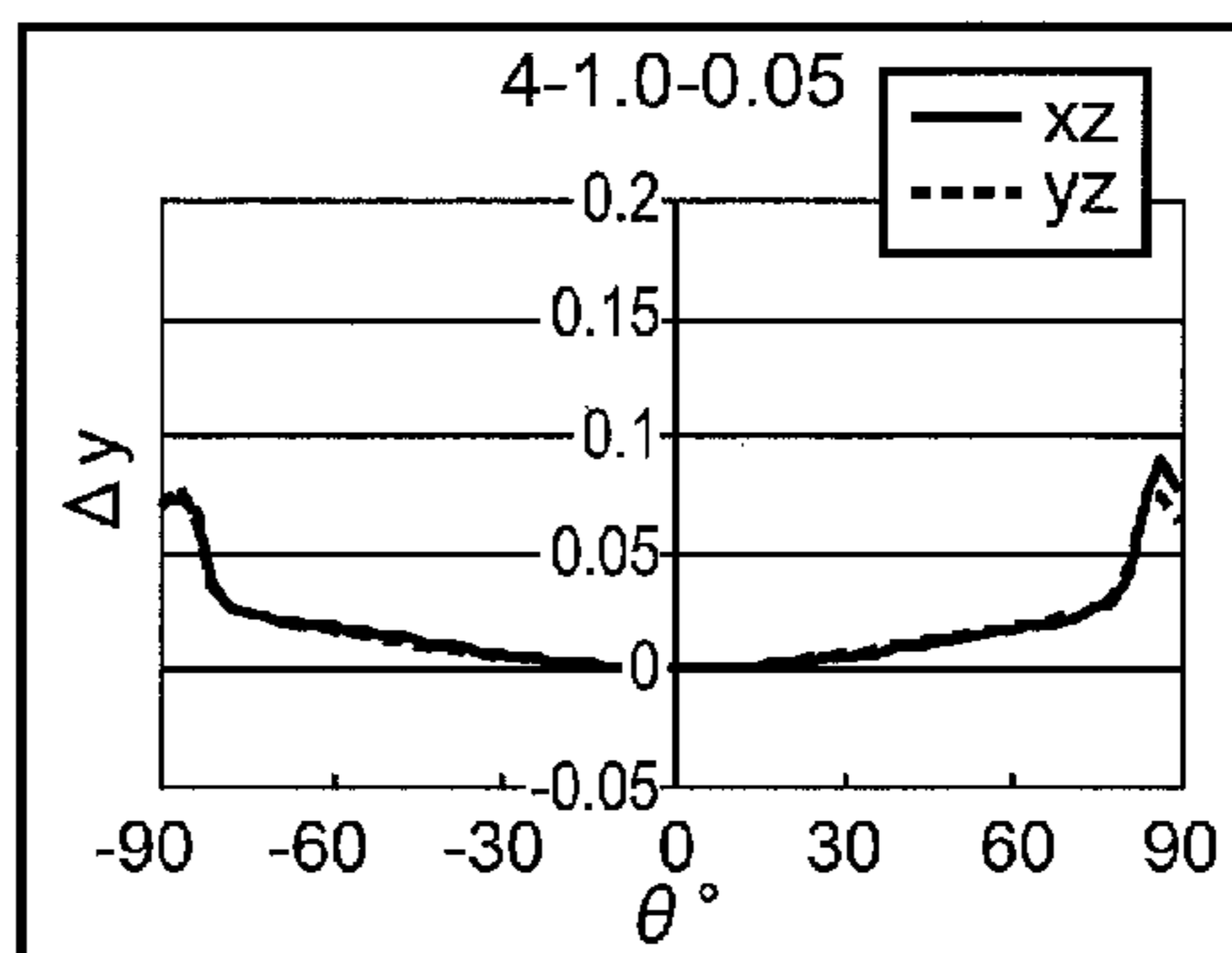
Fig. 12B \Delta_y
