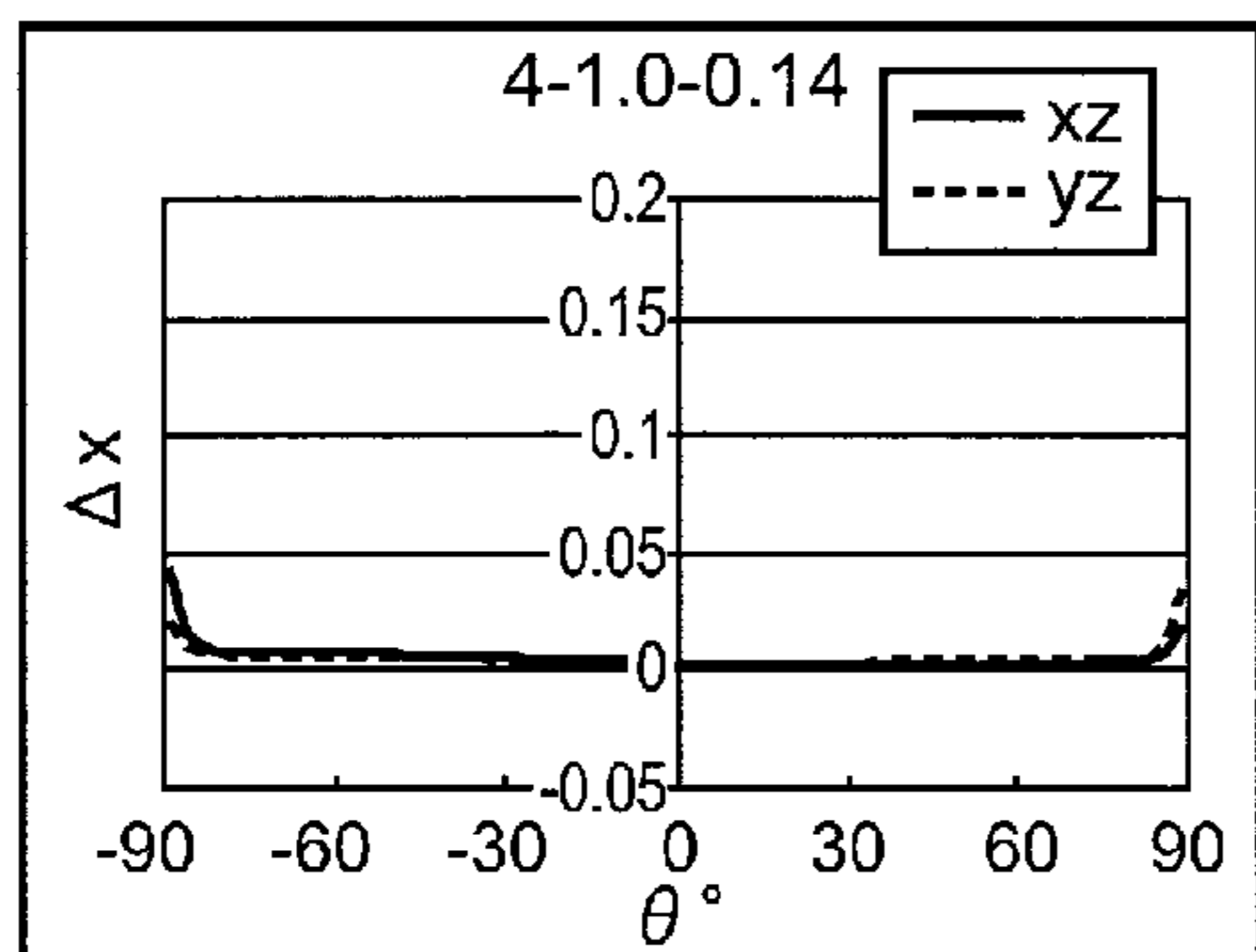
Fig. 14A \Delta_x
