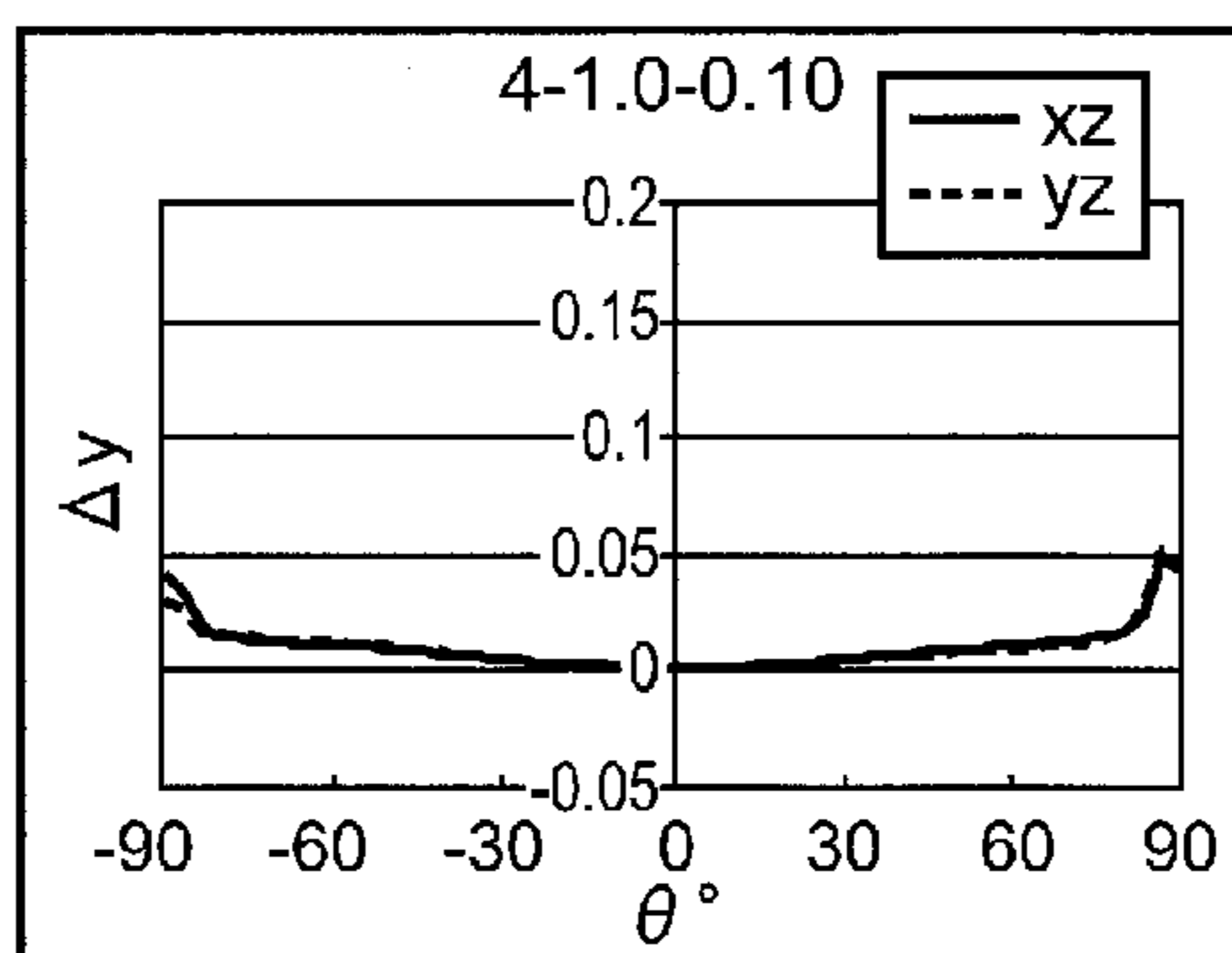
Fig. 13B \Delta_y
