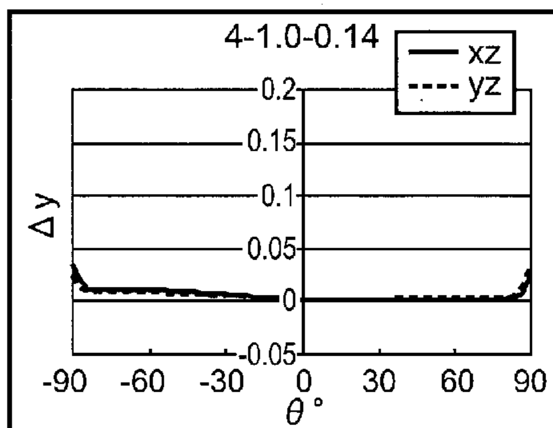
Fig. 14B \Delta_y
