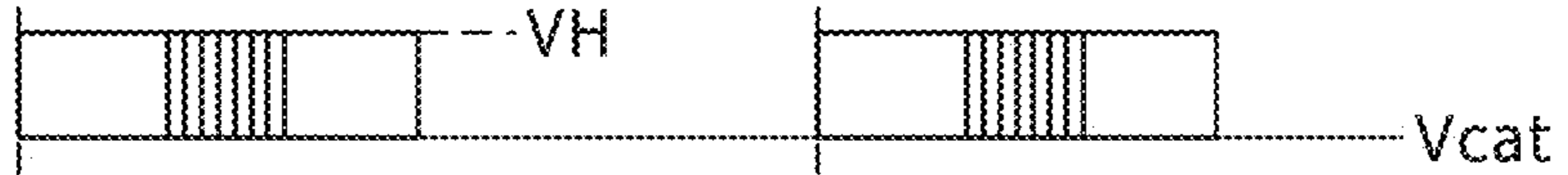
FIG. 32C DUTY40%
