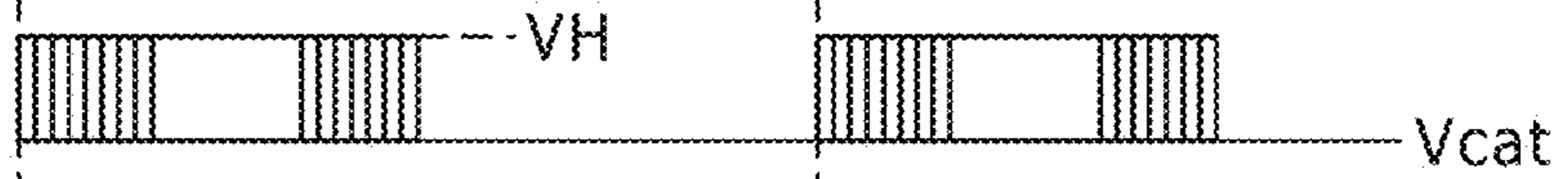
FIG. 32B DUTY40%
