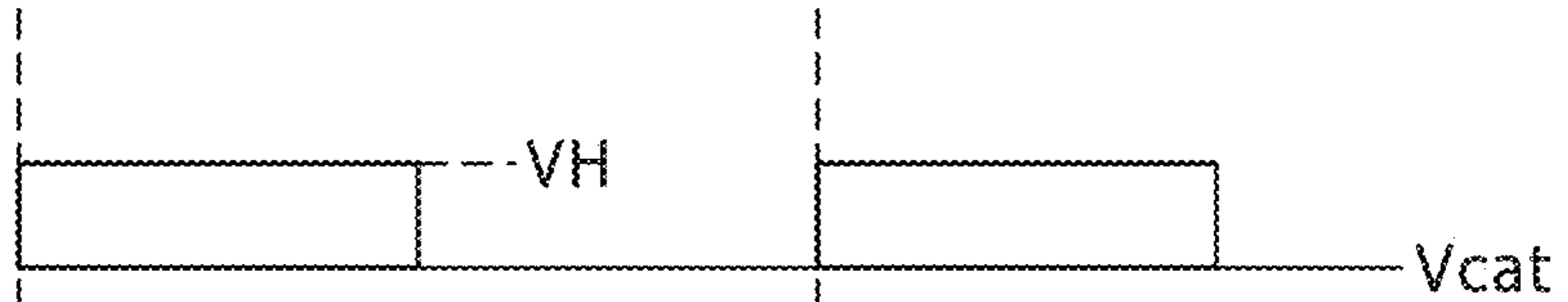
FIG. 32A DUTY50%
