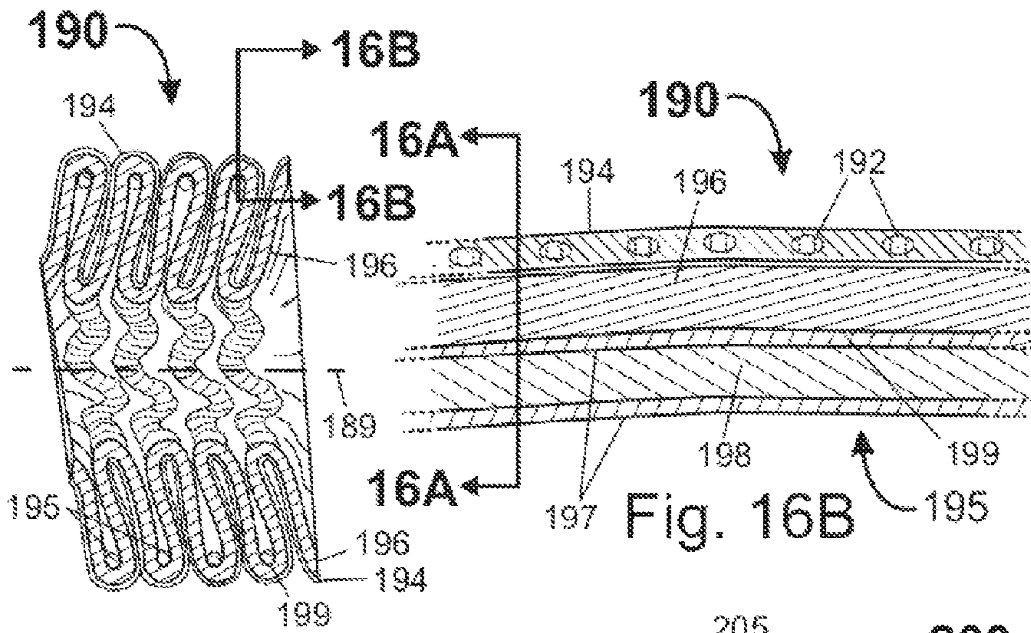
Fig. 16A
