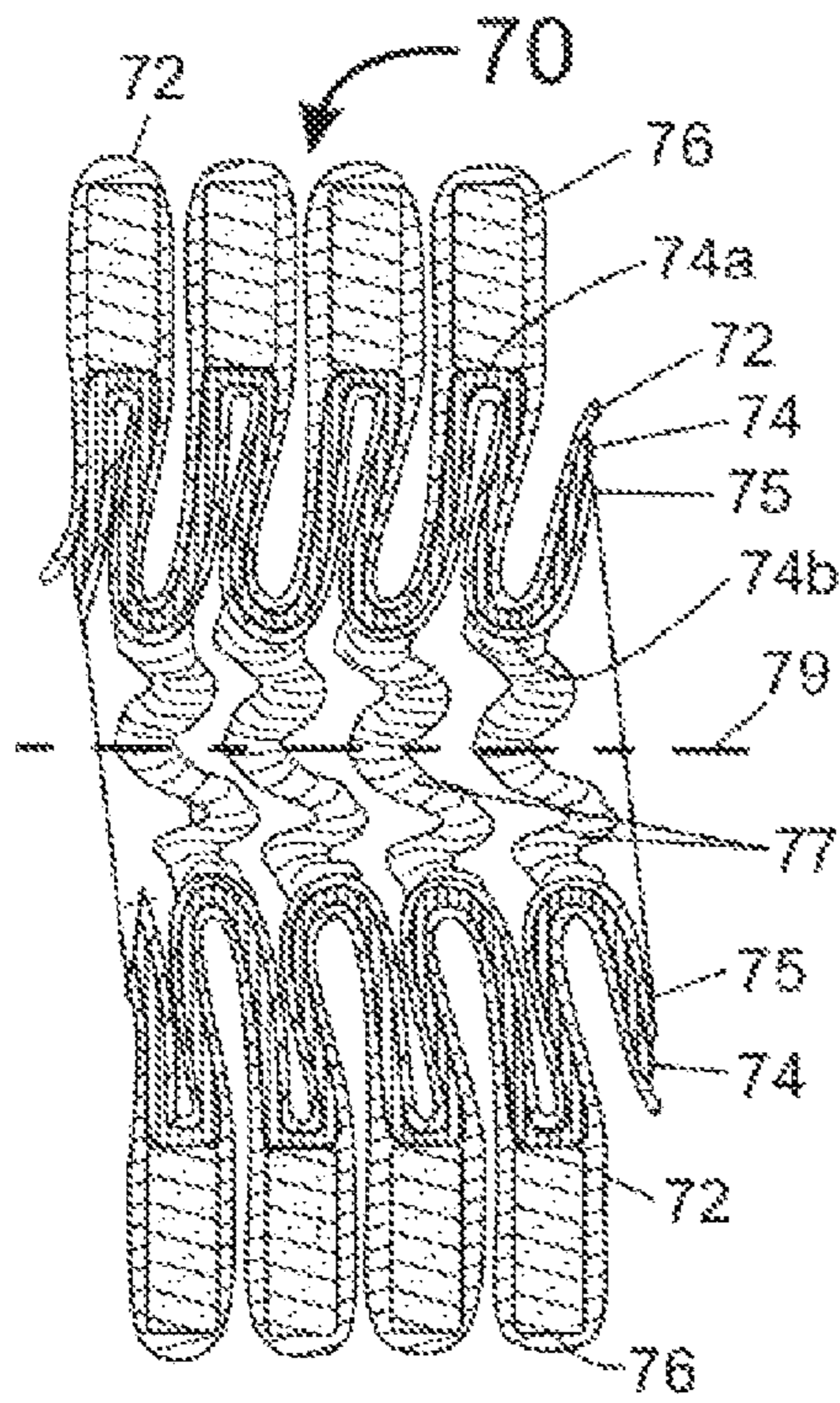
Fig. 4A
