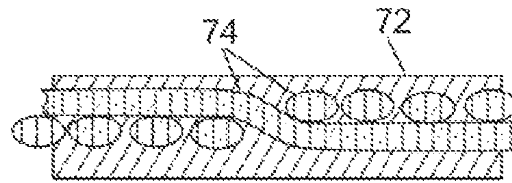
Fig. 4C
