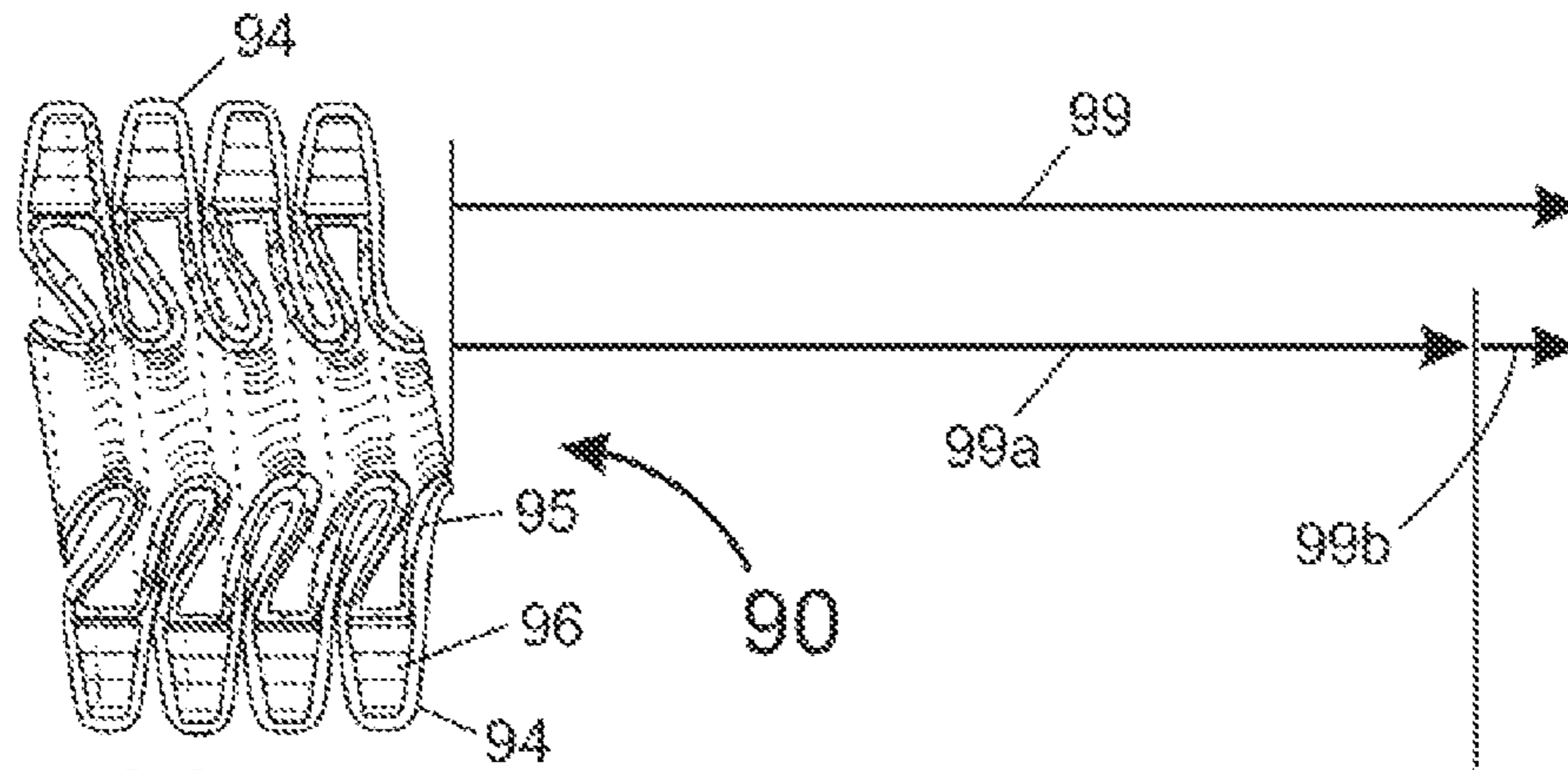
Fig. 6A
