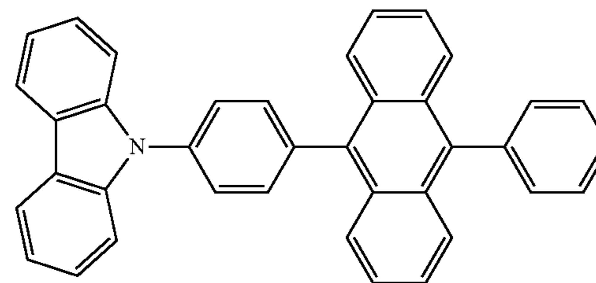
CzPA
