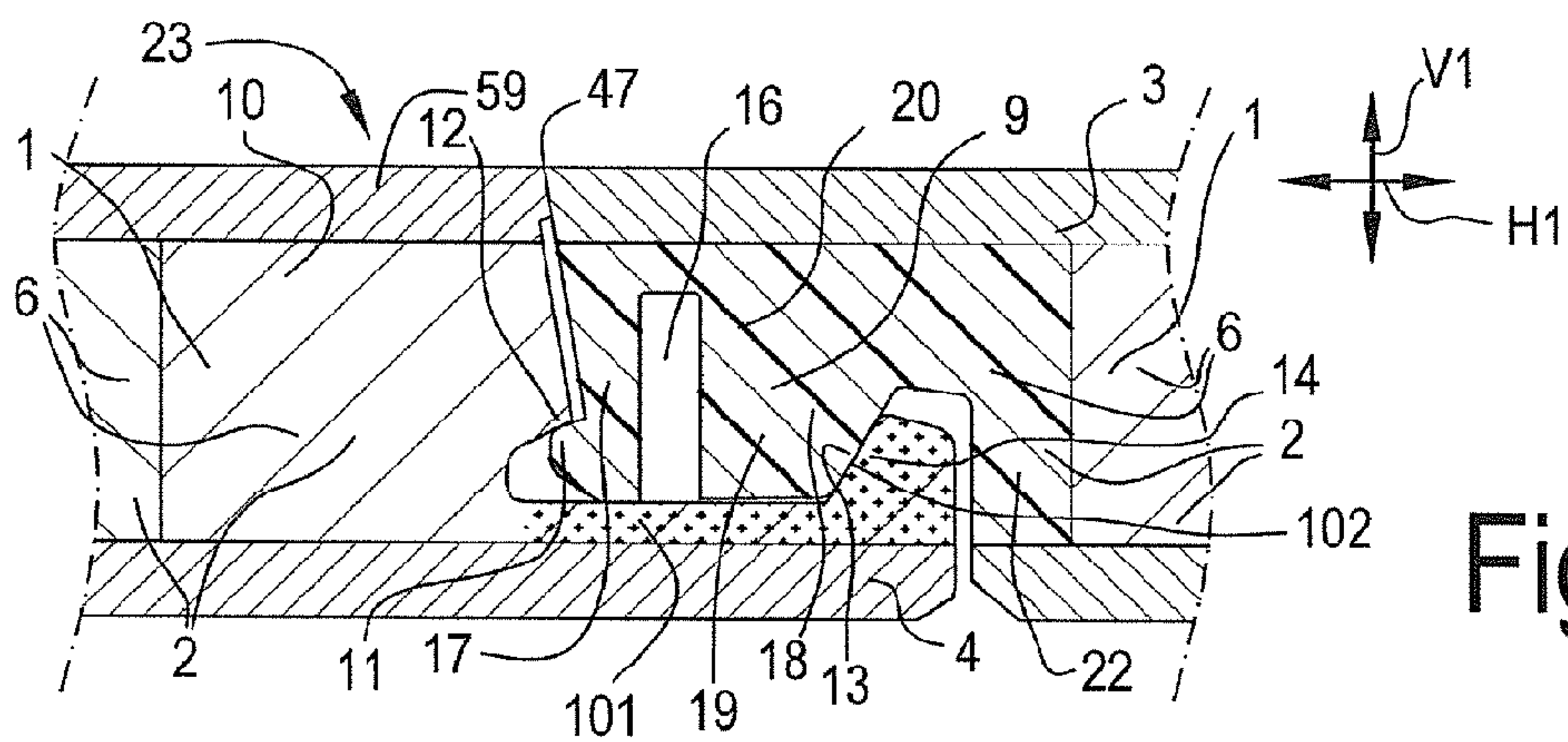
Fig. 31
