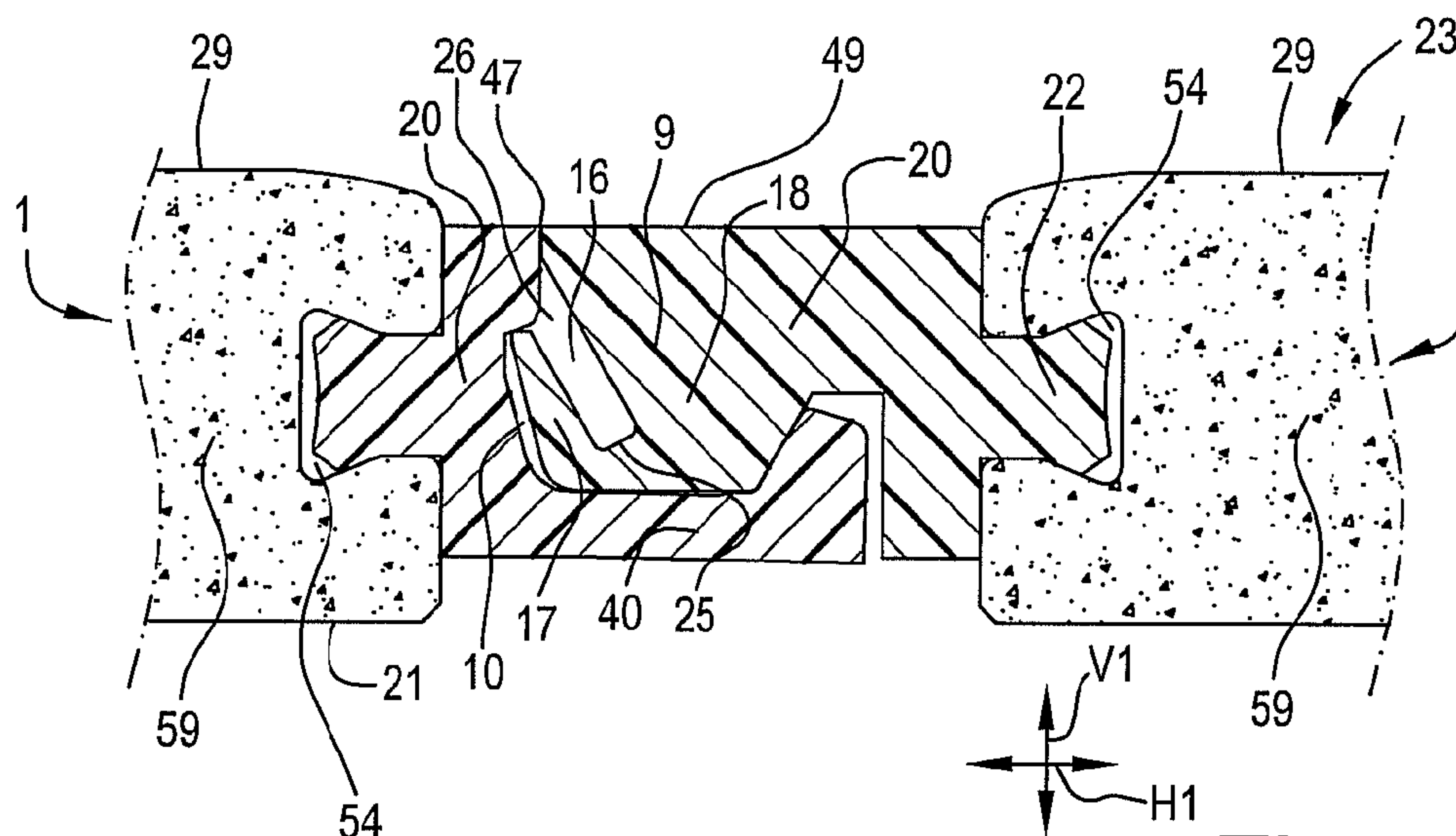
Fig. 15
