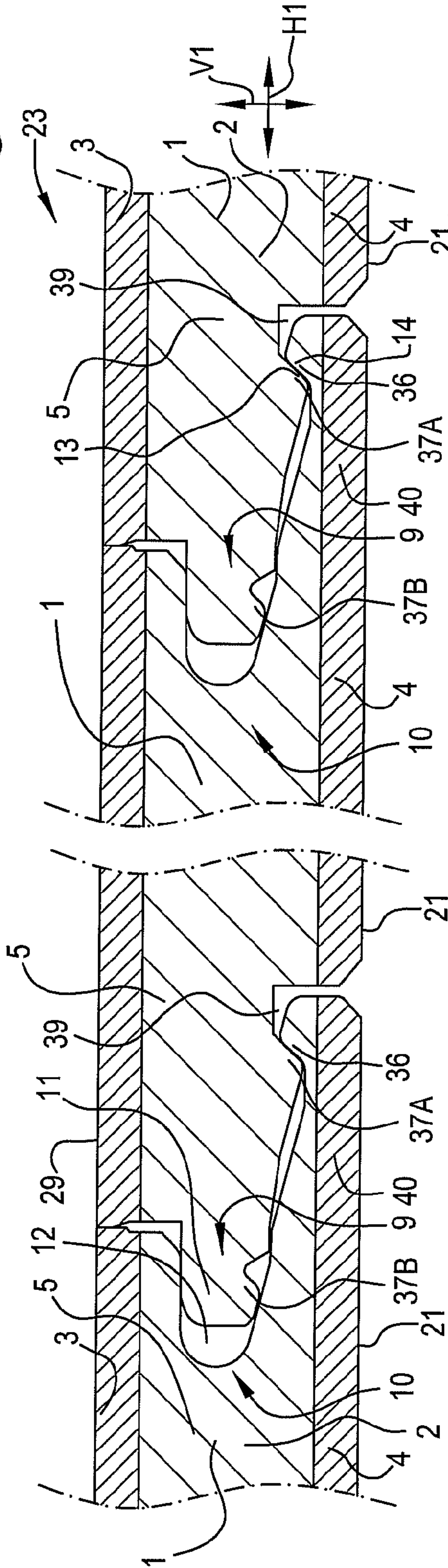
Fig. 17
